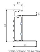
Telaio sezione trasversale
