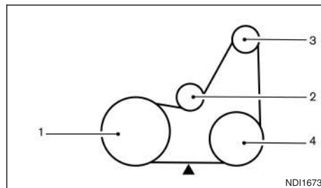
Motore K9K
