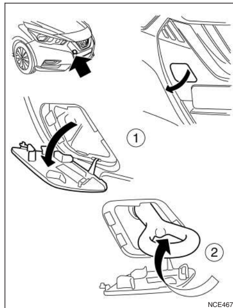
Installazione del gancio di recupero
