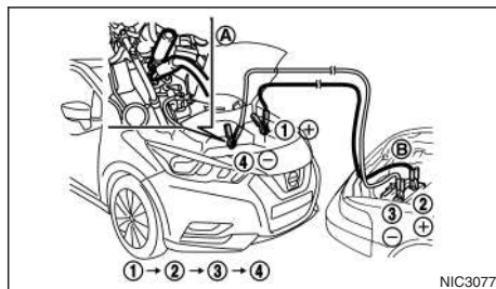
Modelli con motore HR09DET
