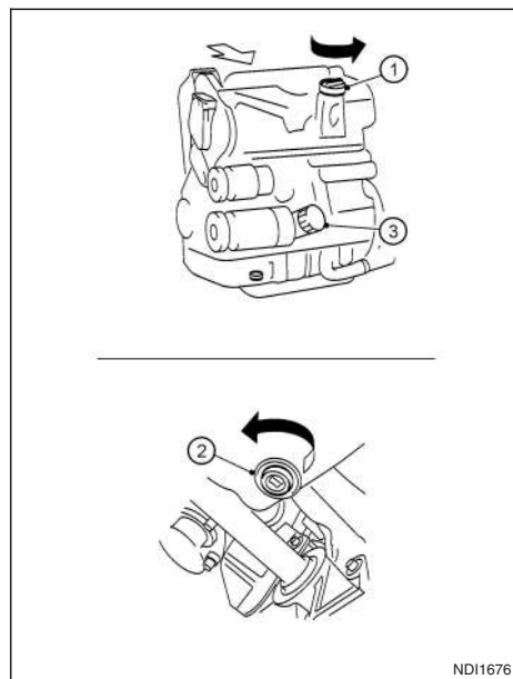
Modello con motore K9K
