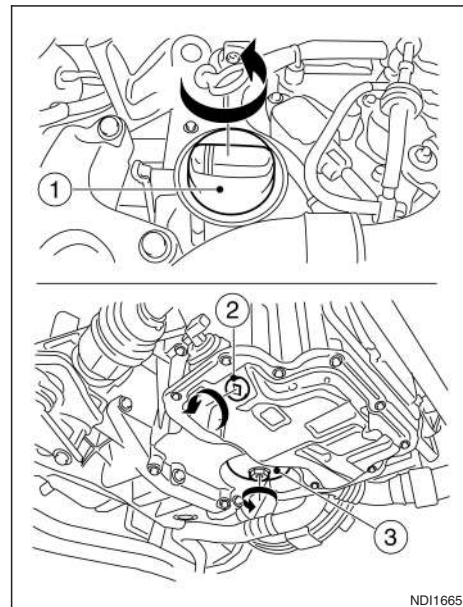
Modello con motore HR09DET, HR10DET e HR10DDT
