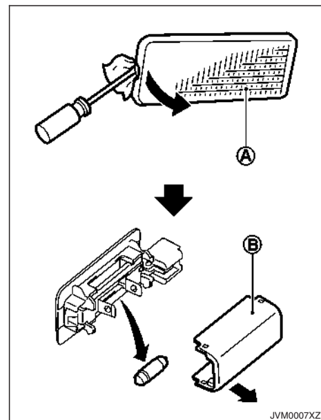
Luce bagagliaio (se in dotazione)
