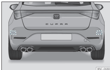
Fig. 162 Vista posteriore del veicolo: zone dei sensori radar.
