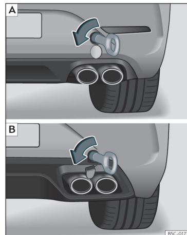
Fig. 50 Sul lato destro del paraurti posteriore: occhiello di traino avvitato. [A] Leon Sportstourer; [B] Leon.
