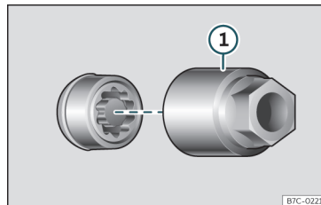
Fig. 40 Vite antifurto con cappuccio ed adattatore.
