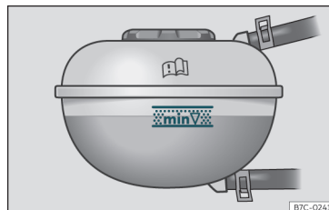
Fig. 217 Nel vano motore: segno nel serbatoio di compensazione del liquido di raffreddamento.
