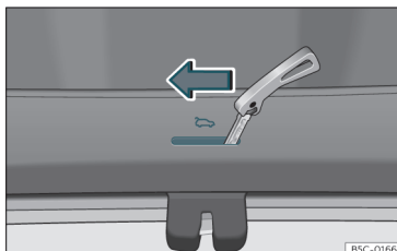
Fig. 89 Particolare del bagagliaio: sblocco di emergenza (Leon).
