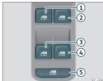
Fig. 91 Dettaglio della porta del conducente: comandi per i finestrini.
