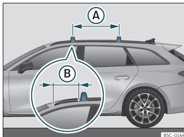
Fig. 136 Punti di fissaggio delle barre longitudinali per il portapacchi sul tetto (Leon Sportstourer).
