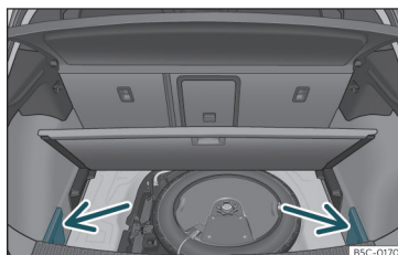
Fig. 116 Nel bagagliaio: coperchi per la rimozione del pianale.
