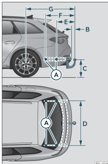
Fig.199 Quote e punti di fissaggio per il montaggio successivo di un dispositivo di traino.
