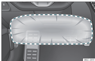
Fig. 22 Sul lato conducente: raggio d'azione dell'airbag per le ginocchia.
