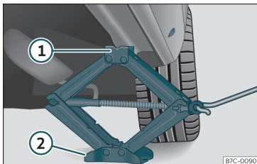
Fig. 43 Longherone: posizionamento del cric del veicolo.
