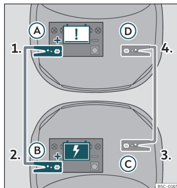
Fig. 46 Schema elettrico per i veicoli con sistema Start/Stop.
