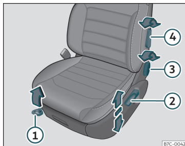
Fig. 104 Sedili anteriori: regolazione manuale del sedile.
