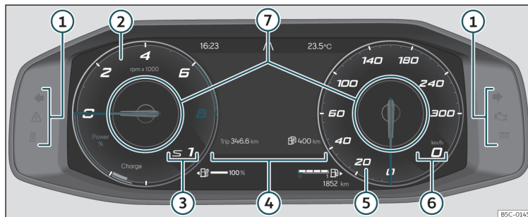
Fig. 56 Digital Cockpit nella plancia (visualizzazione classica).
