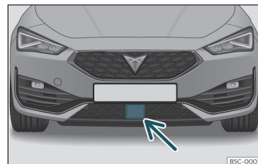
Fig. 159 Sul paraurti anteriore: sensore radar.
