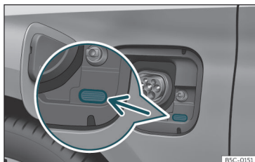
Fig. 203 Dietro il coperchio della presa di ricarica della batteria: indicatore del processo di ricarica.
