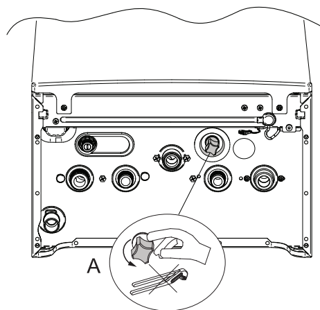
Fig.27 Llenado de la instalación
