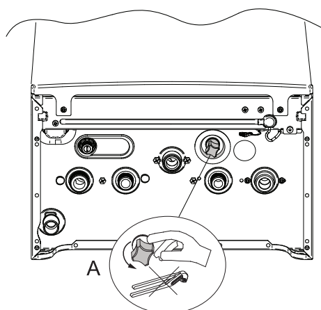
Fig.34 Caricamento impianto
