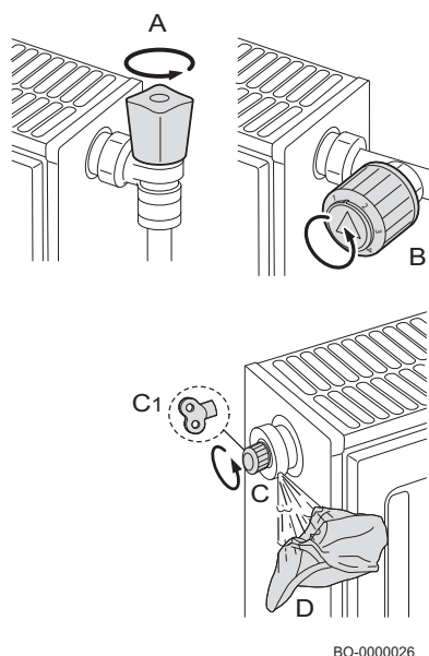
Fig.35 Deareazione impianto
