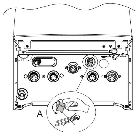
Εικ.13 Πλήρωση της εγκατάστασης
