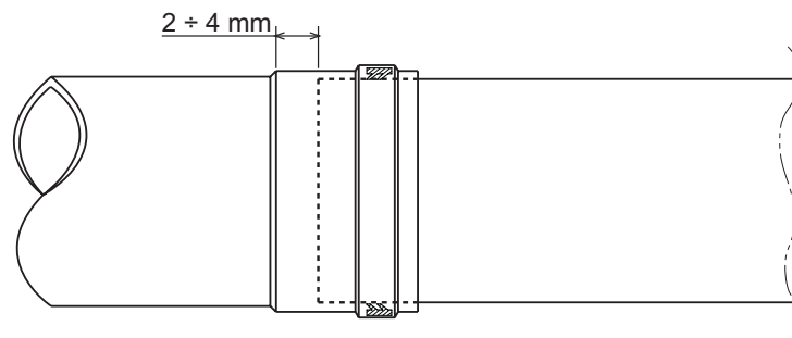
fig. 21 - Dilatazione
