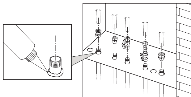
fig. 20 - Sigillatura involucro
