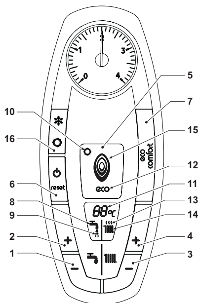
fig. 1 - Pannello di controllo
