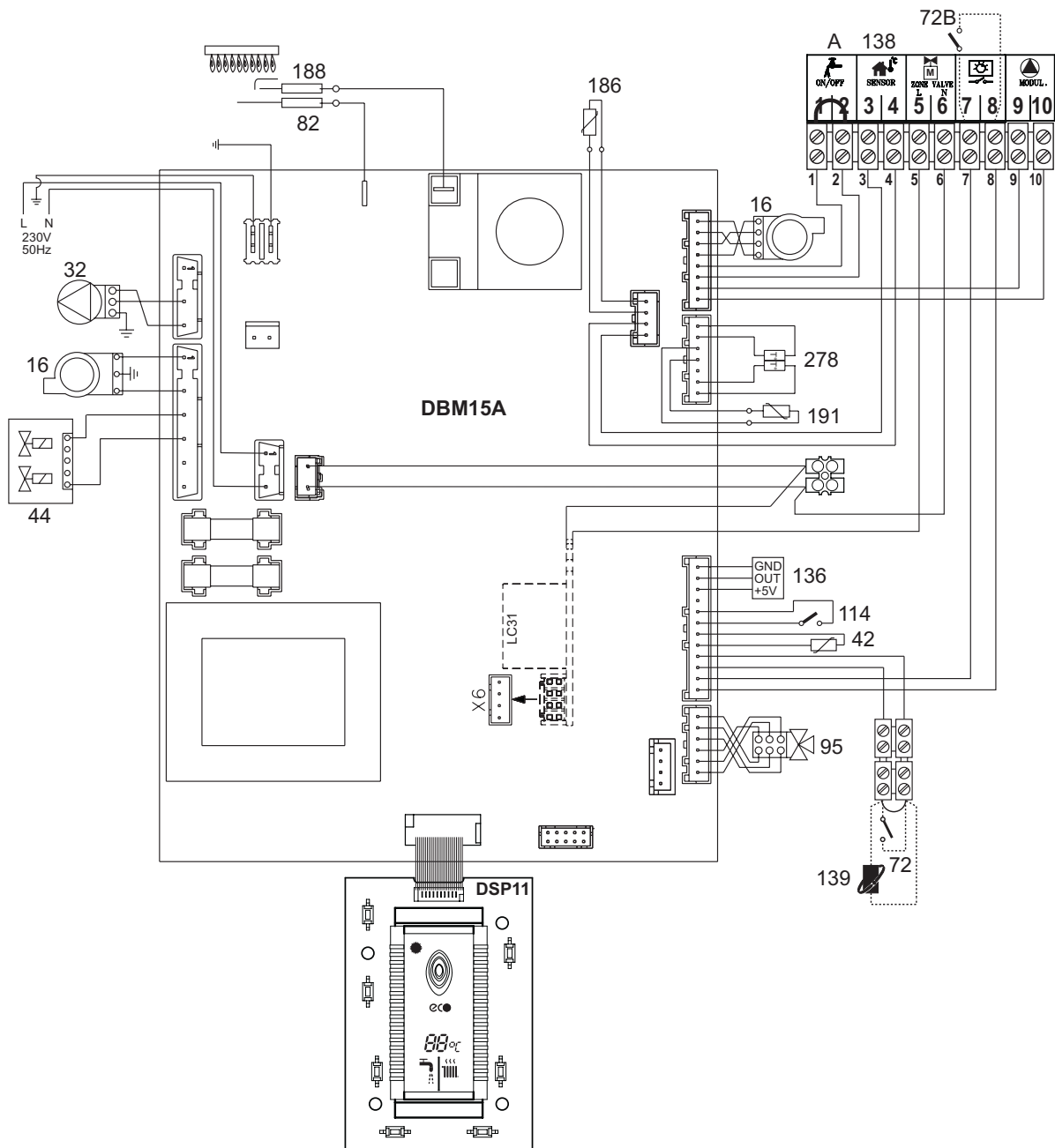
fig. 36 - Schema elettrico
