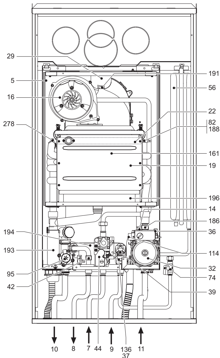
fig. 34 - Vista generale
