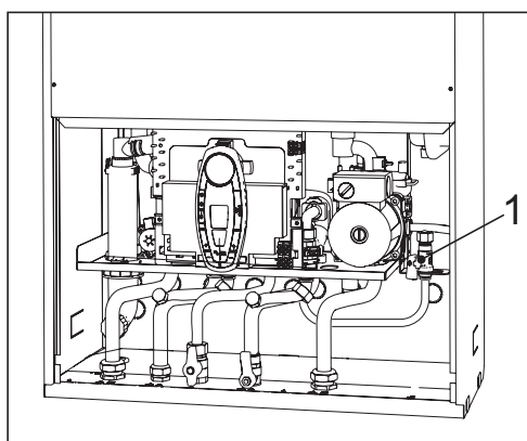
fig. 16 - Rubinetto di carico
