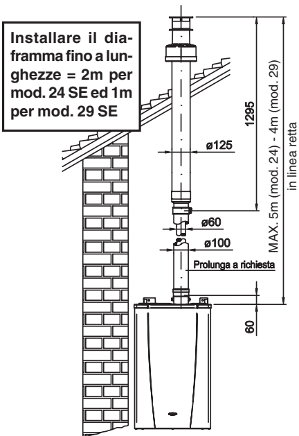
KIT FUMI COASSIALE VERTICALE
