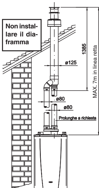
KIT FUMI VERTICALE SDOPPIATO
