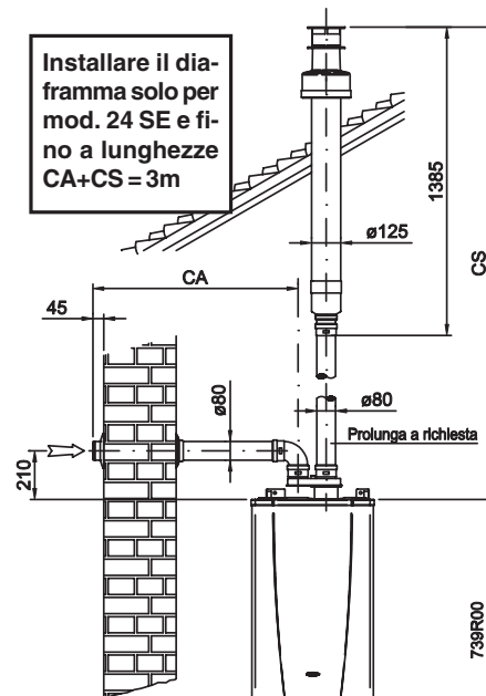
KIT FUMI VERTICALE SOLO SCARICO
