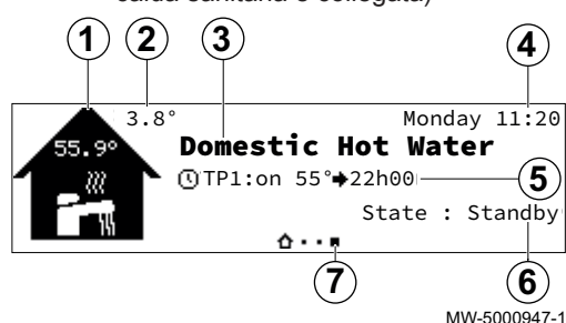
Fig.8 Schermata iniziale per la visualizzazione dell'acqua calda sanitaria (solo se la sonda acqua calda sanitaria è collegata)
