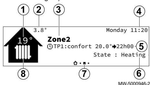
Fig.7 Schermata iniziale Zone2 (solo se la PCB opzionale SCB-04 è collegata)
