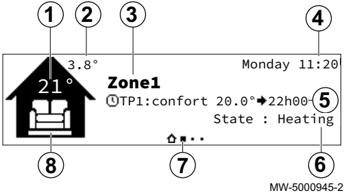
Fig.6 Schermata iniziale Zone1
