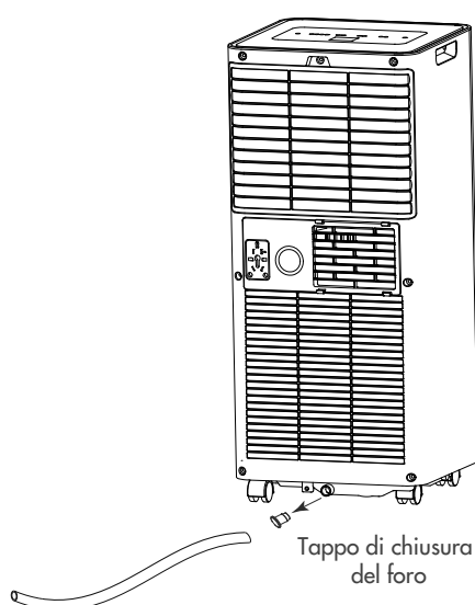
Drenaggio condensa manuale (Raffrescamento)
