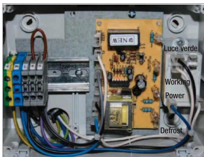
Fig. 4-4 Il quadro elettrico con la scheda elettronica
