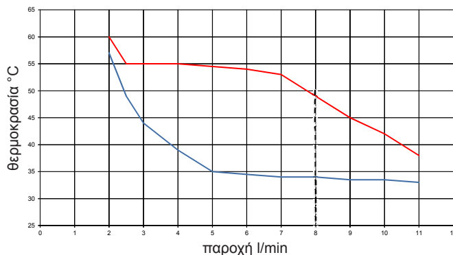
Διάγραμμα IDRABAGNO 11 ESI
