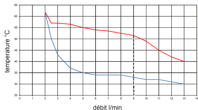
Diagramme IDRABAGNO 13 ESI
