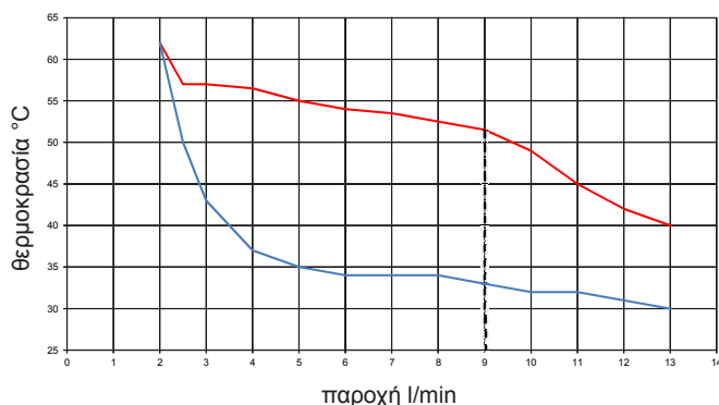
Διάγραμμα IDRABAGNO 13 ESI
