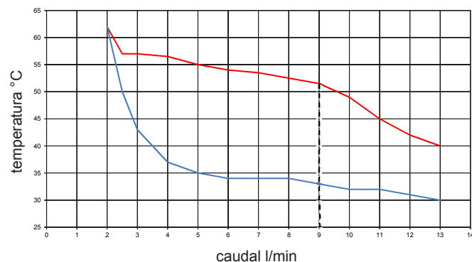
Diagrama IDRABAGNO 13 ESI
