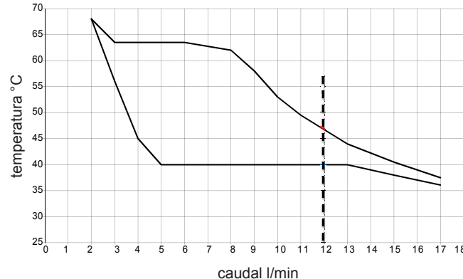
Diagrama de IDRABAGNO 17 ESI
