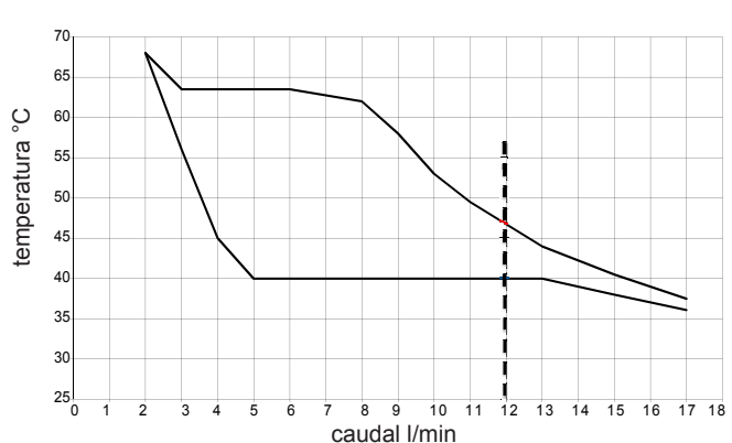
Diagrama IDRABAGNO 17 ESI
