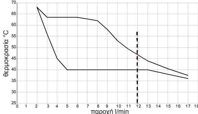
Διάγραμμα IDRABAGNO 17 ESI
