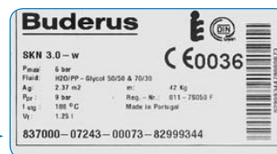
Esempio targhetta collettore solare
