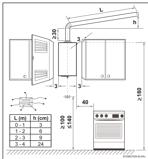
Fig. 11 Distanze minime
