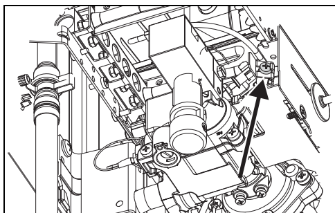
Fig. 14 Vite per regolazione della pressione minima
