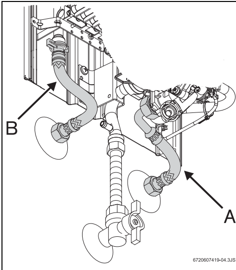
Fig. 11 Collegamento acqua
