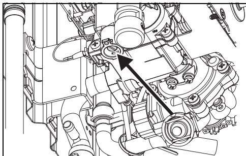
Fig. 13 Vite per regolazione della pressione massima
