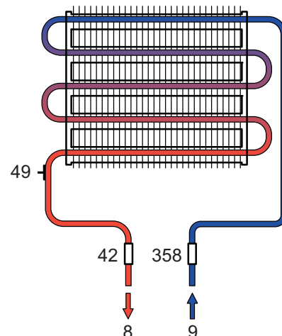
fig. 15 - Circuito idraulico
