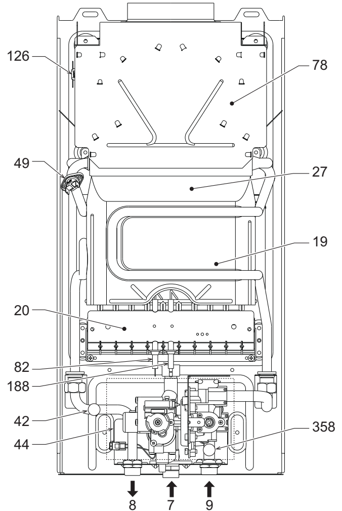
fig. 14 - Vista generale
