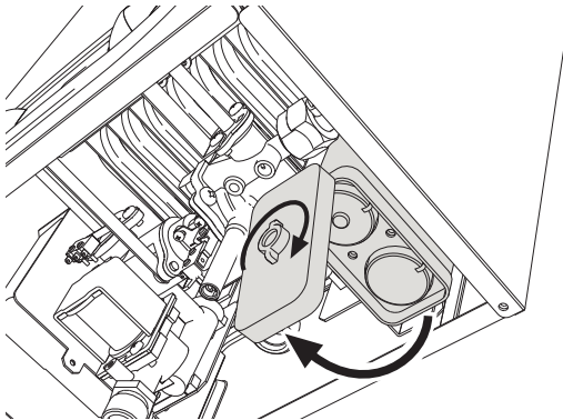
fig. 12 - Sostituzione batterie
