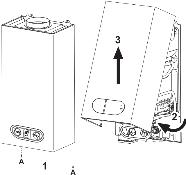
fig. 11 - Apertura mantello
