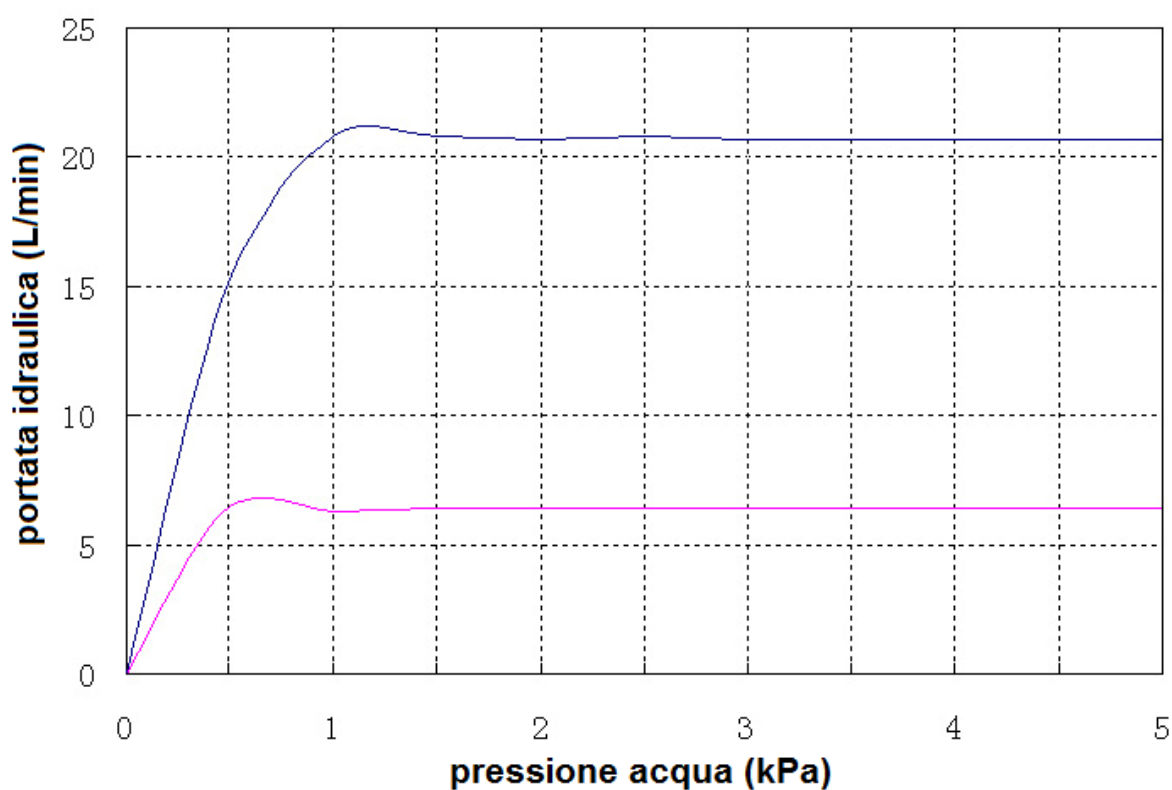
Infinity REU-1720FFU
