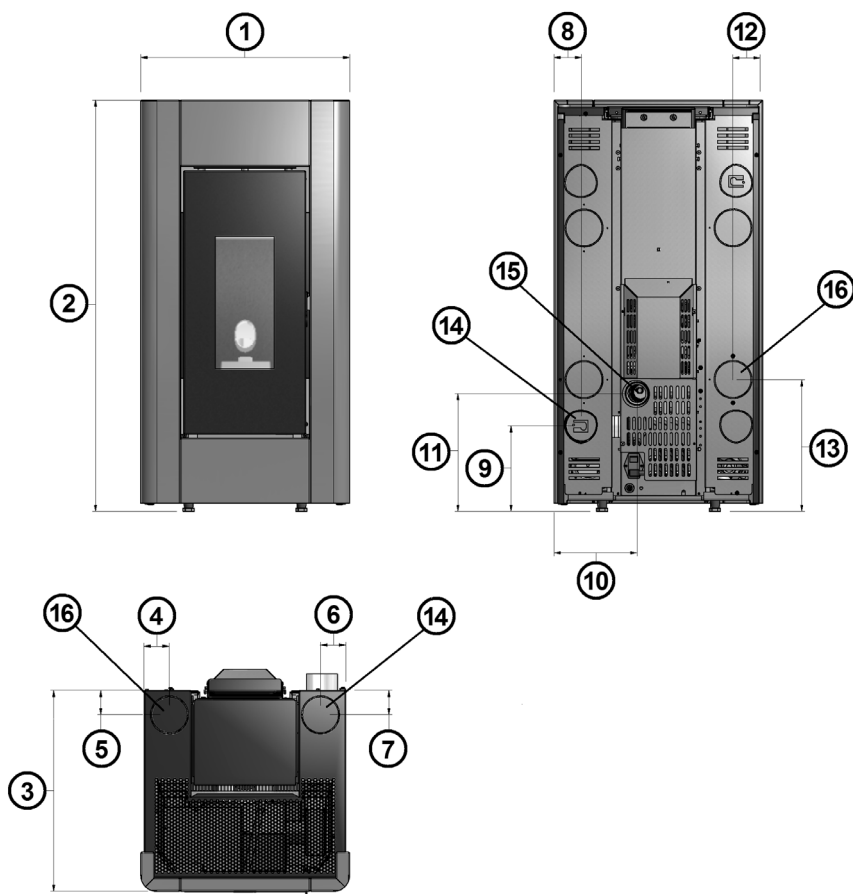
Fig. 19 - Dimensioni generali: Prince³ 11KW / Prince³ Plus 11KW
