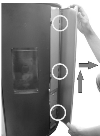
Fig. 80 - Sfera 3 / Sfera 3 Plus: sganciare i pannelli laterali
