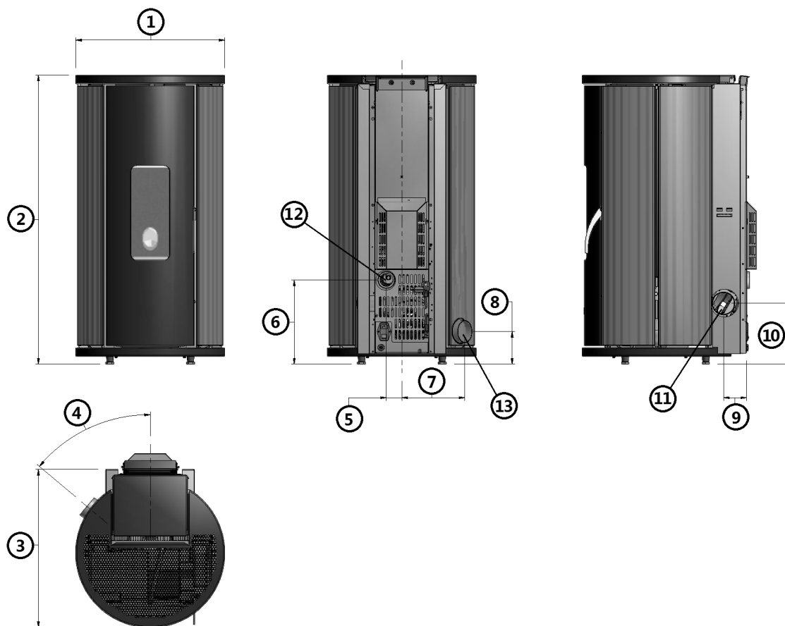
Fig. 18 - Dimensioni generali: Sfera³ 11 KW/Sfera³ Plus 11KW/Globe At
