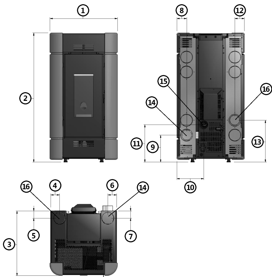
Fig. 16 - Dimensioni generali: Sire³ Plus 11KW
