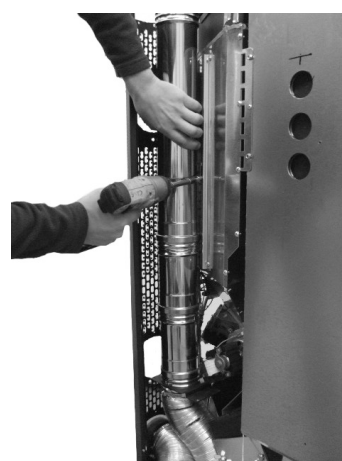
Fig. 64 - Fissaggio tubo
