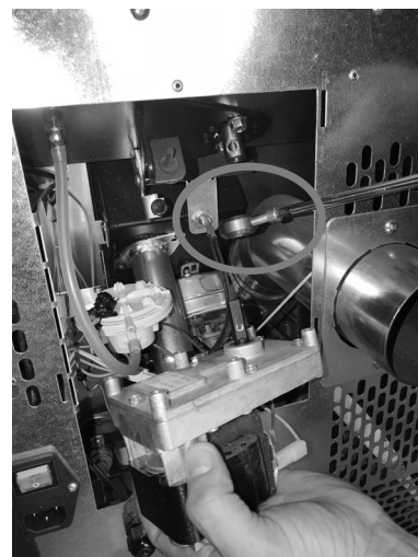
Fig. 72 - Rimozione motoriduttore
