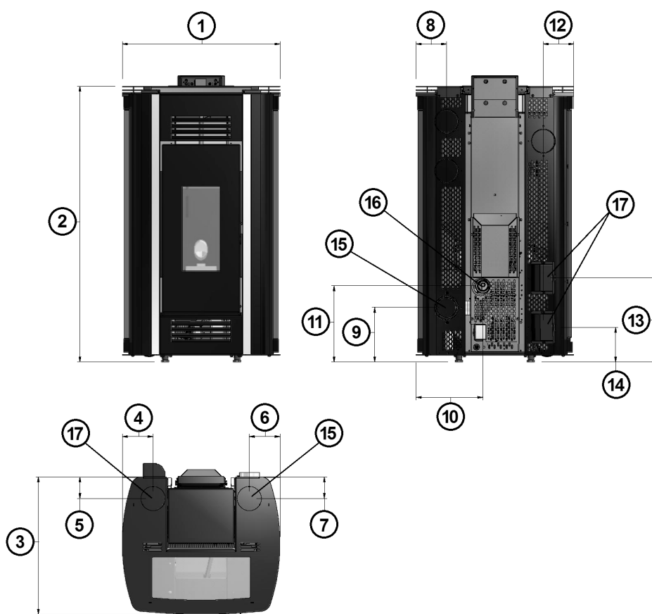
Fig. 21 - Dimensioni generali: Venus³ Plus 12,5KW
