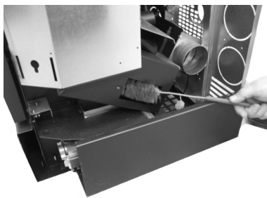
Fig. 100 - Pulizia con scovolino 2
