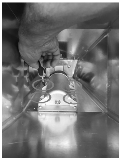
Fig. 70 - Rimozione viti
