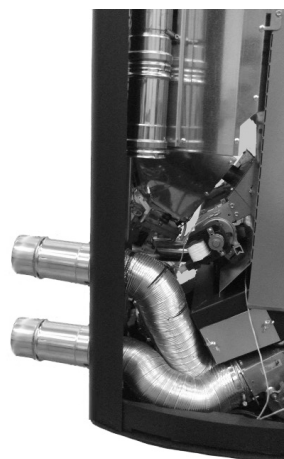
Fig. 67 - Fissaggio tubi
