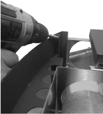
Fig. 44 - Rimozione profili curvi superiori
