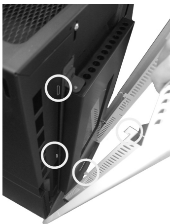
Fig. 24 - Montaggio cornice
