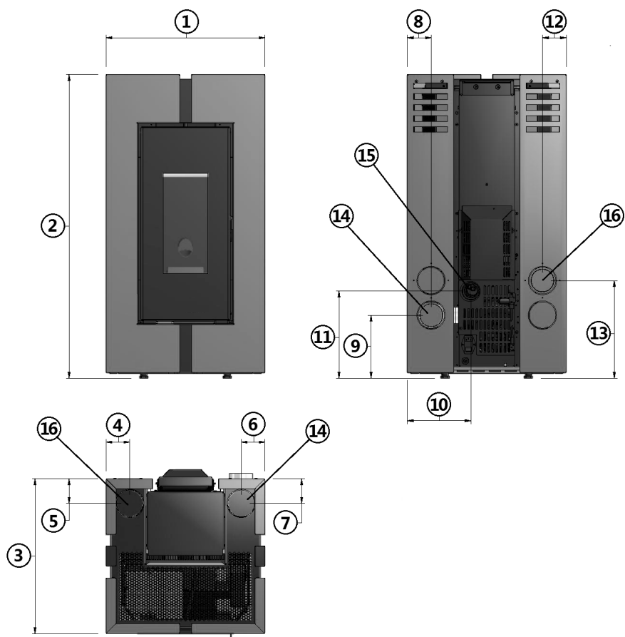
Fig. 17 - Dimensioni generali: Doge³ Plus 11KW
