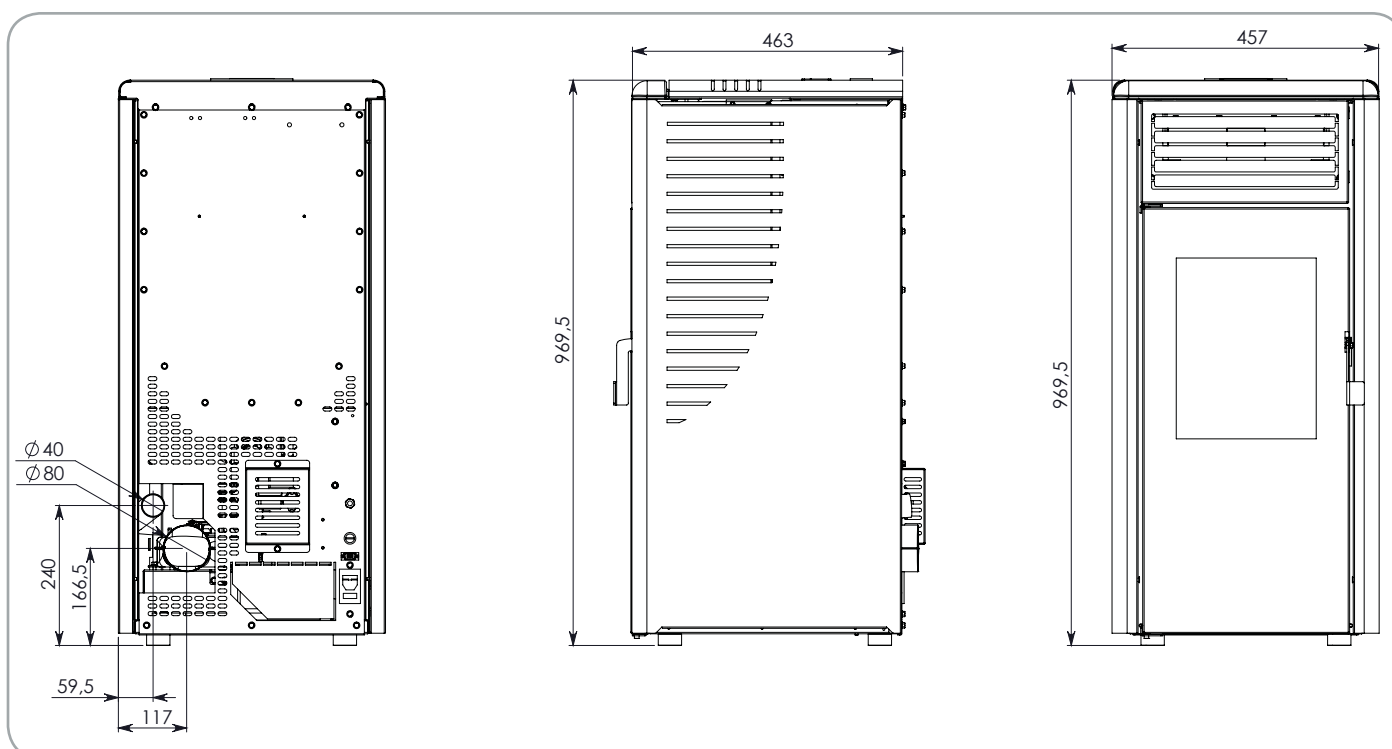
Tavola tecnica Fusion 8
