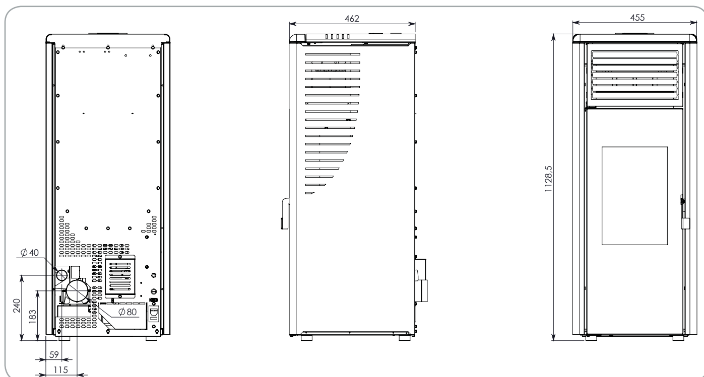
Tavola tecnica Fusion 12
