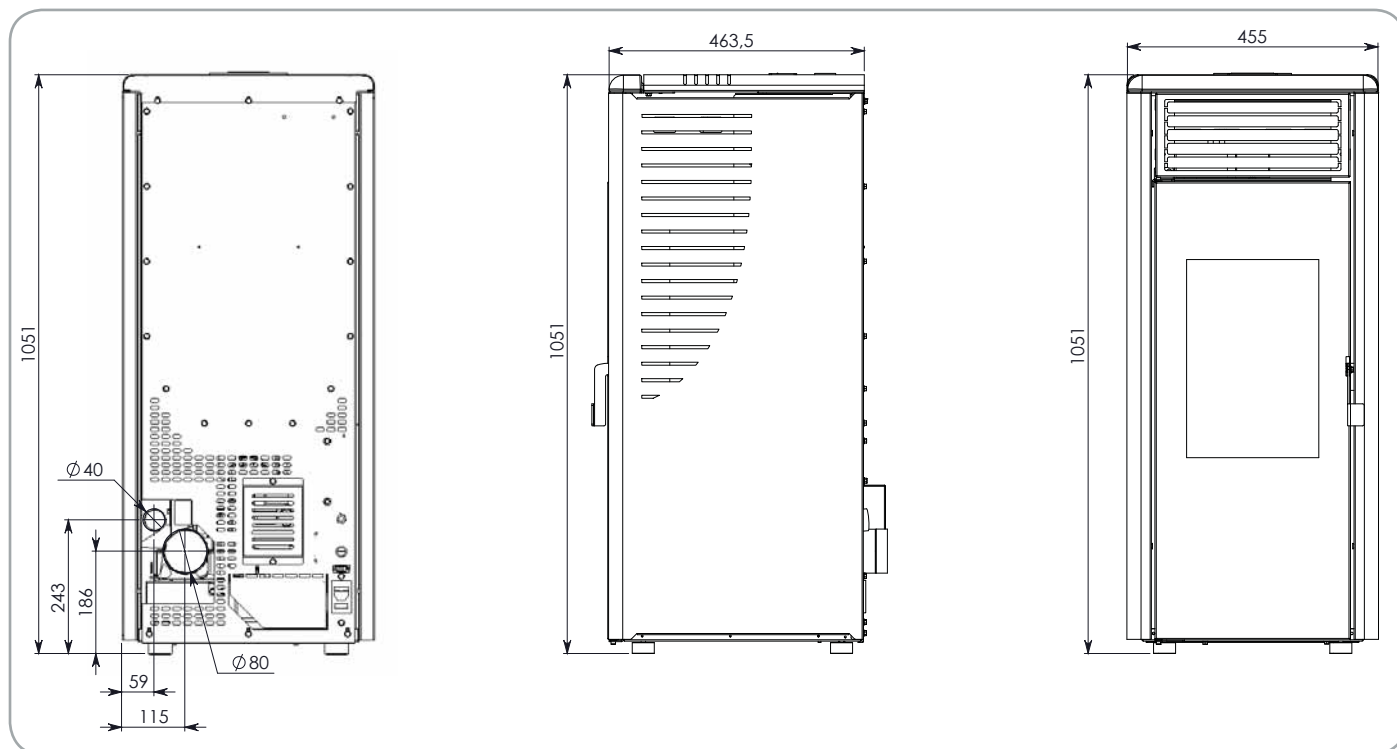
Tavola tecnica Fusion 10
