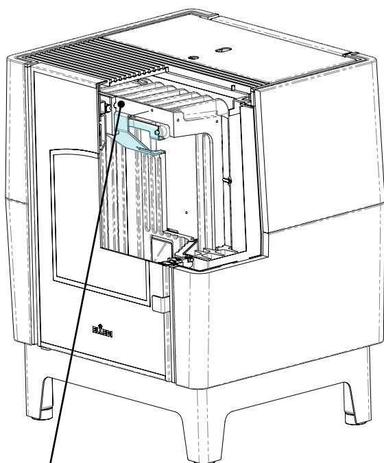
Corta-fogo no alojamento
