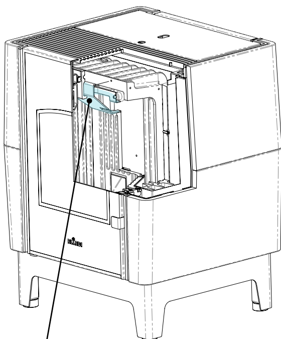
Corta-llama en su alojamiento
