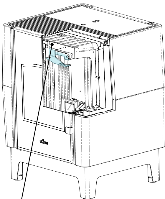
Tagliafiamma in sede
