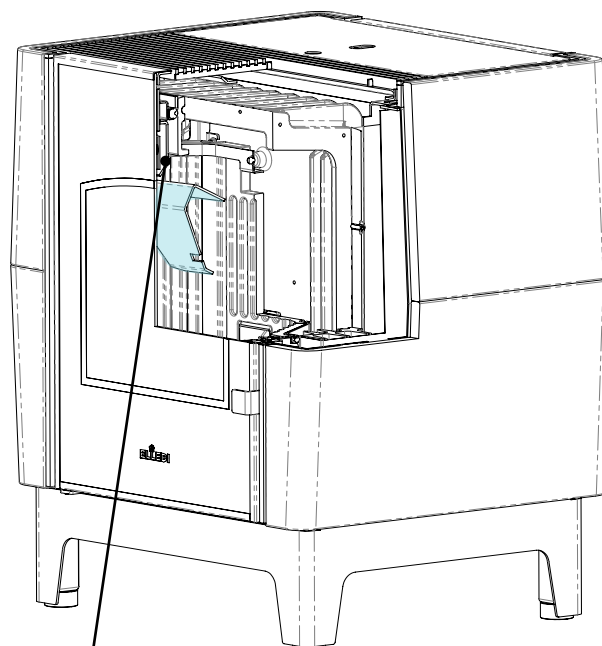
Tagliafiamma estratto
