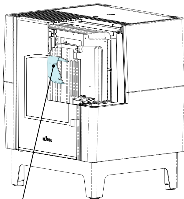
Corta-llama sacada
