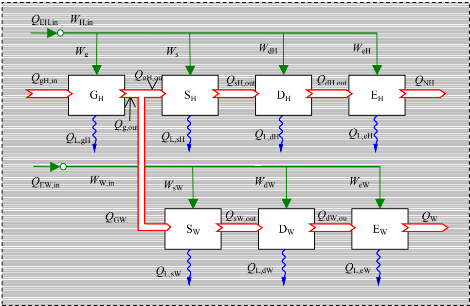
Figura 7 – Schema di calcolo dell'energia primaria per impianti combinati per la climatizzazione invernale e la produzione di acqua calda sanitaria (Fonte: prEN 15316)
