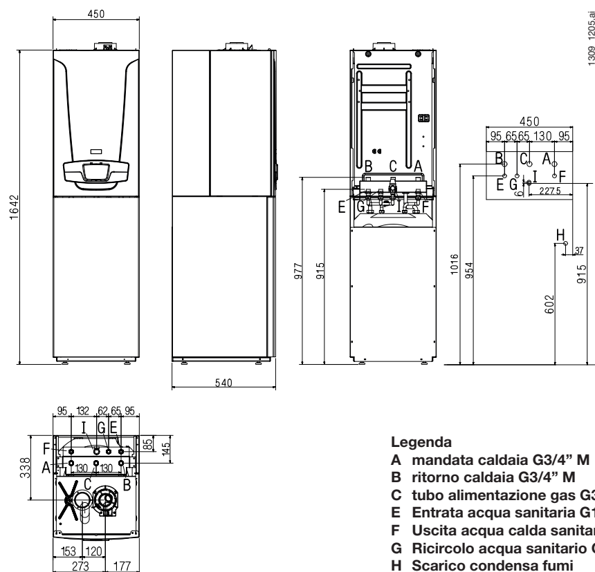
Dimensioni apparecchio
