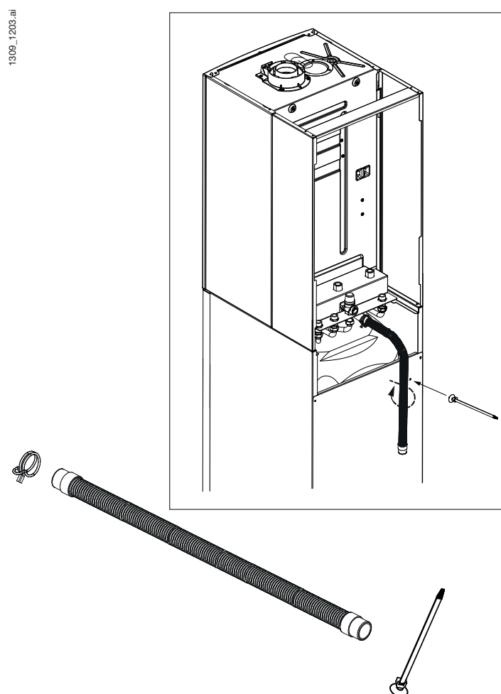
Figura 1B. Sequenza montaggio apparecchio
