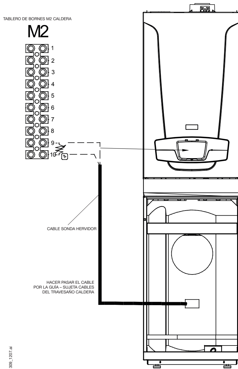
Figura 3: Conexión sonda precedencia sanitario
