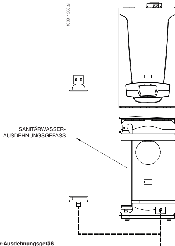
Abb. 4: Sanitärwasser-Ausdehnungsgefäß
