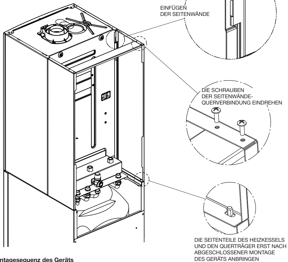
Abb. 1C: Montagesequenz des Geräts
