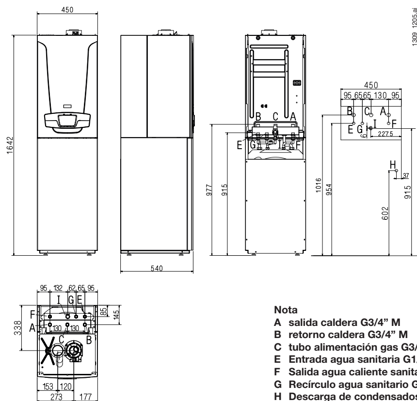
Dimensiones aparato
