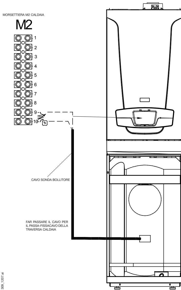
Figura 3: Collegamento sonda precedenza sanitario
