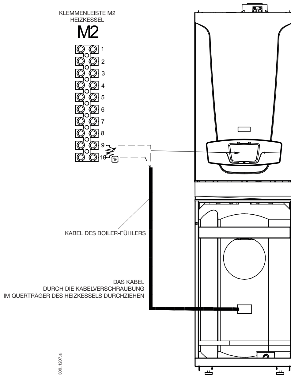
Abb. 3: Anschluss des Sanitärwasser-Prioritätsfühlers
