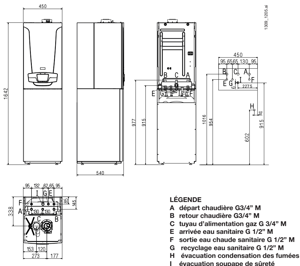
Dimensions de l'appareil
