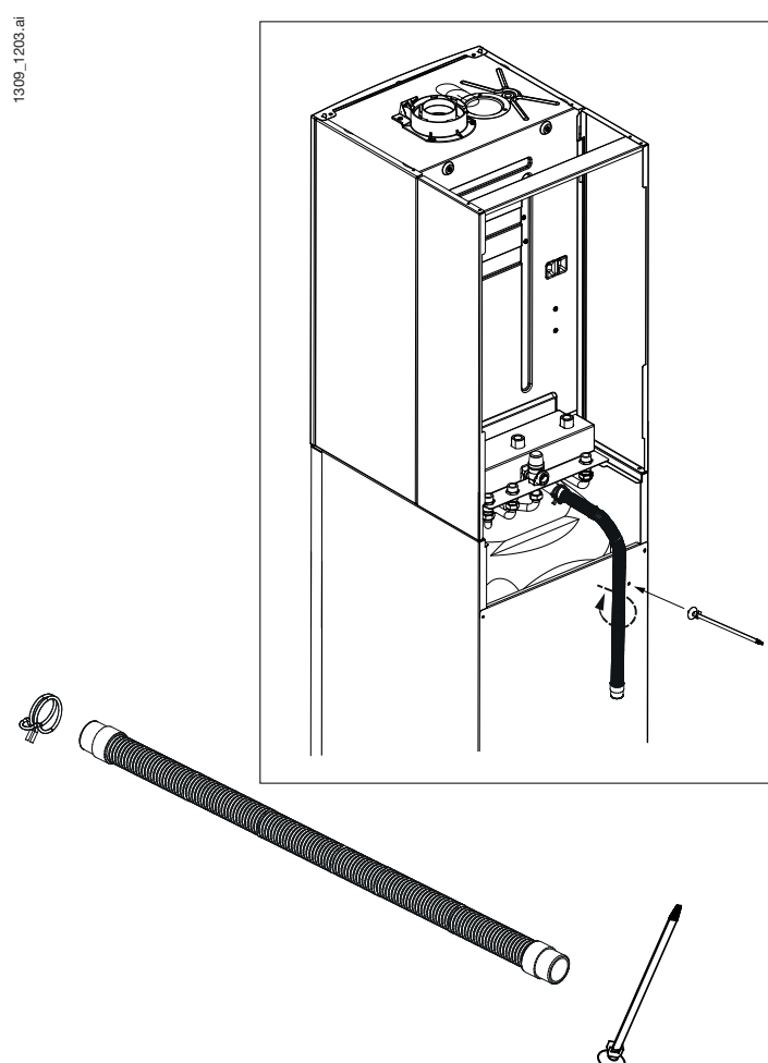
Figura 1B. Secuencia montaje aparato
