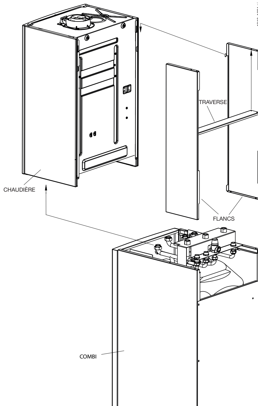
Figure 1A. Séquence de montage de l'appareil
