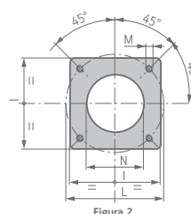
Dimensioni flangia e dima di foratura caldaia.
