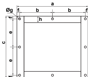
D...-TRON 4-5
