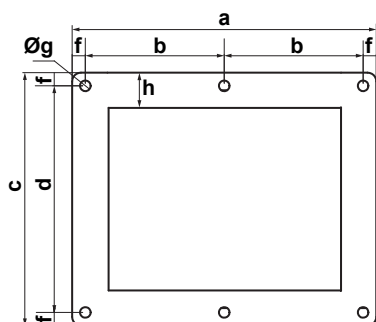
D...-TRON 2-3
