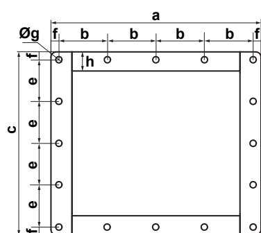
D...-TRON 8
