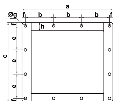
D...-TRON 7
