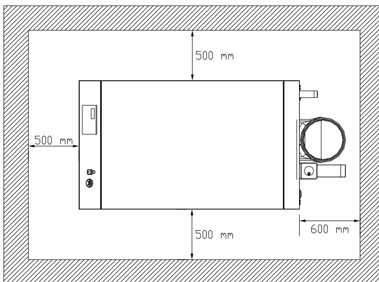
Distanze minime da rispettare ai lati della caldaia.
