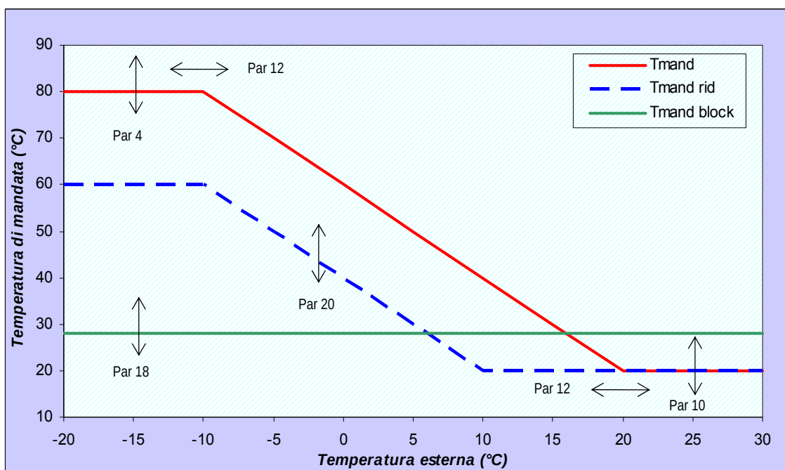
Curva standard di riscaldamento
