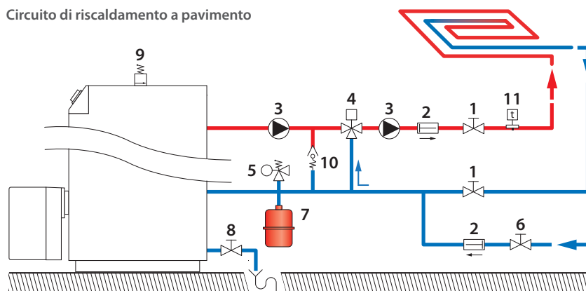
Circuito di riscaldamento a pavimento
