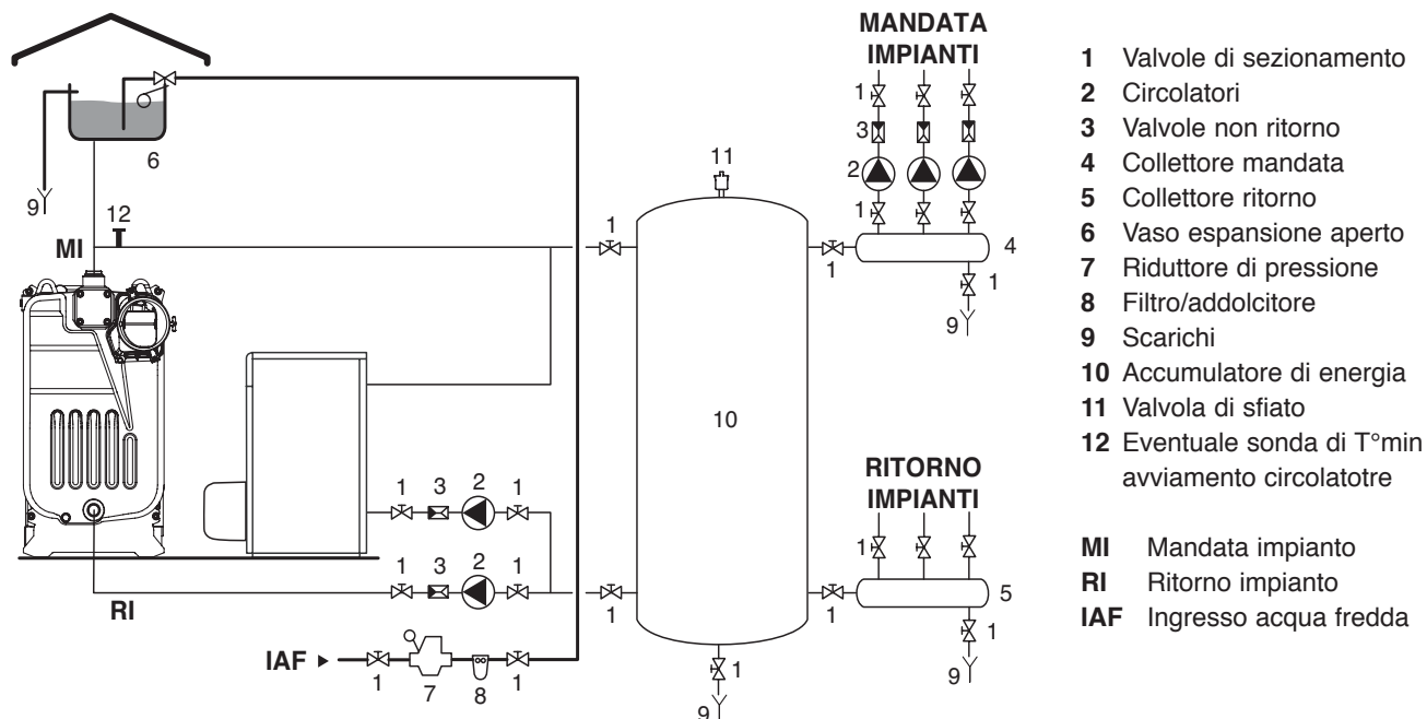
Schema 3: caldaia 3WOOD, abbinata ad altra caldaia, con accumulatore di energia per alimentare gli impianti
