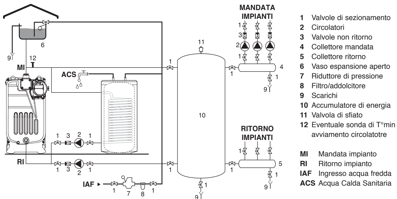
Schema 4: caldaia 3WOOD, abbinata ad un bollitore ACS, con accumulatore di energia per alimentare gli impianti
