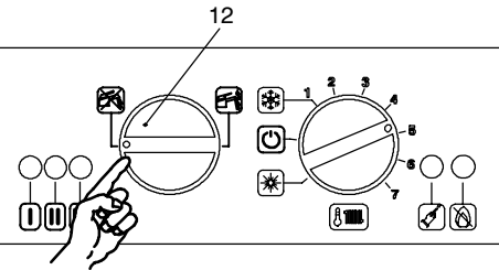
fig. 2.9 Nel caso si voglia escludere l'uso del serbatoio dinamico sanitario (non mantenerlo in temperatura) e mantenere attiva la caldaia nel solo funzionamento riscaldamento, ruotare la manopola settaggio serbatoio dinamico 12 come illustrato in fig. 2.9 Nel caso si preveda un lungo periodo di inattività del serbatoio dinamico: 1 Chiudete il rubinetto entrata acqua sanitaria 8 in fig. 2.8; 2 provvedete allo svuotamento del serbatoio dinamico e del circuito idraulico sanitario vedi sez.9.3 a pag.38
