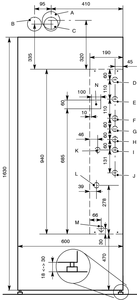
fig. 5.2 (tutte le misure sono in mm) A – espulsione fumi/aspirazione aria (coassiale ø 100/60) B – espulsione fumi (sdoppiato ø 80) C – aspirazione aria (sdoppiato ø 80)
