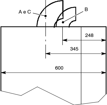
fig. 5.3 (tutte le misure sono in mm)
