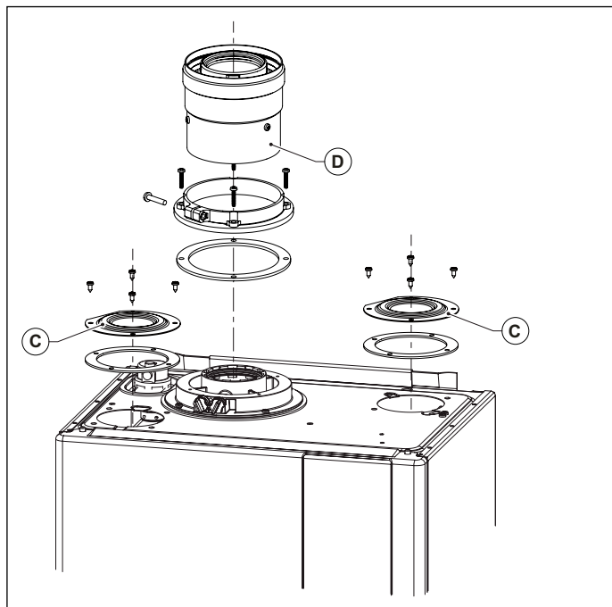
Fig. 2 Installazione kit coassiale
