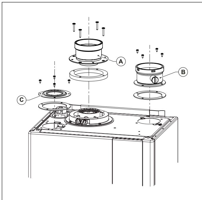
Fig. 1 Installazione kit sdoppiato
