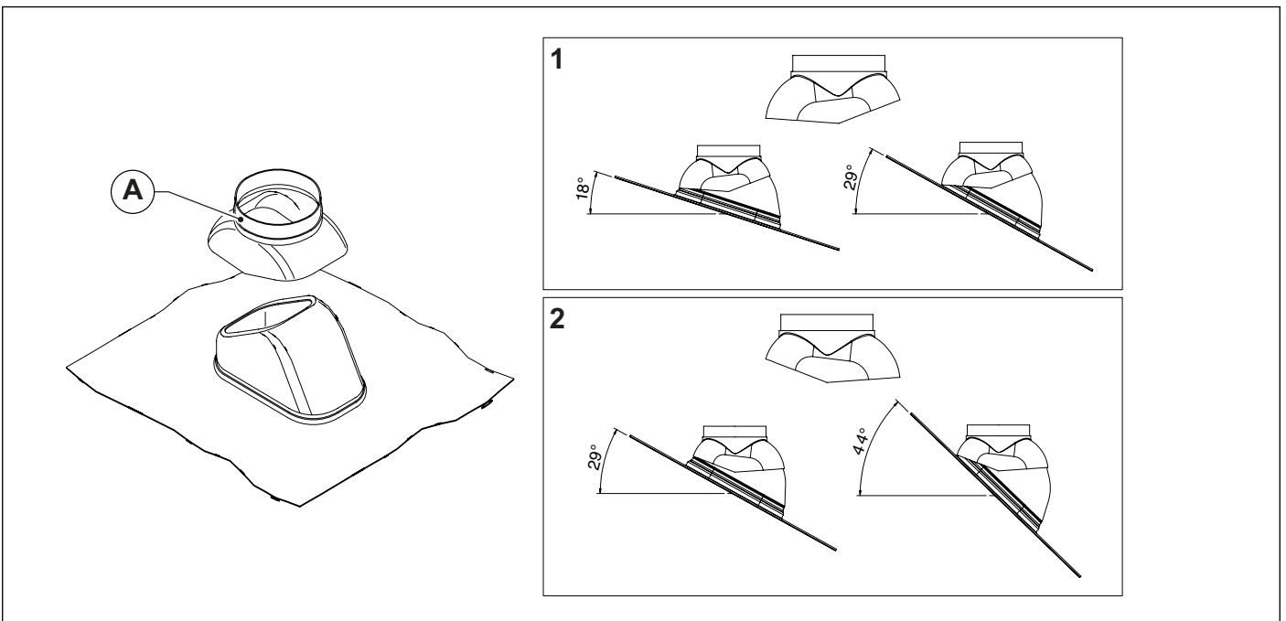
Fig. 6 Tegola per tetti inclinati
