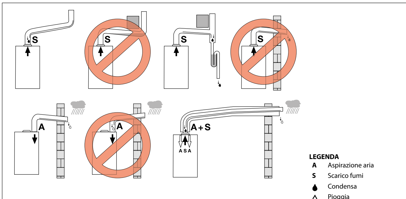
Fig. 3 Esempi di installazione
