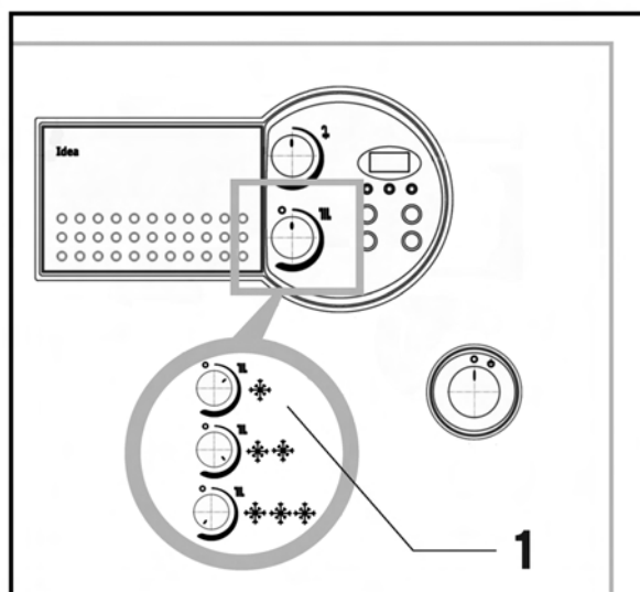
Fig. 4.6 Temperatura di mandata - Impostazione sulla caldaia
