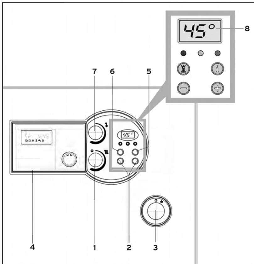
Fig. 4.2 Elementi di comando
