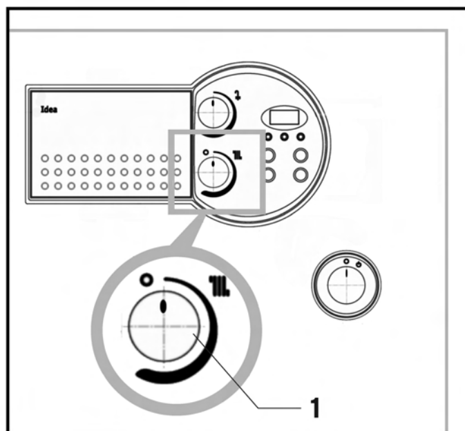
Fig. 4.5 Impostazione della temperatura di mandata mediante un dispositivo di regolazione
