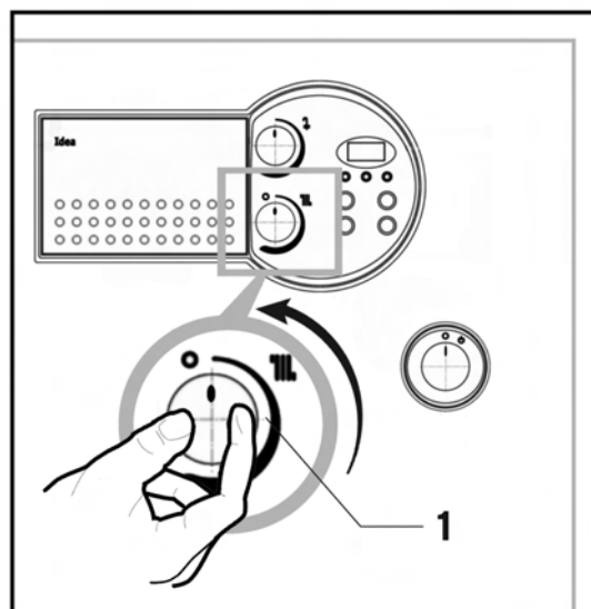
Fig. 4.7 Disattivazione della modalità di riscaldamento (modalità estiva)
