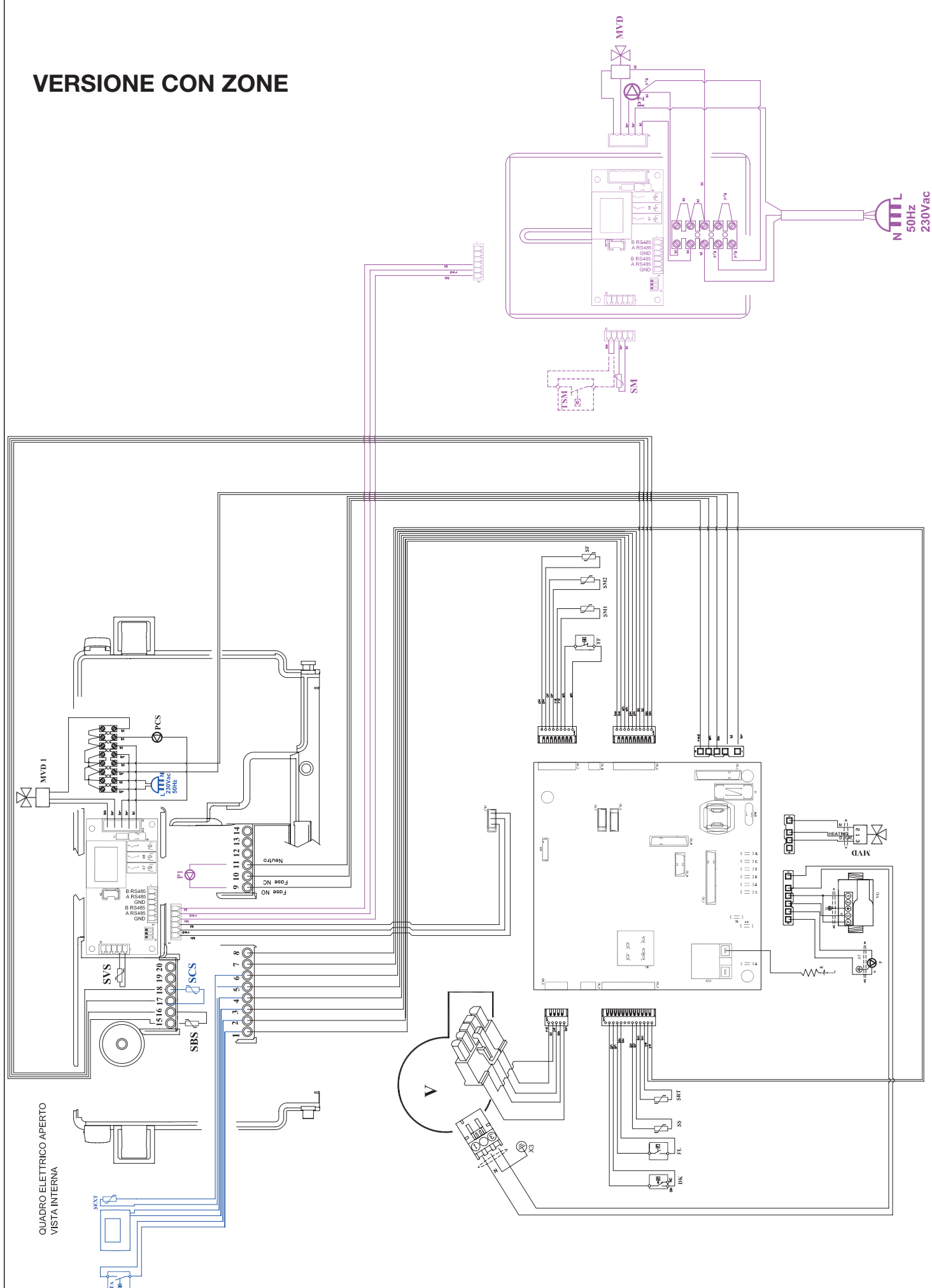
fig. 25 - Schema elettrico
