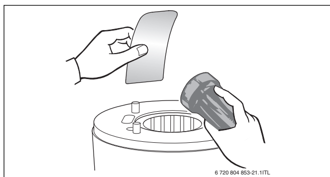
Fig. 52 Controllo della presenza di residui nello scambiatore primario
