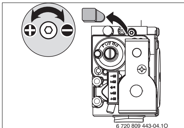
Fig. 41 Rimozione del sigillo
