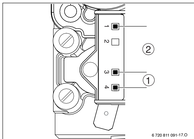
Fig. 60 Punti di misurazione sulla valvola del gas
