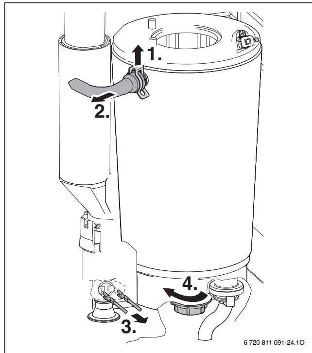
Fig. 65 Smontaggio del tubo di mandata e scollegamento dei cavi
