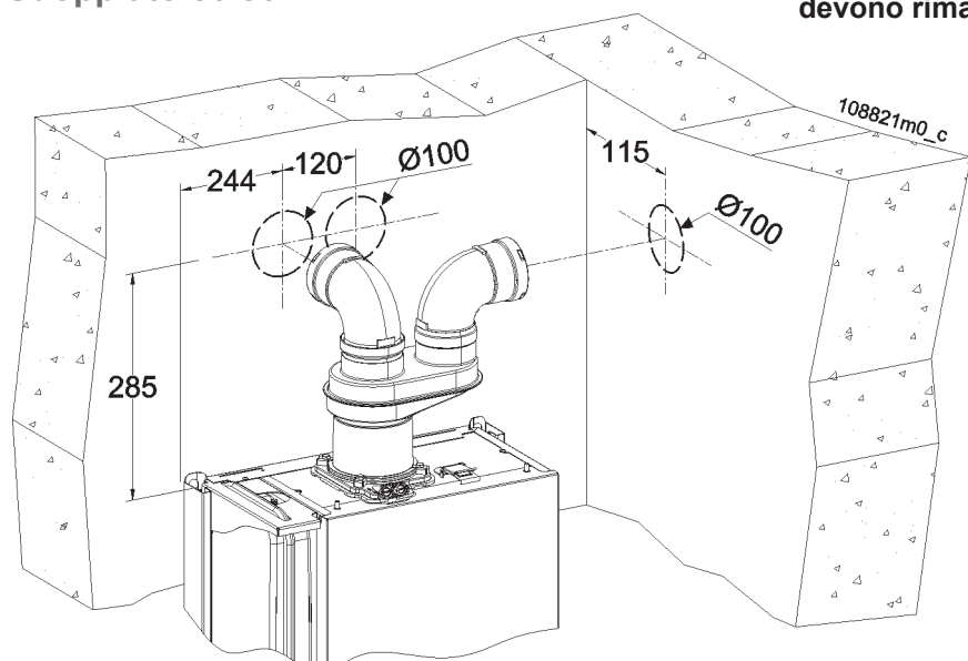
Figura 5-11 - Quote interassi dello scarico "Sdoppiato 80/80 PP"
