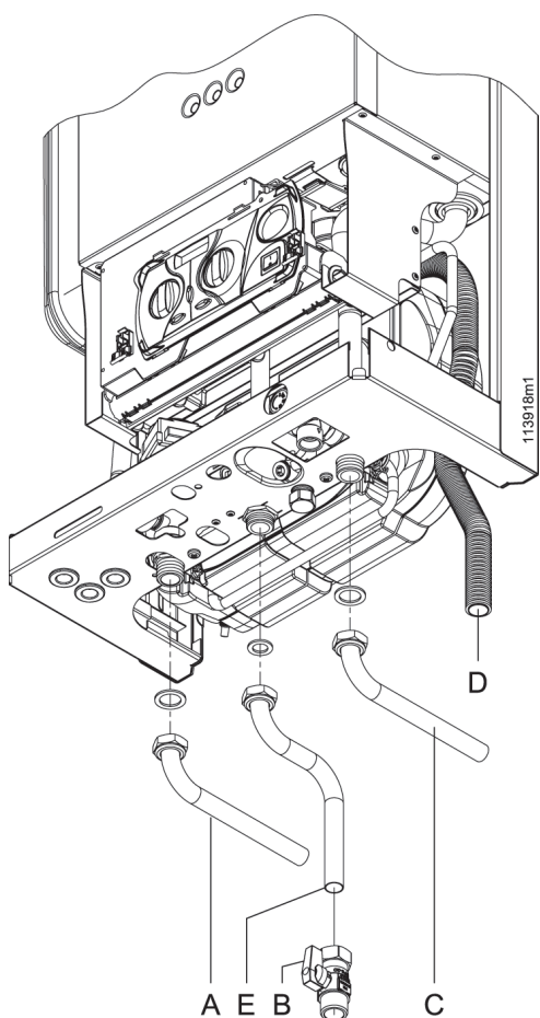
Figura 5-4 - Connessioni idrauliche e gas
