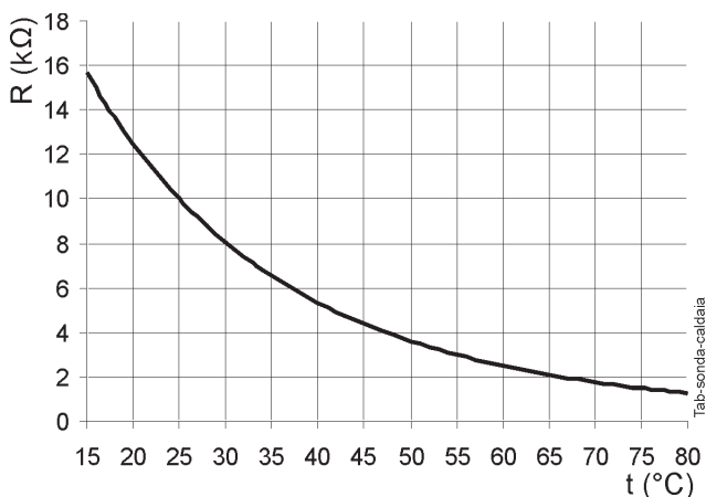
Figura 8-7- Curva sensori acqua
