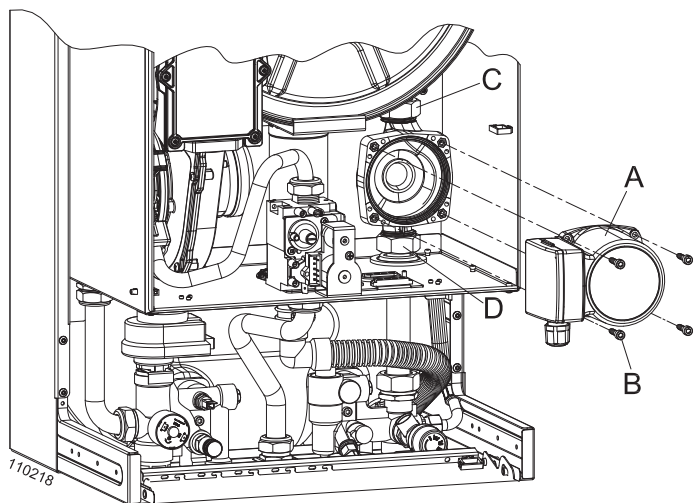
Figura 8-5 - Sostituzione del motore della pompa
