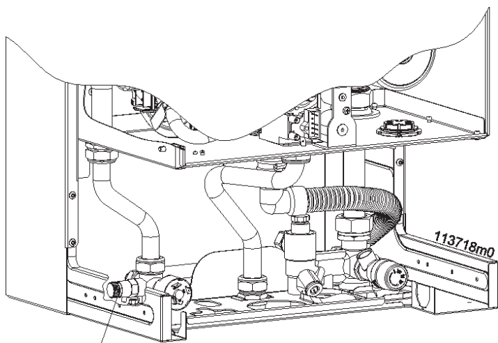
Figura 8-6 - Rubinetto di scarico circuito riscaldamento
