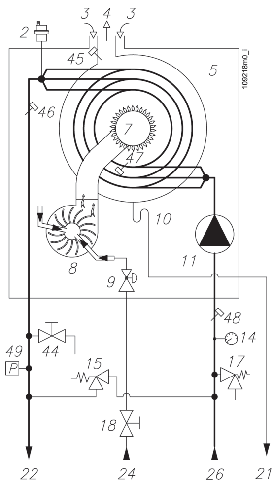
Figura 4-1 - Schema idraulico CIELODENS 45C
