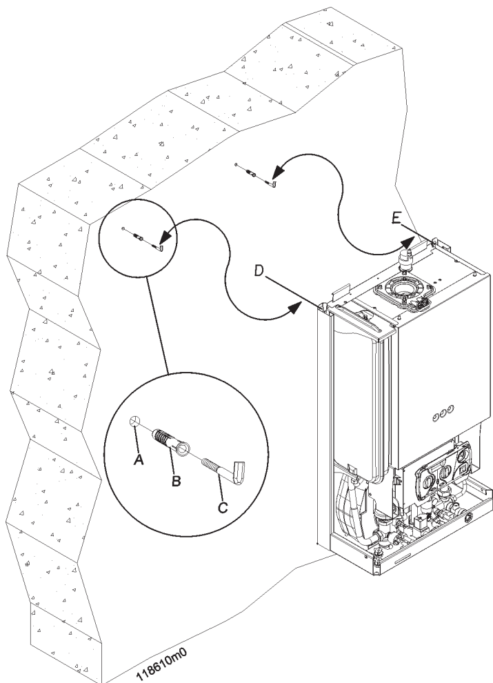
Figura 5-3 - Tasselli di sostegno
