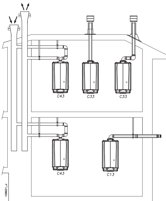
Figura 5-9 - Sistemi di scarico/aspirazione
