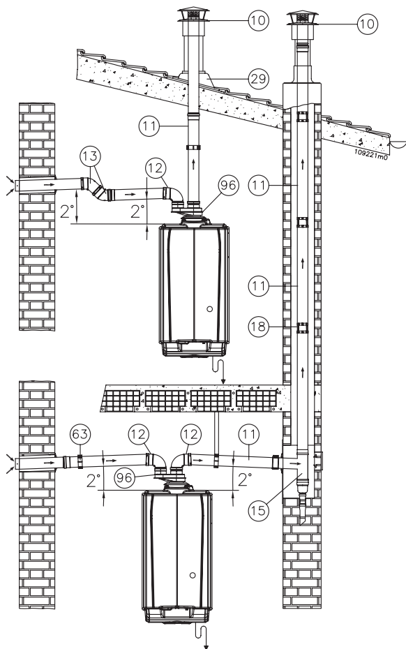
Figura 5-12 - Esempio di installazione "Sistema 80/80 PP"
