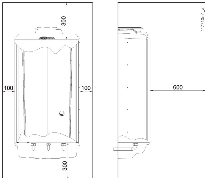
Figura 5-1 - Distanze minime di rispetto
