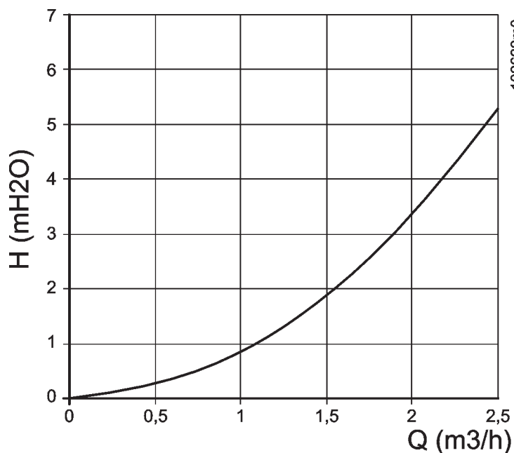
Figura 4-4 - Resistenze idrauliche della CIELODENS 45A (priva di pompa)
