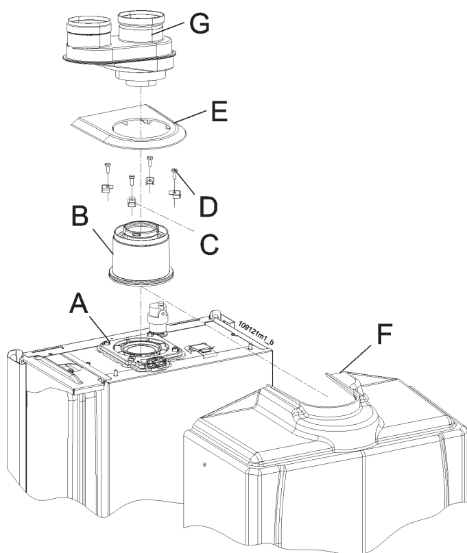
Figura 5-10 - Installazione del sistema "Sdoppiato 80/80 PP"
