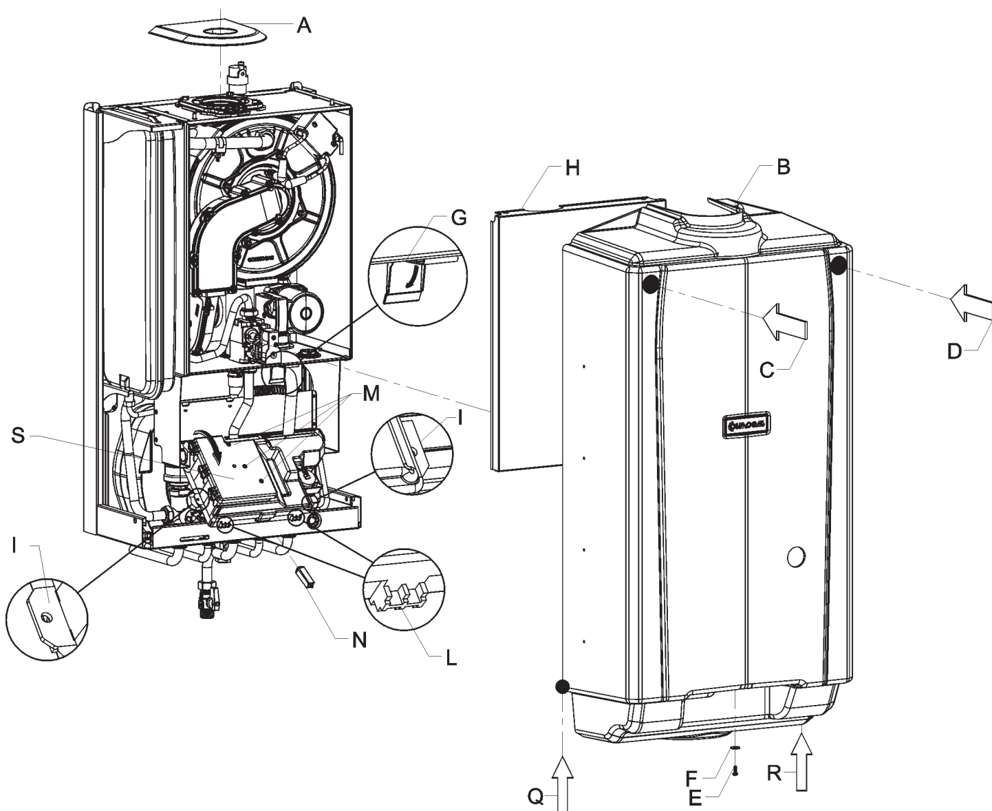
Figura 8-1 - Montaggio e smontaggio della mantellatura e accesso ai componenti interni
