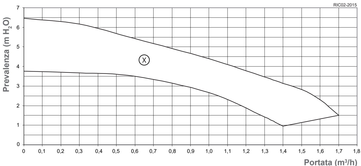
Figura 4-3 - Diagramma della prevalenza residua all'impianto per il modello 45C (con pompa integrata) (la "X" corrisponde al campo di modulazione del circolatore)
