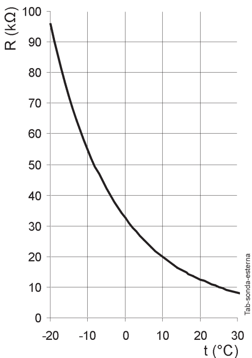
Figura 8-8 - Curva sensore temperatura esterna
