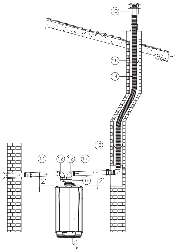
Figura 5-13 - Esempio di installazione "Sistema 80/80 PP"
