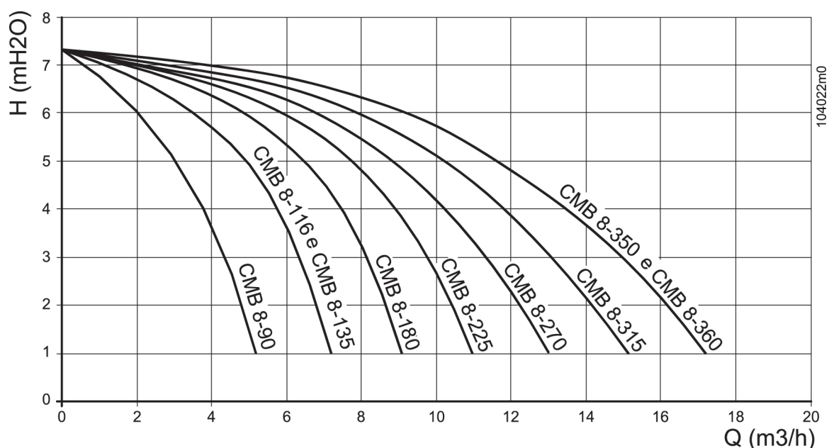
Figura 5b - Diagramma della prevalenza residua all'impianto, senza disconnettore idraulico
