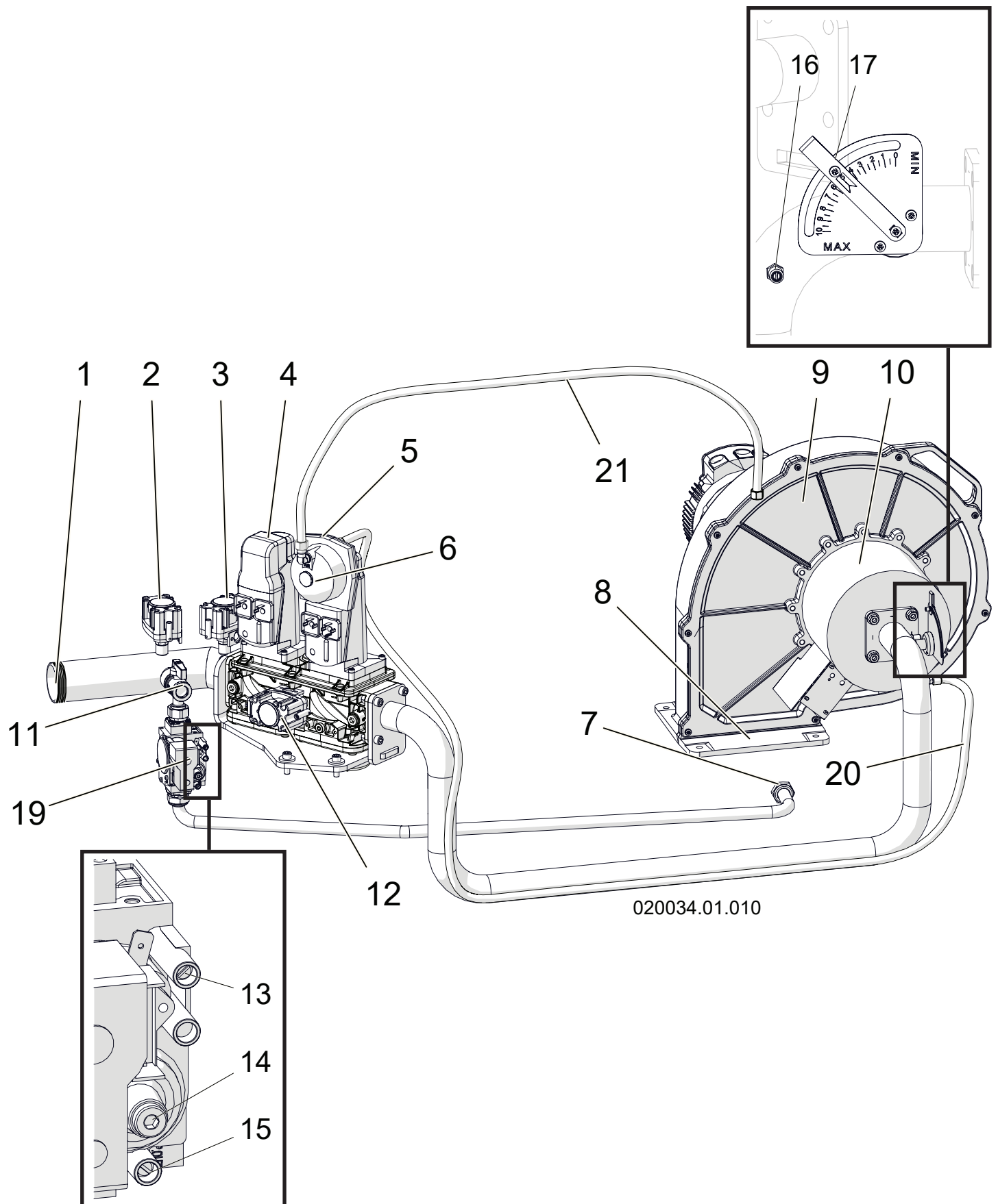
Figura 5-8 - Circuito gas
