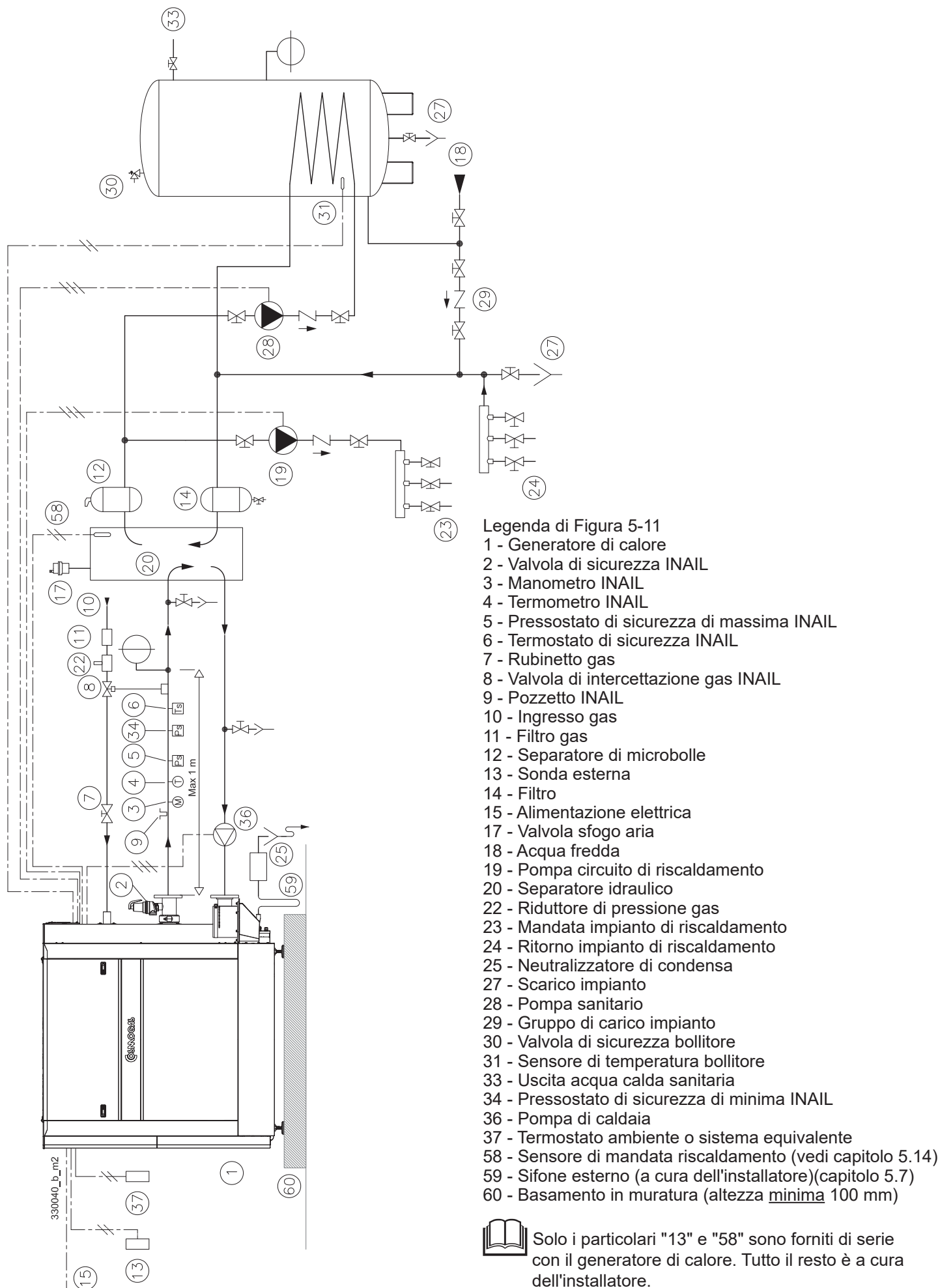
Figura 5-11 - Esempio di collegamento con separatore idraulico e bollitore
