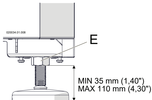
Figura 5-4 Piedini regolabili
