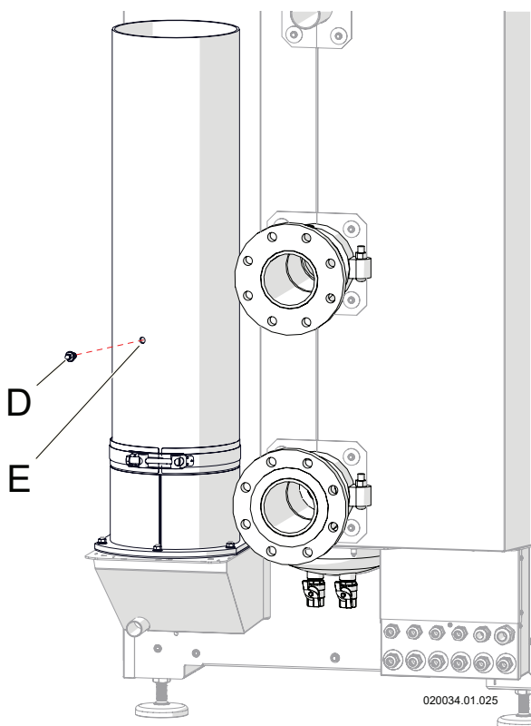
Figura 6-7 - Foro per analisi combustione
