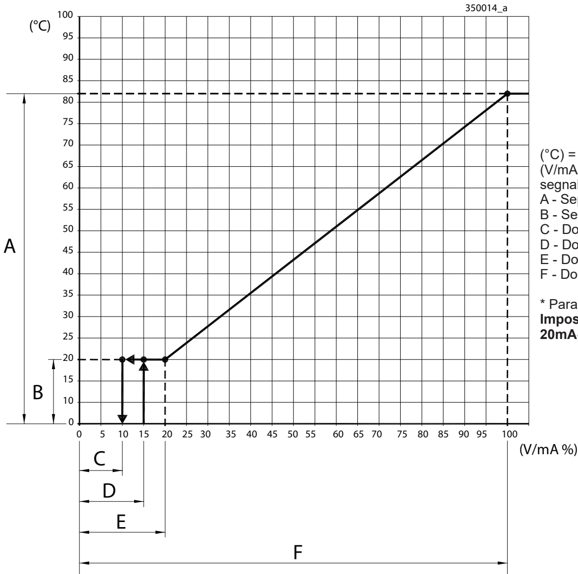
Figura 5-19 - Grafico del controllo della temperatura di setpoint in funzione del segnale 0-10Vdc o 4-20mA
