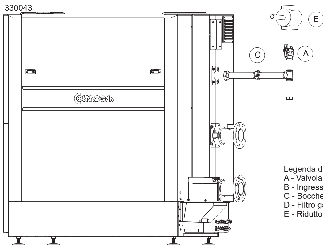
Figura 5-7 - Collegamento gas
