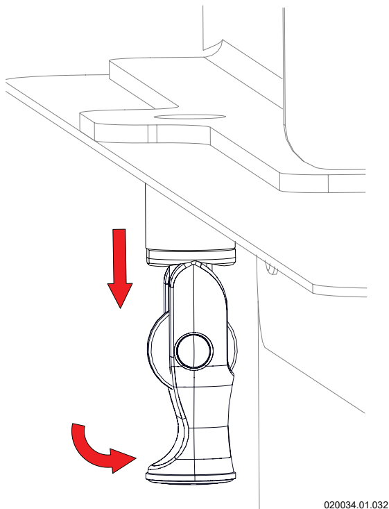
Figura 8-9 - Perno di serraggio
