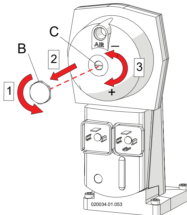
Figura 6-9 - Regolatore CO 2 alla minima potenza
