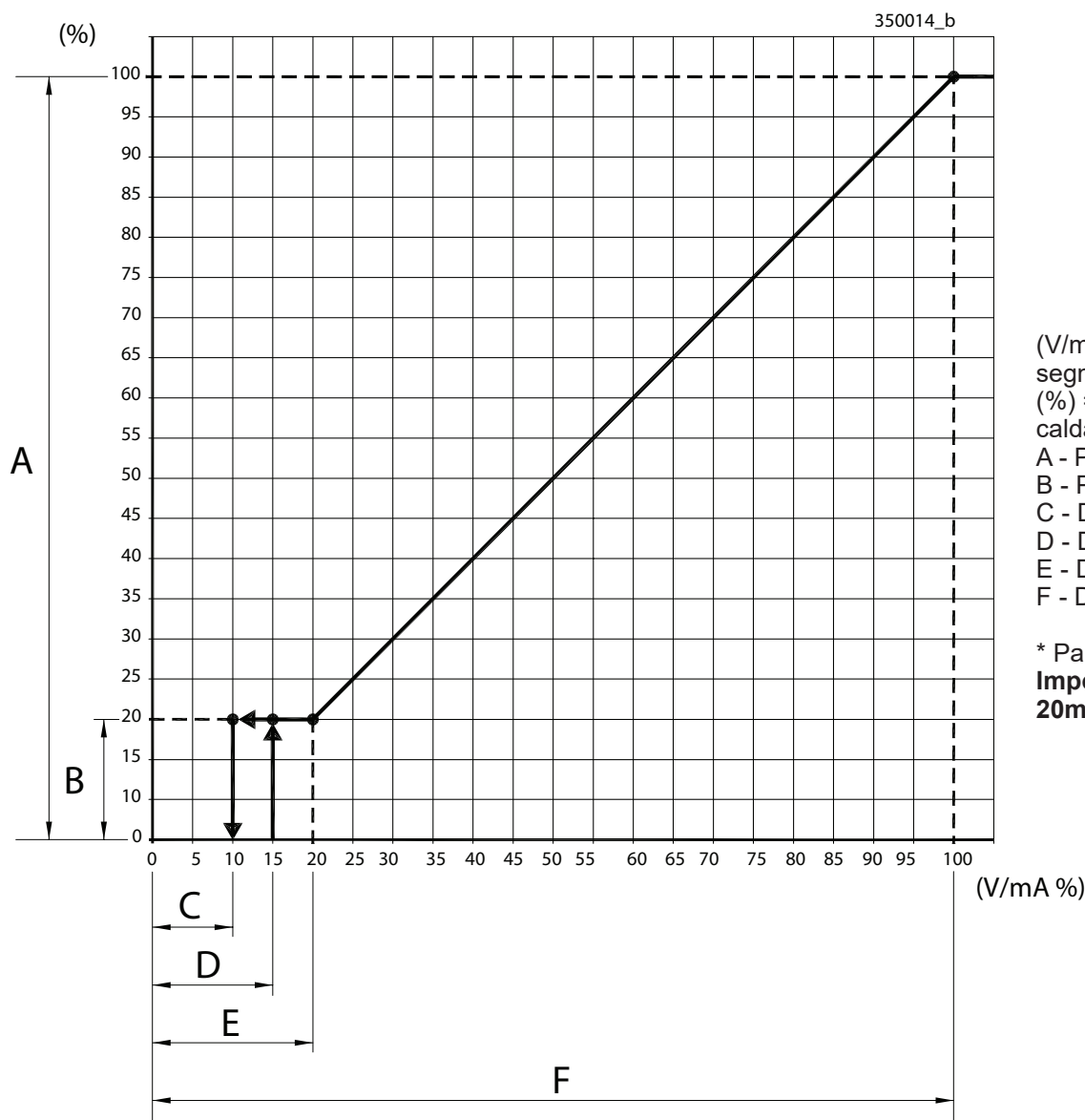
Figura 5-21 - Grafico del controllo della potenza del bruciatore in funzione del segnale 0-10Vdc o 4-20mA COSMOGAS
