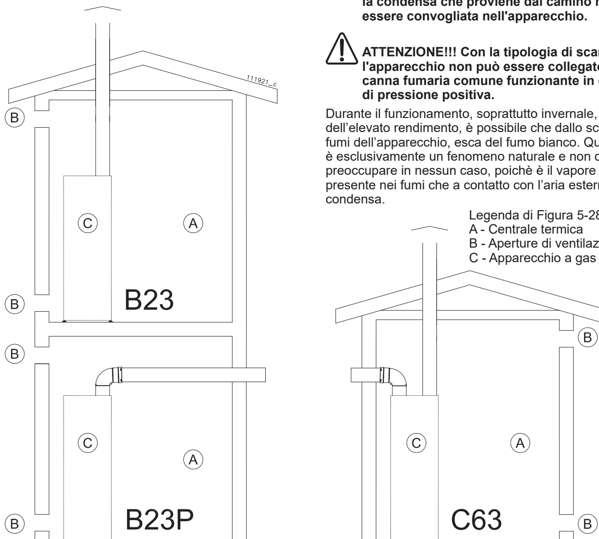
Figura 5-28 - Sistemi di aspirazione/scarico
