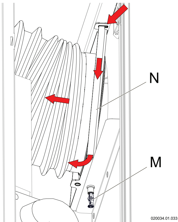
Figura 8-10 - Rimozione tubo aspirazione aria
