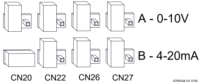
Figura 5-20 - Posizione jumper per segnale esterno 0-10V / 4-20mA (jumper nel quadro elettrico, Figura 3-4)
