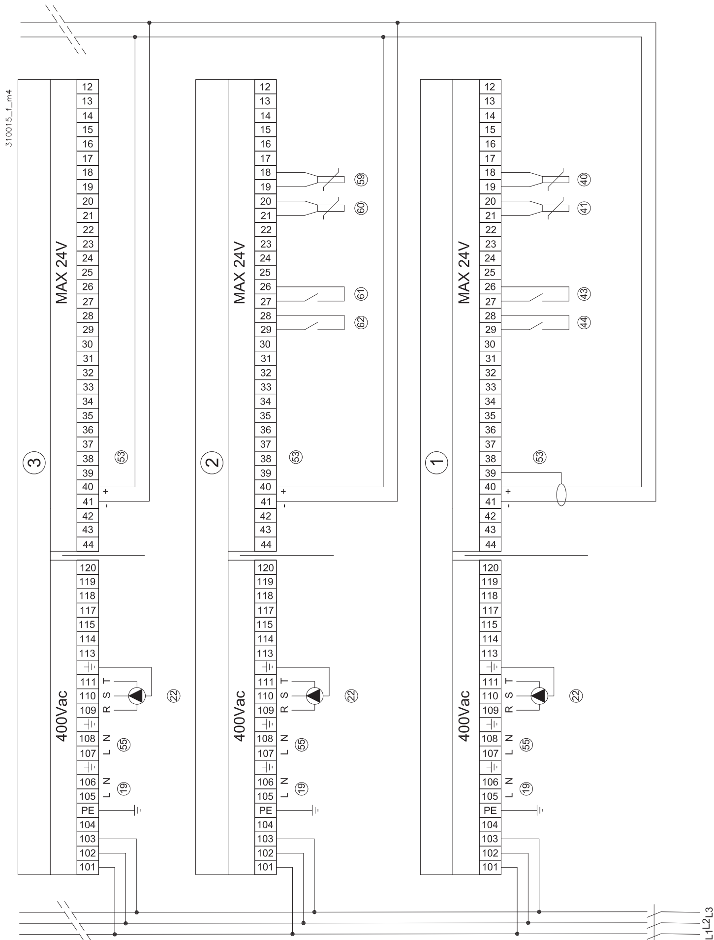
Figura 5-26 - Esempio di collegamento elettrico della cascata con due MASTER (modelli 1100) (per i modelli 495 e 750 occorre aggiungere il cavo di neutro)
