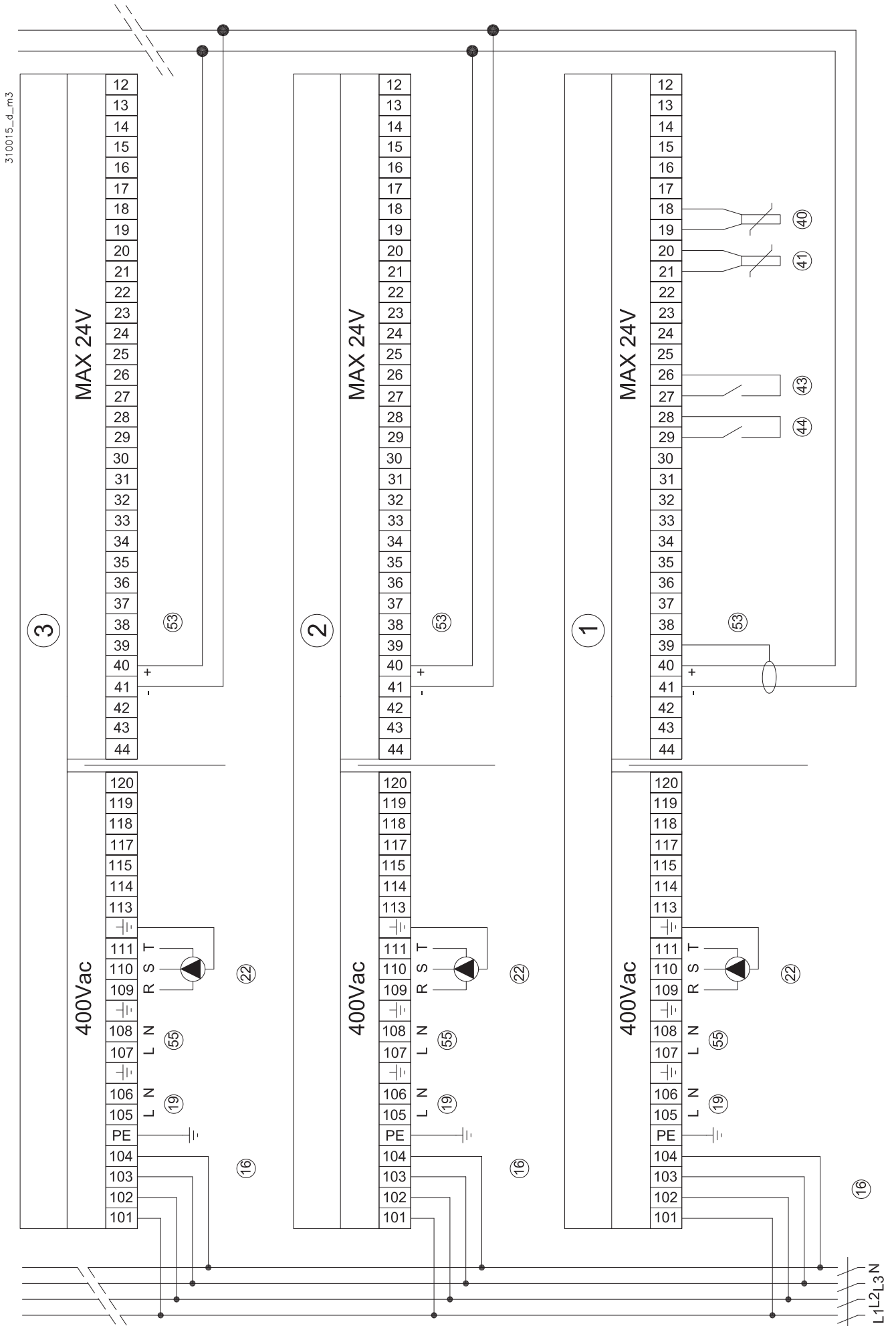
Figura 5-24 - Esempio di collegamento elettrico della cascata con un MASTER (modelli 495 e 750) (per modelli 1100 non è necessario collegare il neutro)
