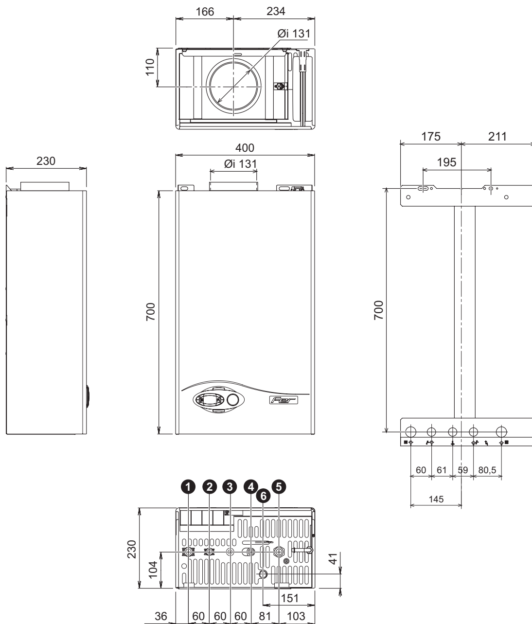
fig. 18 - Dimensioni e attacchi
