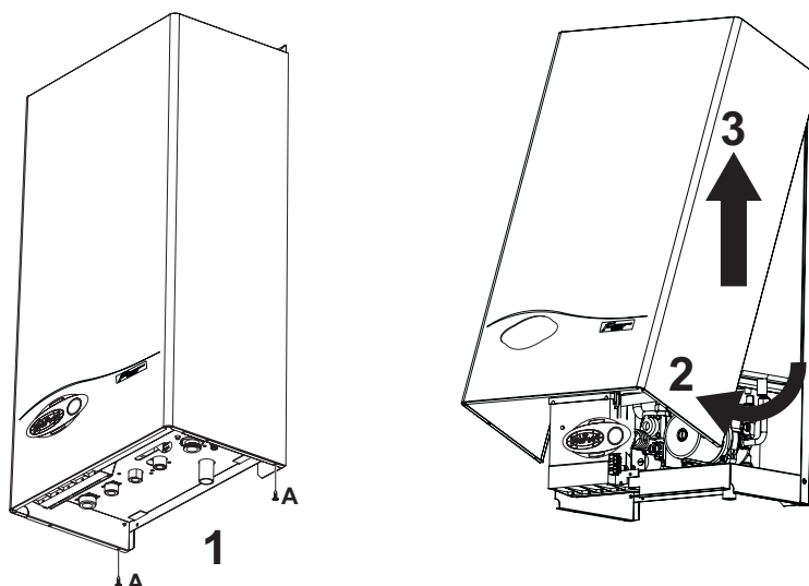
fig. 17 - Apertura mantello
