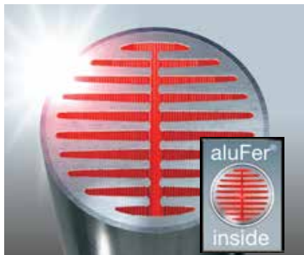
Scambiatore di calore aluFer® per la massima efficienza
