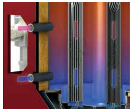
Attacchi di ritorno separati per alta e bassa temperatura per una condensazione ottimale
