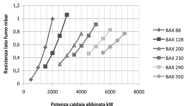
Grafico resistenza lato fumi con temperatura di ritorno tra 30° e 50°C
