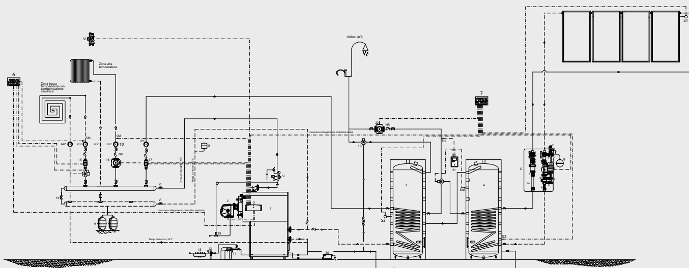
Schema impianto solare per integrazione ACS con 2 bollitori mono serpentino collegati in serie
