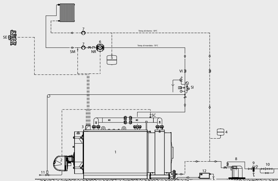
Schema impianto per caldaia GREENOX BT COND : 1 zona diretta, 1 generatore
