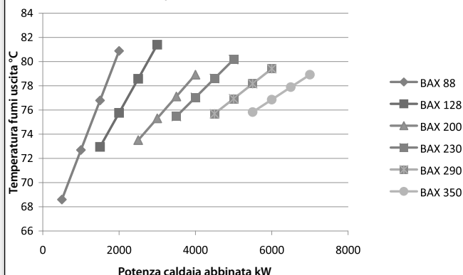
Grafico temperatura uscita fumi con temperatura di ritorno tra 60° e 80°C
