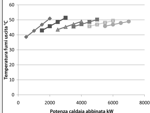
Grafico temperatura uscita fumi con temperatura di ritorno tra 30° e 50°C
