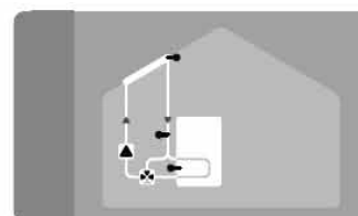
Solare con bypass
