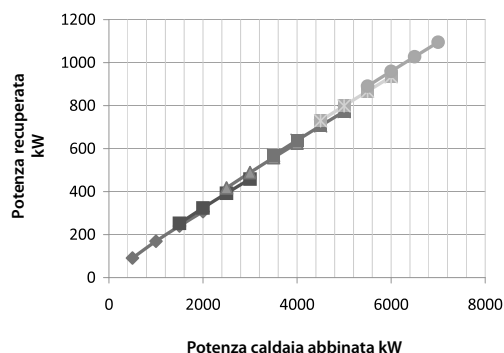
Grafico potenza recuperata con temperatura di ritorno tra 30° e 50°C
