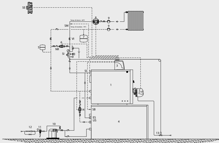
Schema impianto per caldaia modello BLUNOX.e B : 1 zona diretta, 1 generatore, 1 bollitore integrato
