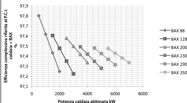
Grafico efficienza complessiva generatore e BAX con temperatura di ritorno tra 60° e 80°C
