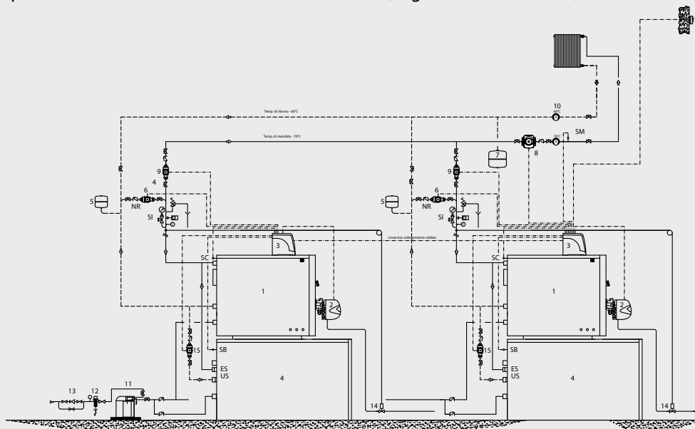
Schema impianto per caldaia modello BLUNOX.e B : 1 zona diretta, 2 generatori in cascata, 2 bollitori integrati
