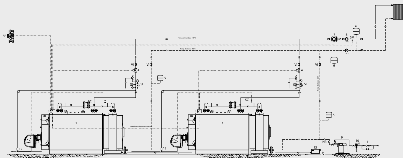
Schema impianto per caldaia GREENOX BT COND : 1 zona diretta, 2 generatori in cascata
