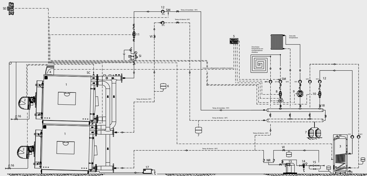
Schema impianto per caldaia STELT DUAL : 1 zona diretta, 1 zona miscelata, 1 generatore, 1 bollitore
