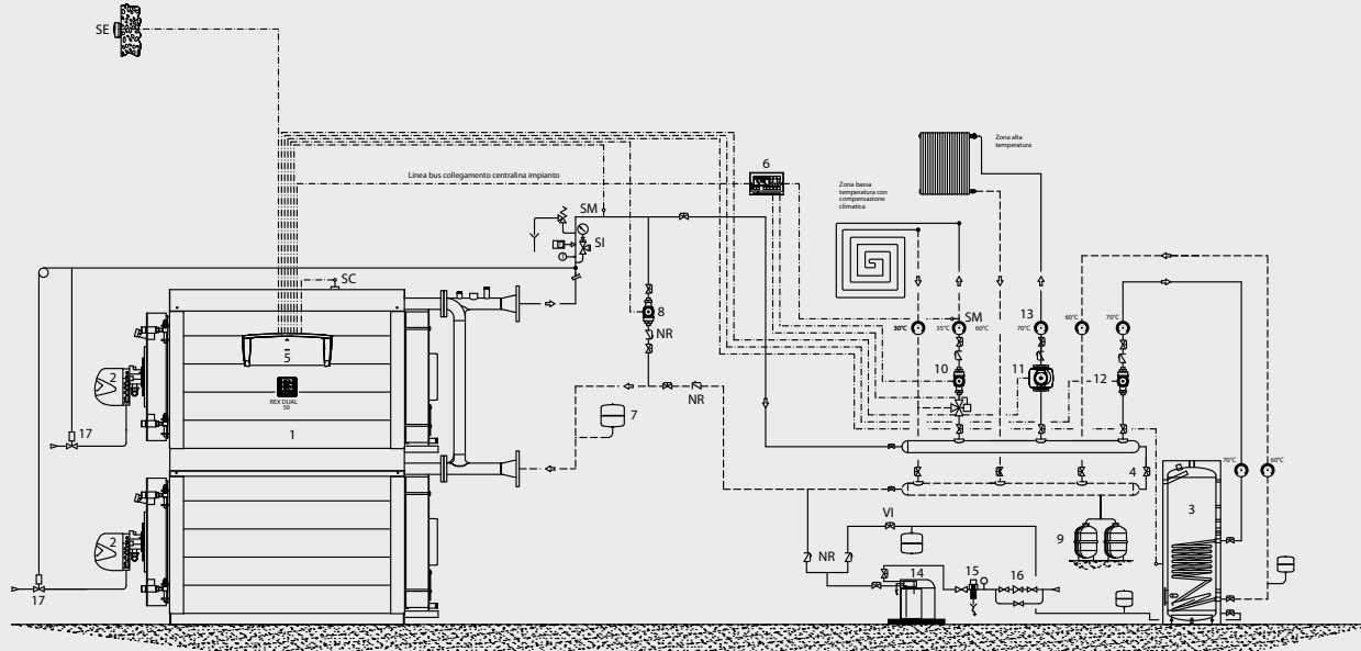
Schema impianto per caldaia modelli REX DUAL e REX DUAL F : 1 zona diretta, 1 zona miscelata, 2 generatori in cascata, 1 bollitore
