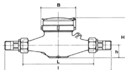
Dimensioni
