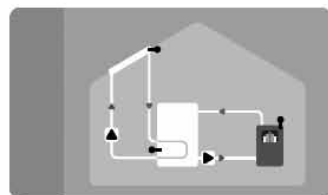
Solare con caldaia a Combustibile solido
