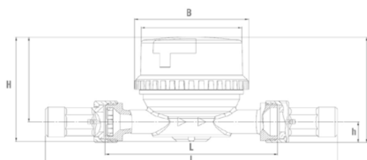
Dimensioni
