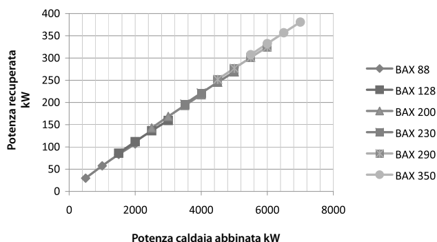
Grafico potenza recuperata con temperatura di ritorno tra 60° e 80°C
