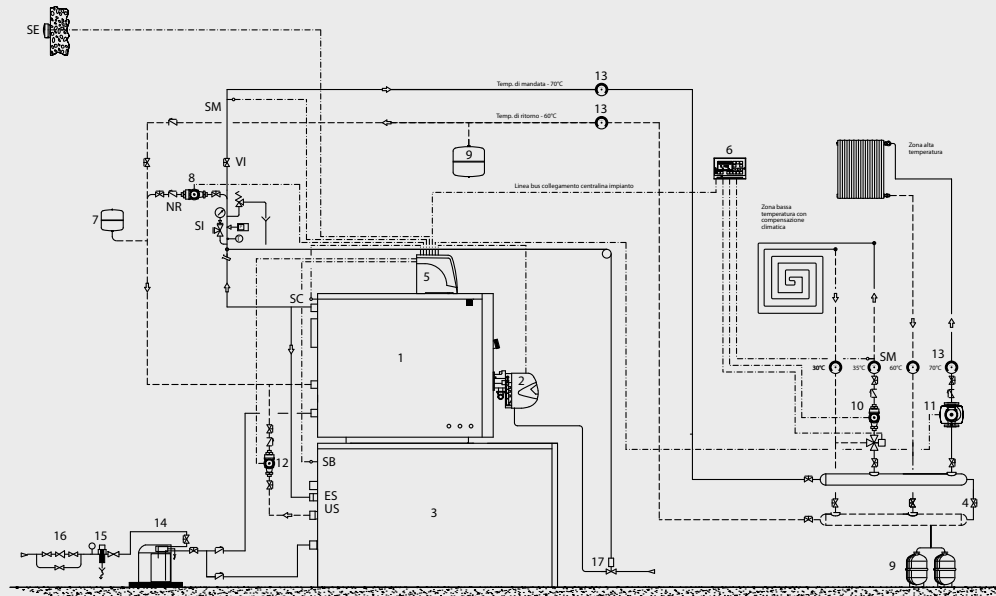
Schema impianto per caldaia modello BLUNOX.e B : 1 zona diretta, 1 zona miscelata, 1 generatore, 1 bollitore integrato
