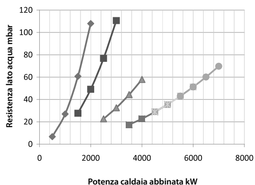
Grafico resistenza lato acqua con temperatura di ritorno tra 30° e 50°C
