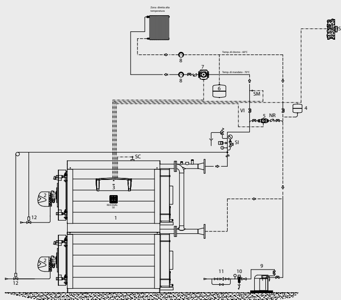
Schema impianto per caldaia modelli REX DUAL e REX DUAL F : 1 zona diretta, 2 generatori in cascata
