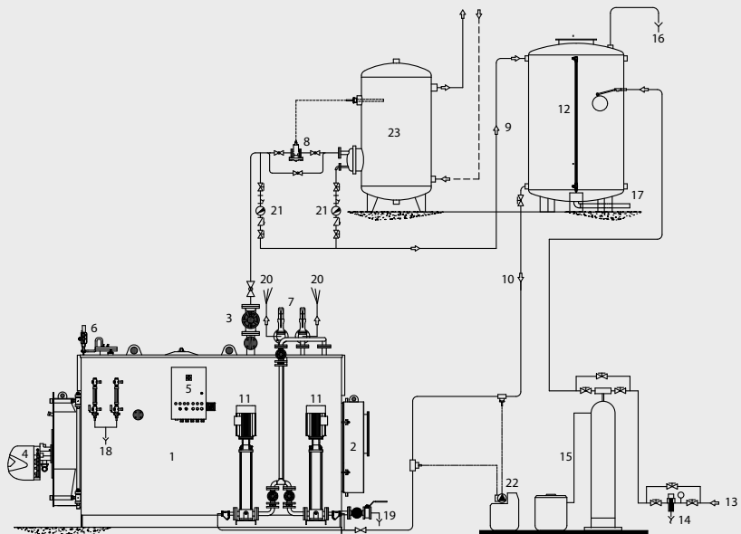
Schema impianto con recupero condensa, per generatori vapore modello SIXEN, BX, FX, GX e GXC
