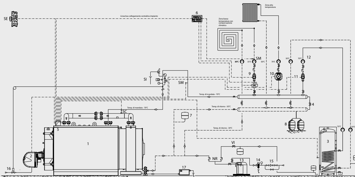
Schema impianto per caldaia GREENOX BT COND : 1 zona diretta, 1 zona miscelata, 1 generatore, 1 bollitore
