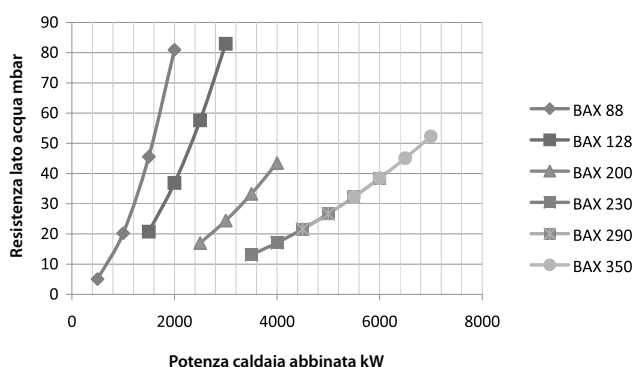
Grafico resistenza lato acqua con temperatura di ritorno tra 60° e 80°C
