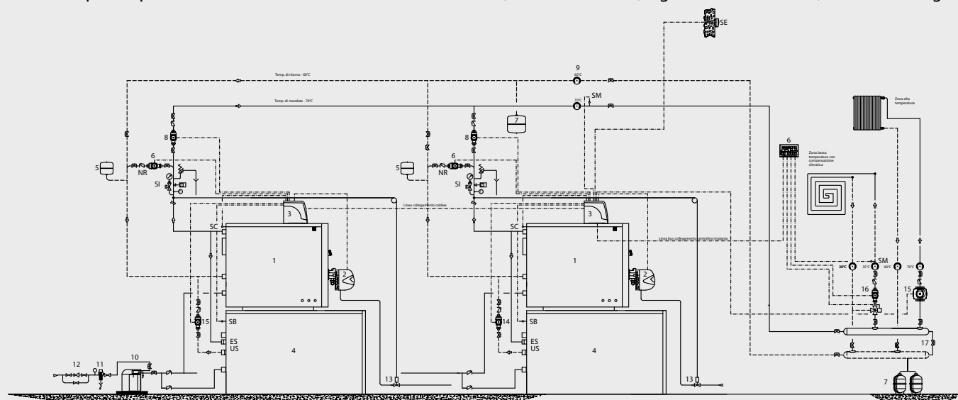
Schema impianto per caldaia modello BLUNOX.e B : 1 zona diretta, 1 zona miscelata, 2 generatori in cascata, 2 bollitori integrati
