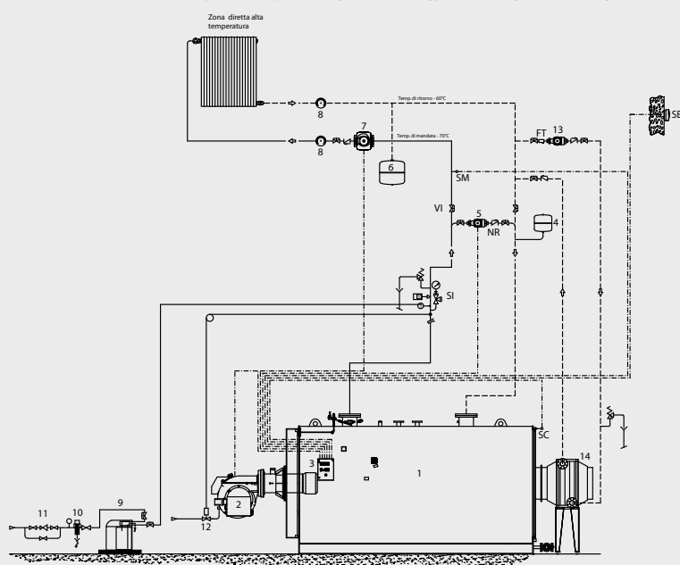
Schema impianto per generatore modello TNX , TNOX, REX (400-600), REX F (400-600) con economizzatore
