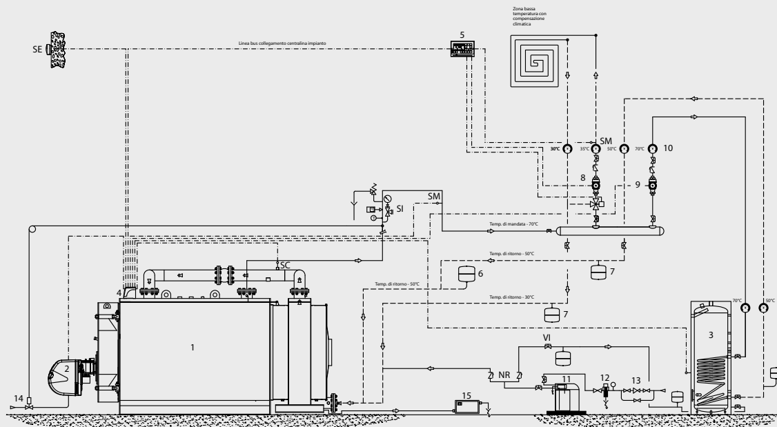
Schema impianto per caldaia GREENOX BT COND : 1 zona miscelata, 1 generatore, 1 bollitore
