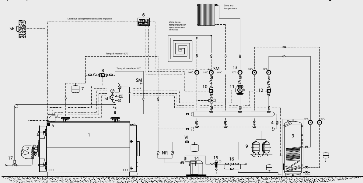
Schema impianto per caldaia modelli REX, BLUNOX.E, REX K, REX F, REX KF e GREENOX.E : 1 zona diretta, 1 zona miscelata, 1 generatore, 1 bollitore
