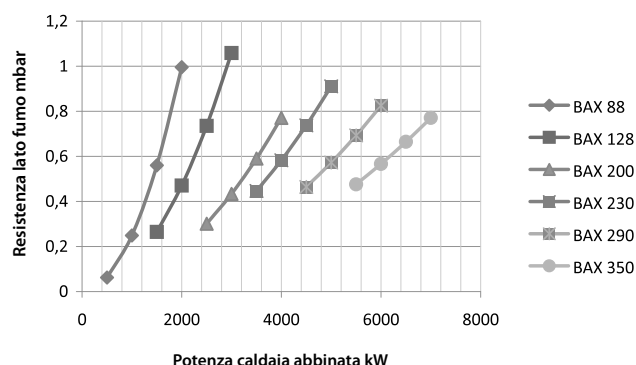
Grafico resistenza lato fumi con temperatura di ritorno tra 60° e 80°C
