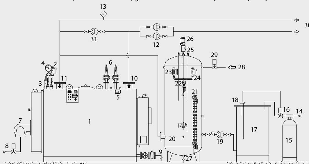
Schema impianto a circuito chiuso per riscaldamento, generatori modello ASX, ASGX EN, TNX, TNOX e TNOX.e
