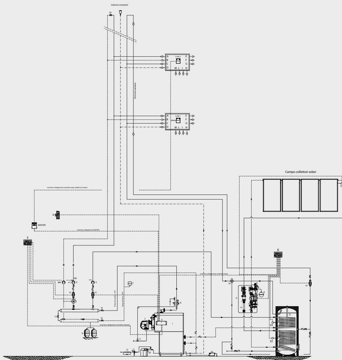
Schema impianto centralizzato ed integrazione solare termico per satelliti modello NEREIX PAVIMENTO
