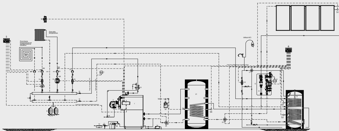
Schema impianto solare per integrazione ACS e riscaldamento, con bollitore doppio serpentino e accumulo puffer
