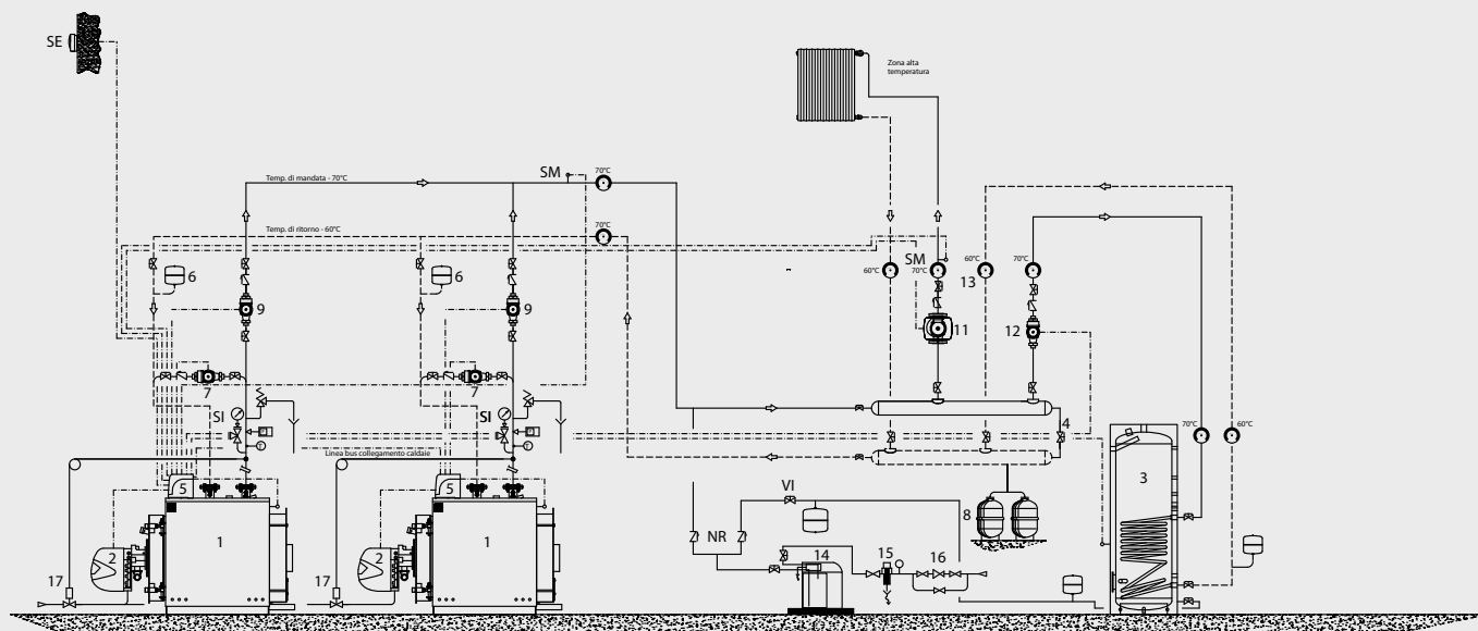
Schema impianto per caldaia modello REX, BLUNOX.E, REX K, REX F, REX KF e GREENOX.E : 1 zona diretta, 2 generatori in cascata, 1 bollitore
