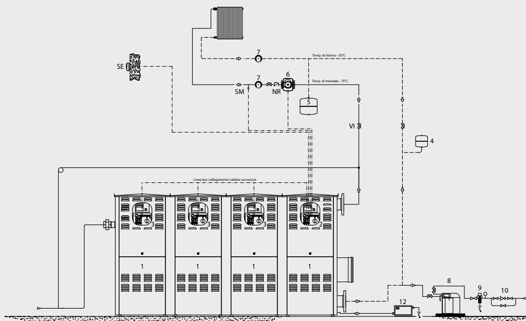
Schema impianto per gruppo termico modulare WALL-WALL M : 1 zona diretta, 1 gruppo termico
