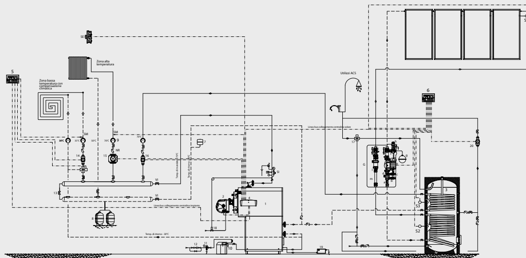
Schema impianto solare per integrazione ACS con bollitore doppio serpentino
