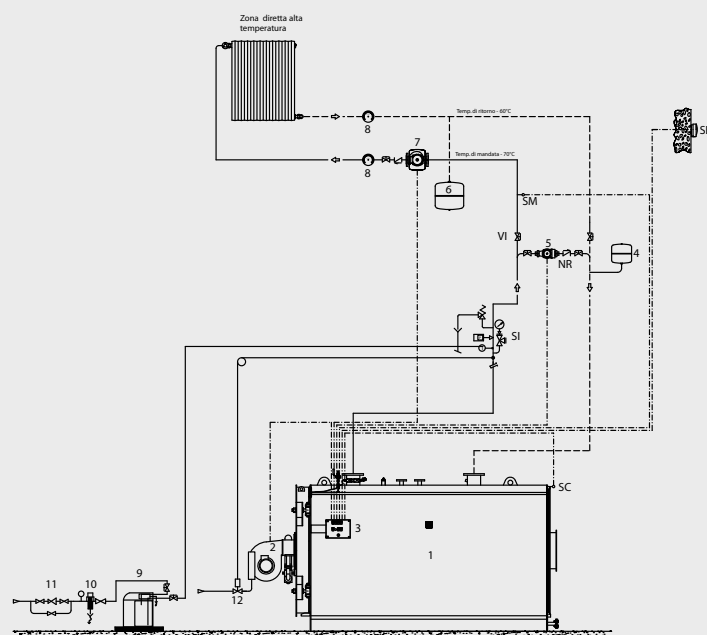
Schema impianto per generatore modello TNX , TNOX, REX (400-600), REX F (400-600)
