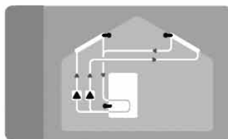
Solare con 2 collettori e 2 pompe
