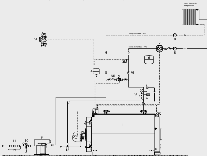
Schema impianto per caldaia modelli REX, BLUNOX.E, REX K, REX F, REX KF e GREENOX.E : 1 zona diretta, 1 generatore
