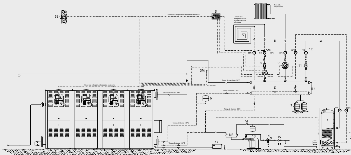
Schema impianto per gruppo termico modulare WALL-WALL M : 1 zona miscelata, 1 zona diretta, 1 gruppo termico, 1 bollitore
