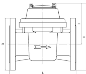
Dimensioni
