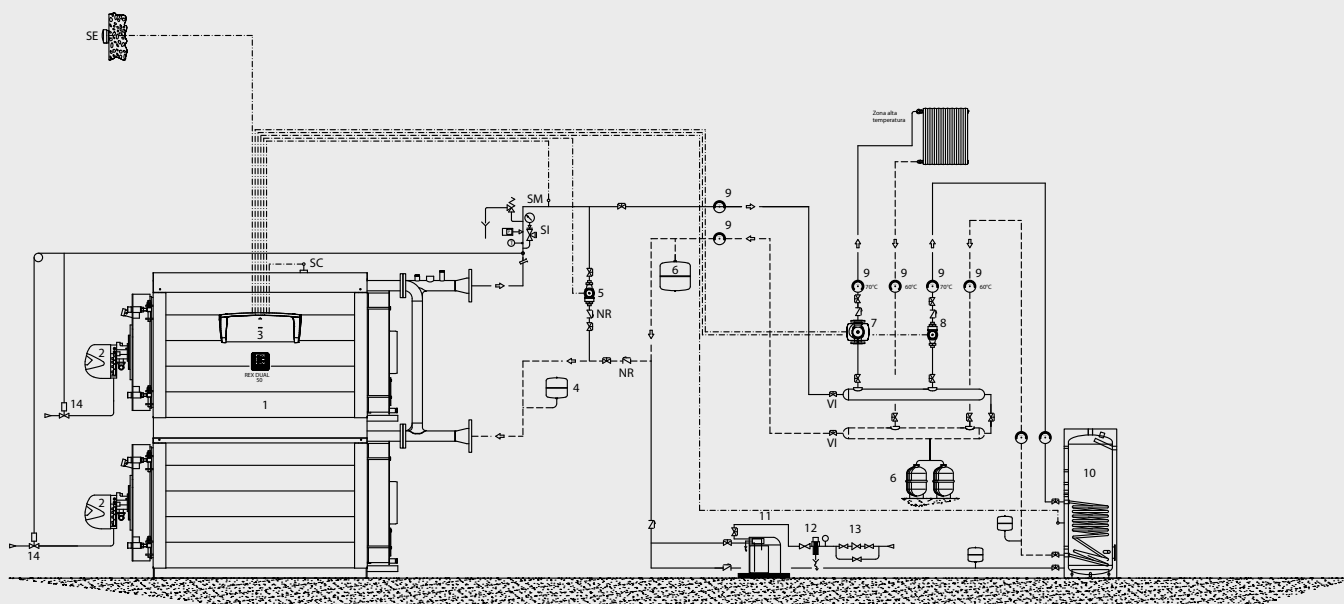
Schema impianto per caldaia modello REX DUAL e REX DUAL F : 1 zona diretta, 2 generatori in cascata, 1 bollitore
