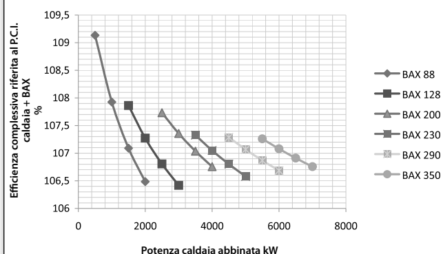
Grafico efficienza complessiva generatore e BAX con temperatura di ritorno tra 30° e 50°C
