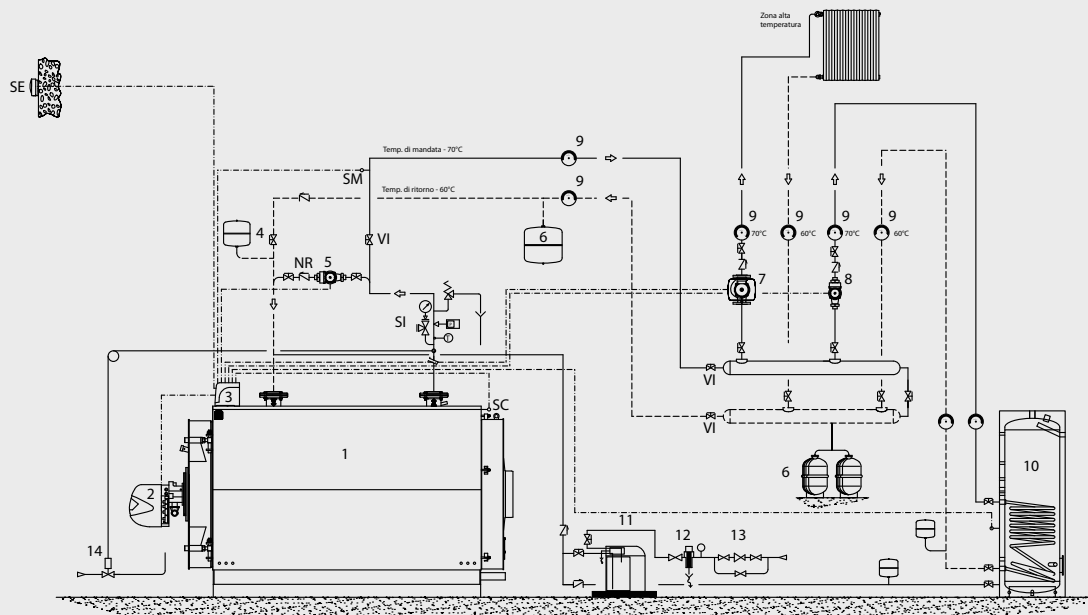
Schema impianto per caldaia modello REX, BLUNOX.E, REX K, REX F, REX KF e GREENOX.E : 1 zona diretta, 1 generatore, 1 bollitore
