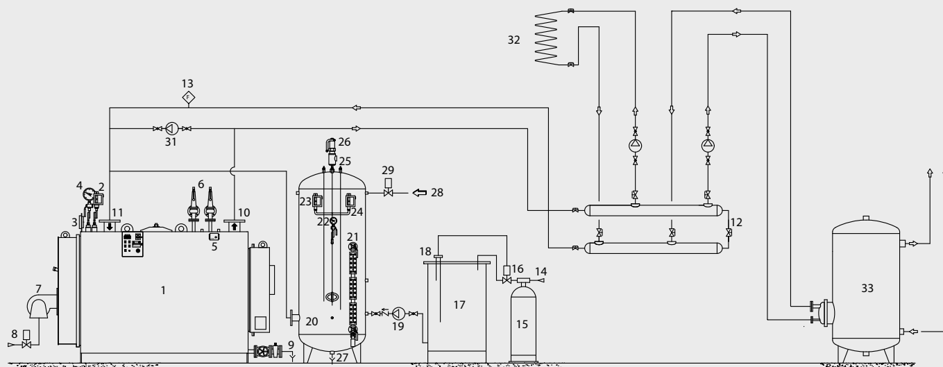
Schema impianto a circuito chiuso per riscaldamento e produzione di ACS, generatori modello ASX, ASGX EN, TNX, TNOX e TNOX.e
