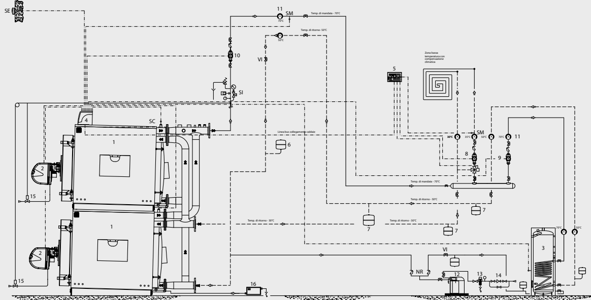
Schema impianto per caldaia STELT DUAL : 1 zona miscelata, 1 generatore, 1 bollitore
