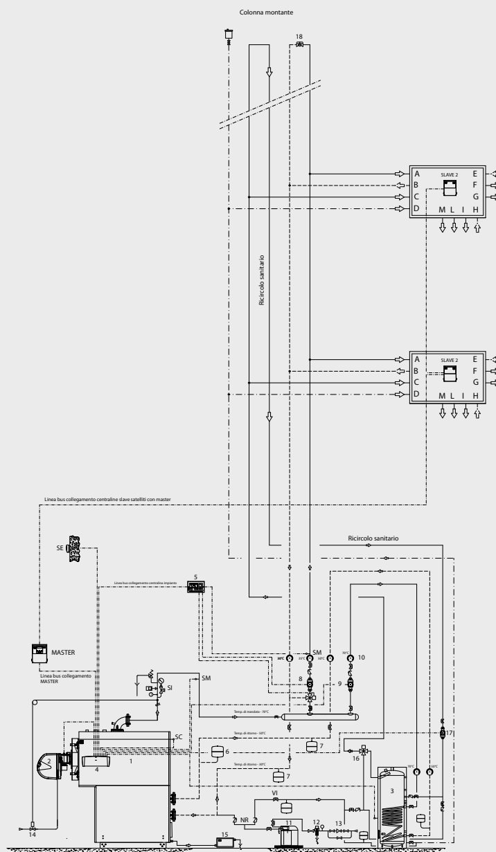
Schema impianto centralizzato, per satelliti modello NEREIX PAVIMENTO
