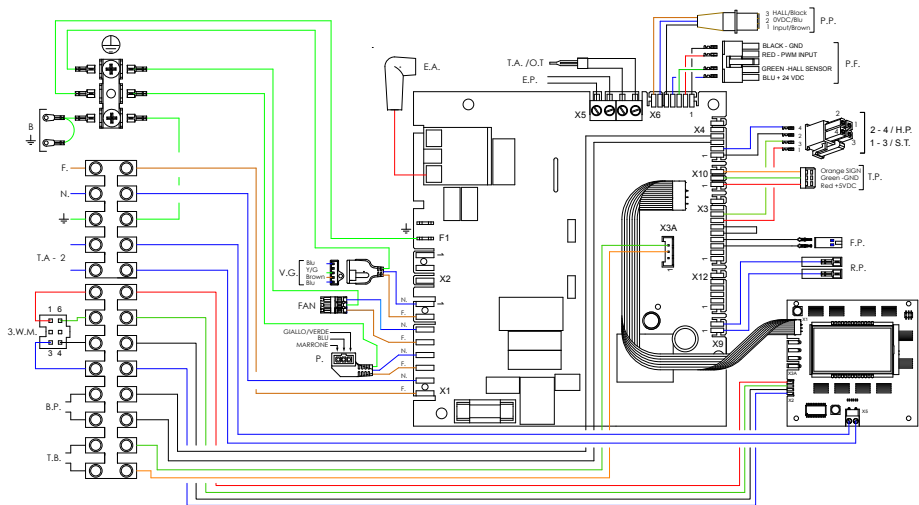
Lista connessioni GIMAX PLUS MR/MN
