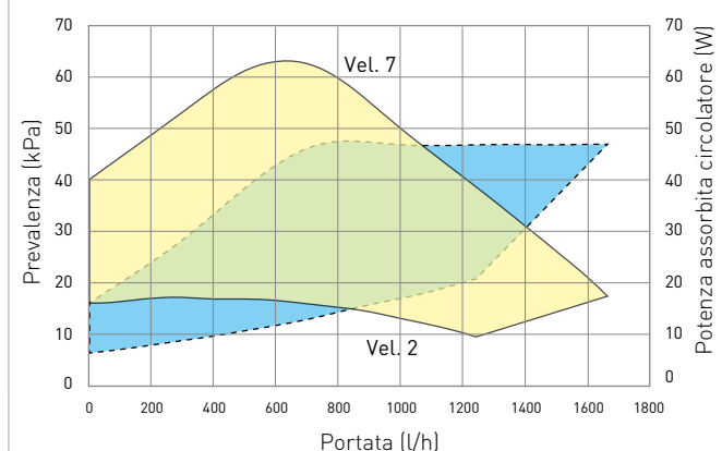
Grafico zona miscelata
