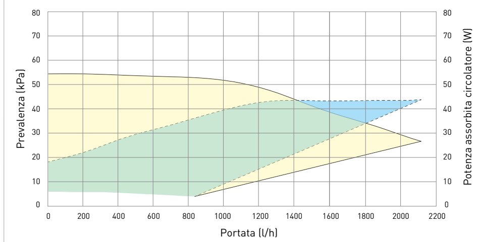
Grafico portata e prevalenza
