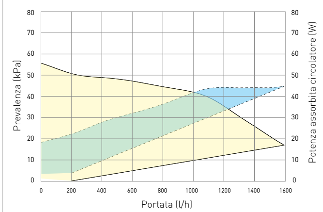
Grafico portata e prevalenza ZONA DIRETTA
