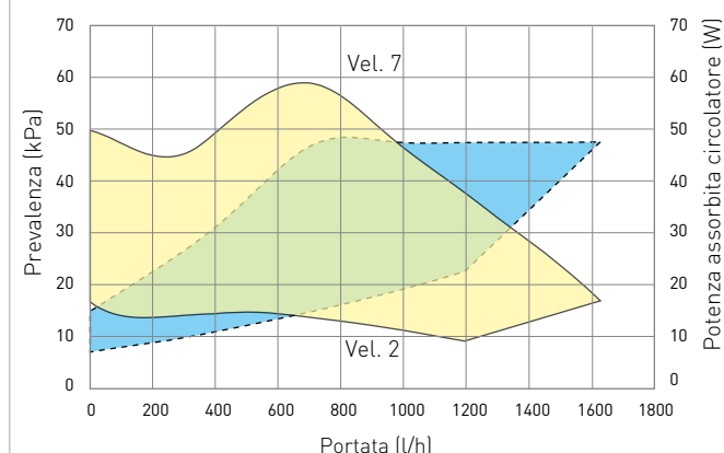
Grafico zona diretta
