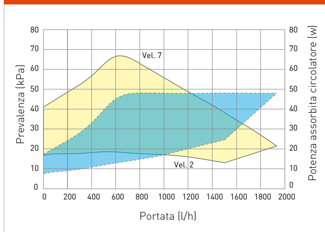
Grafico portata e prevalenza
