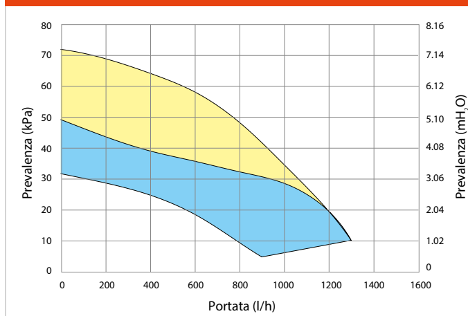
Grafico portata e prevalenza VICTRIX SUPERIOR 26 ErP
