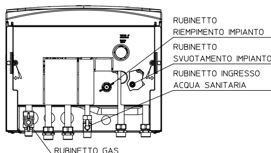
VISTA INFERIORE
