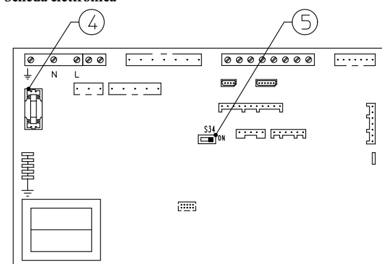
Scheda elettronica
