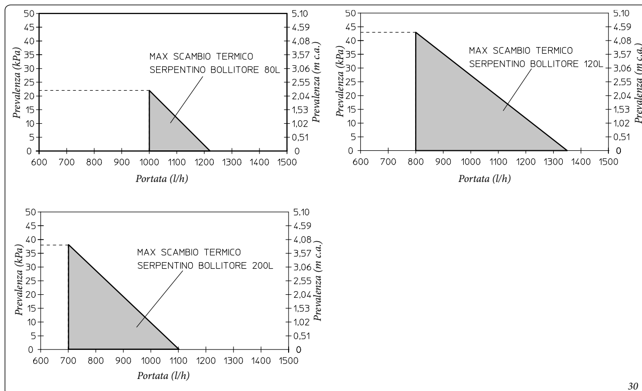
Prevalenza disponibile all'Unità Bollitore.
