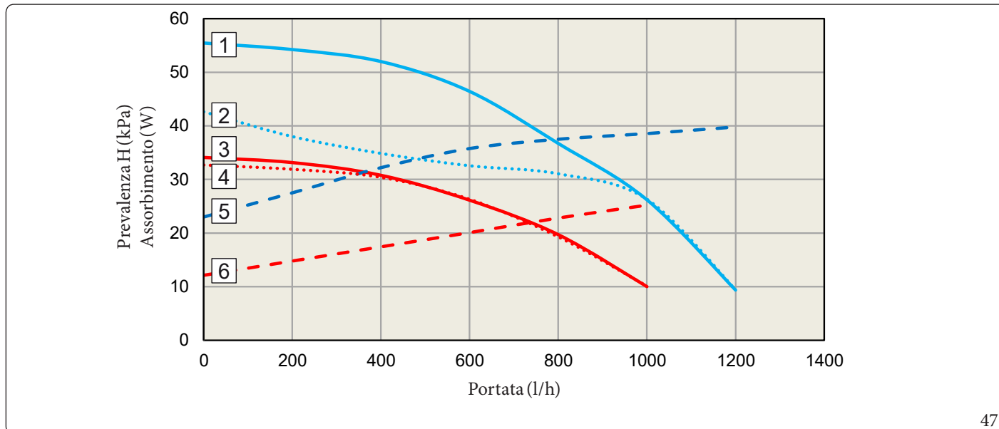
Grafico Portata - Prevalenza - Assorbimento Victrix Zeus 25
