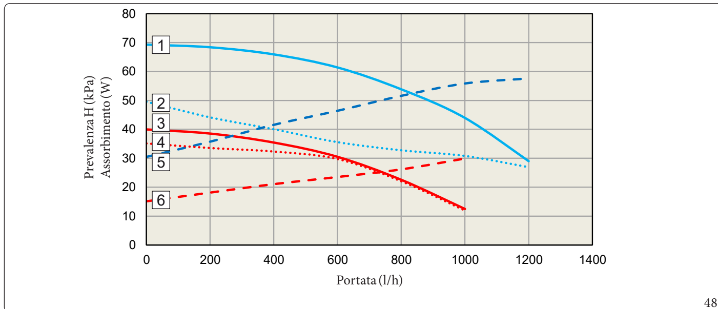
Grafico Portata - Prevalenza - Assorbimento Victrix Zeus 32
