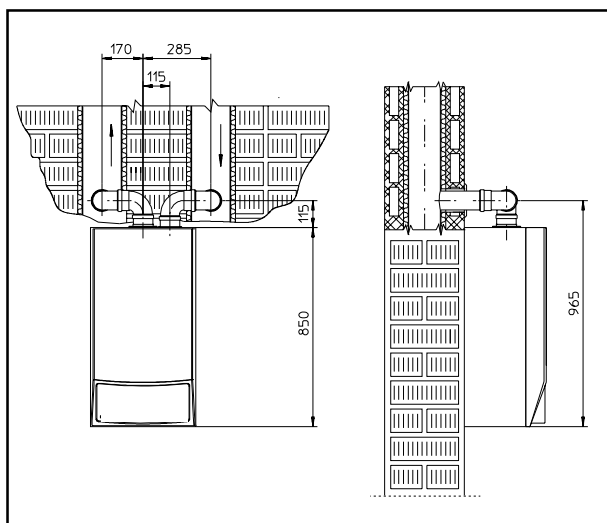
Massime lunghezze utilizzabili (compreso il terminale di aspirazione grigliato e le due curve a 90°)
