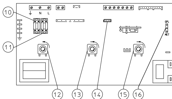
Scheda elettronica
