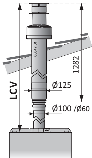
Esempio di sistema coassiale verticale (C 32 )
