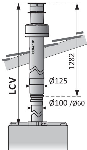
Esempio di sistema coassiale verticale (C 32 )
