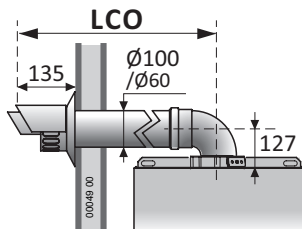
Esempio di sistema coassiale orizzontale (C 12 )
