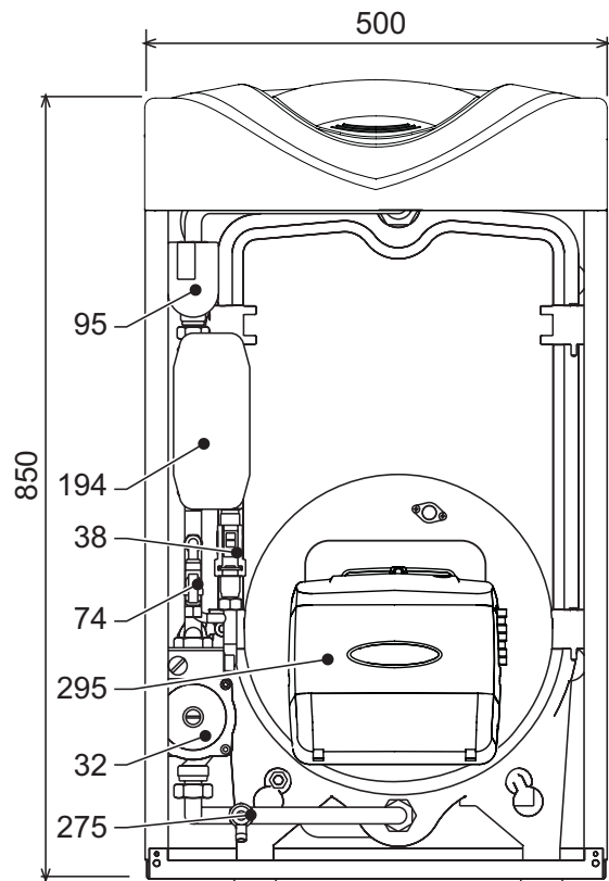
fig. 18 - vista anteriore
