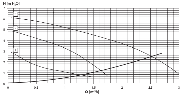
fig. 21 - Perdite di carico
