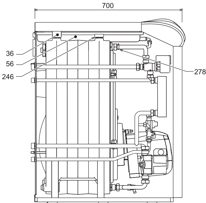
fig. 19 - vista laterale
