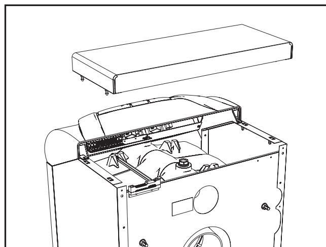
fig. 16 - Accesso alla morsettiera
