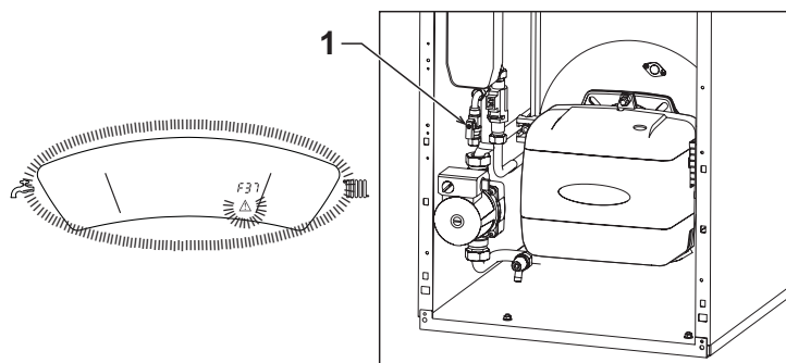
fig. 15 - Anomalia pressione impianto insufficiente - Rubinetto di caricamento
