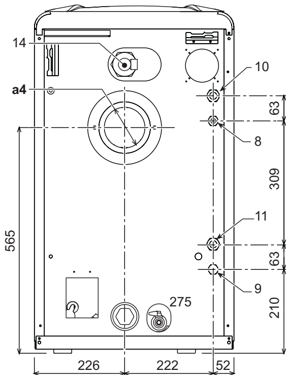
fig. 20 - Vista posteriore
