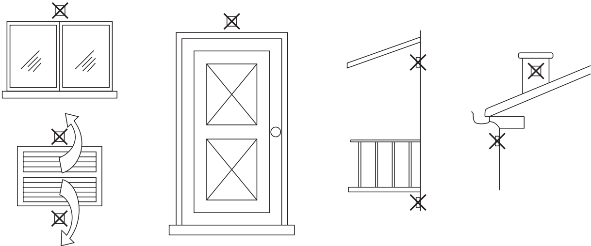
fig. 17 - Posizionamento sconsigliato sonda esterna
