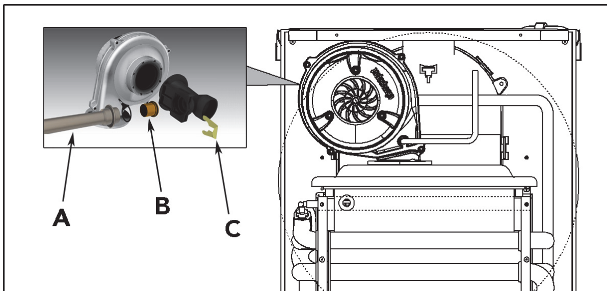
fig. 26 - Trasformazione gas
