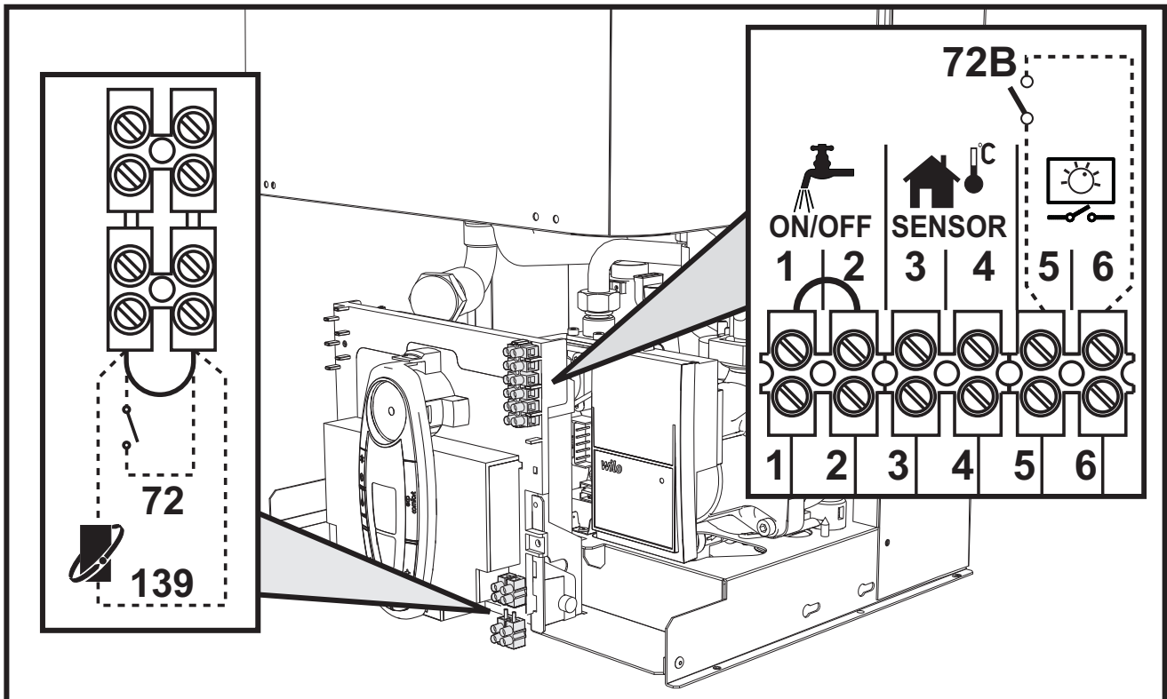
fig. 18 - Accesso alla morsetteria
