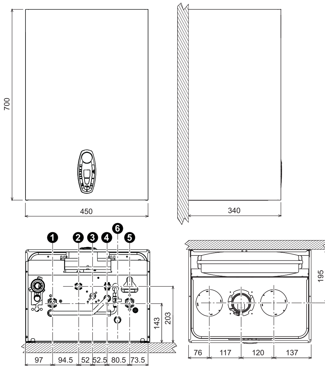
fig. 30 - Dimensioni e attacchi
