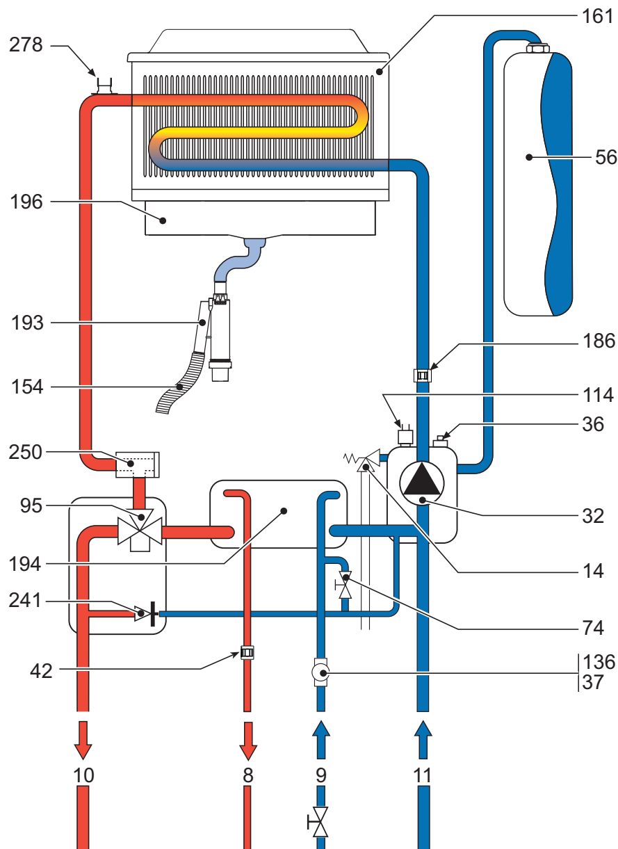
fig. 32 - Circuito idraulico
