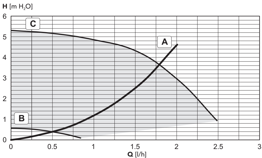
fig. 33 - Perdita di carico/prevalenza circolatori
