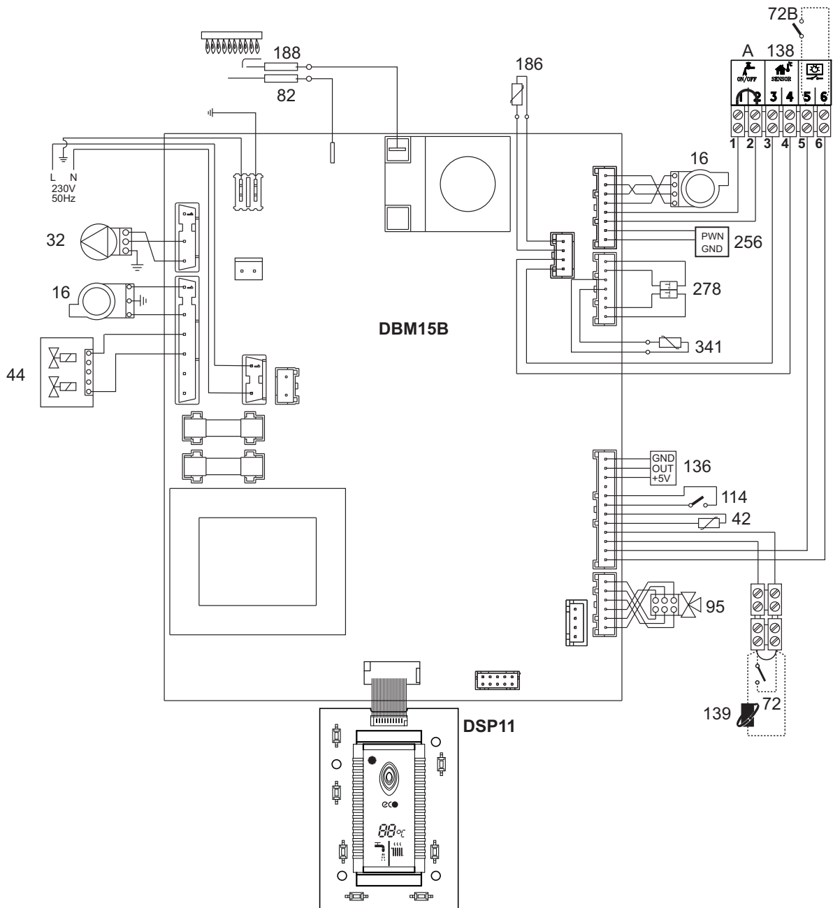
fig. 34 - Schema elettrico
