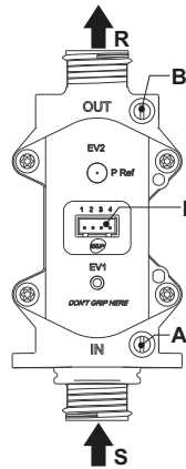
рис. 10 - Газовый клапан
