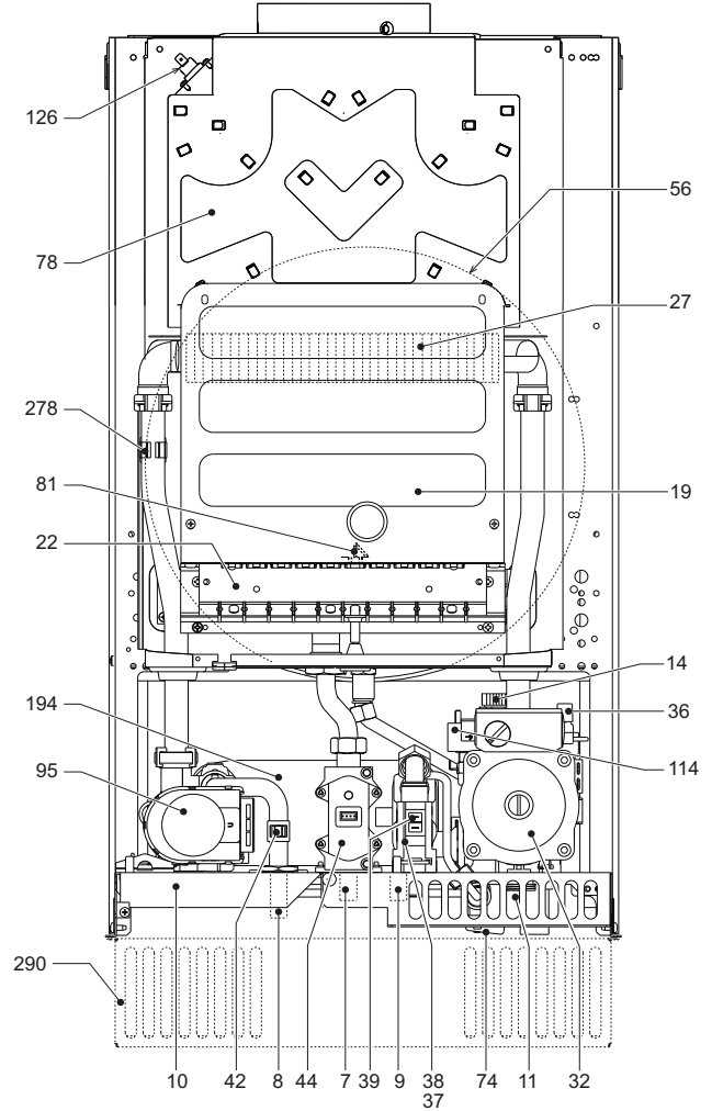
рис. 13 - Общий вид CLIZIA D 24 A
