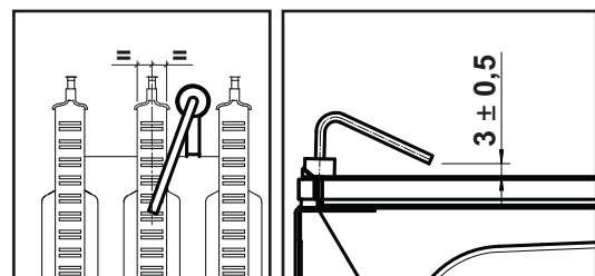
fig. 12 - Posizionamento elettrodo
