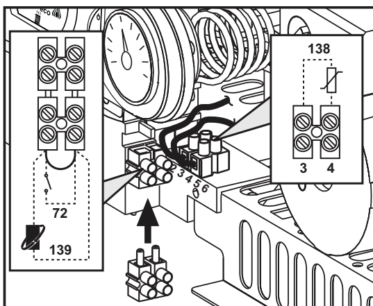
fig. 8 - Accesso alla morsettiera
