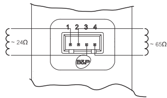
рис. 11 - Электрический разъем для подключения газового клапана
