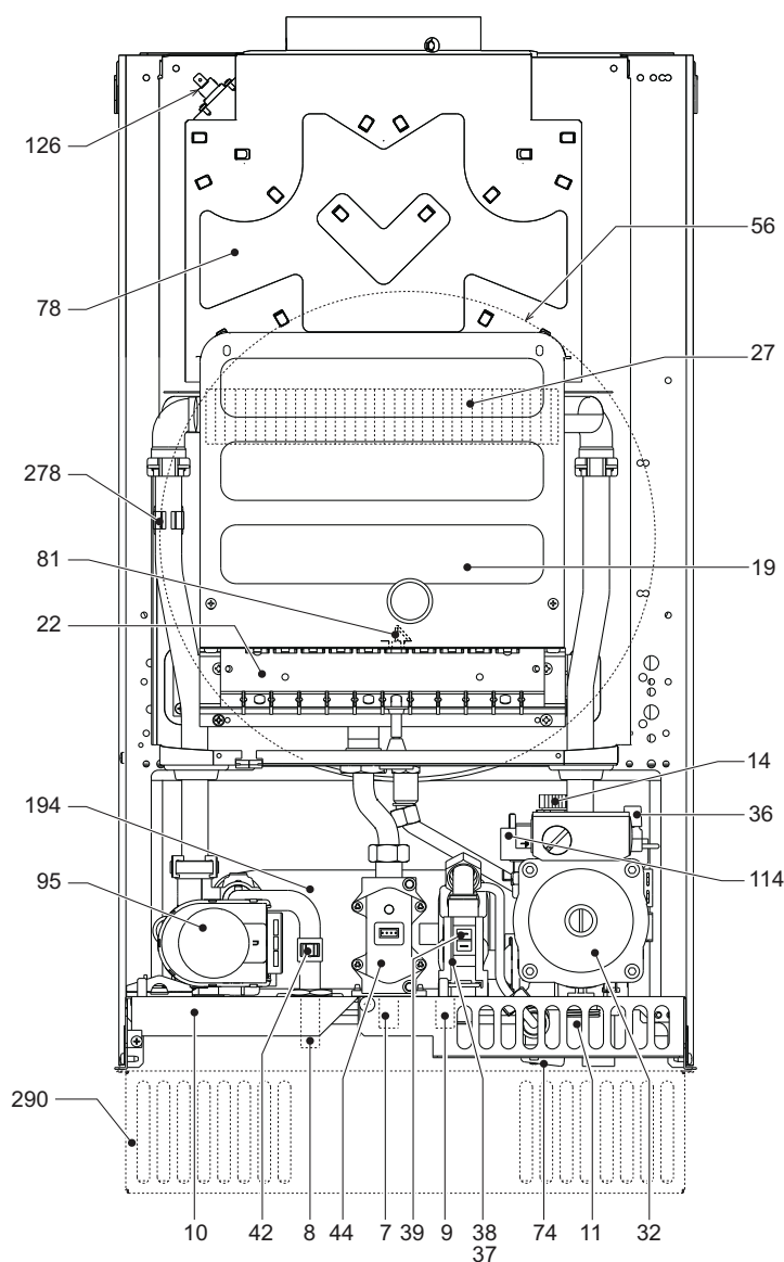
fig. 13 - Vista generale CLIZIA D 24 A
