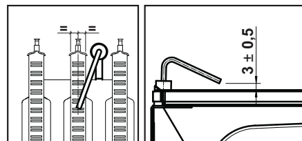
рис. 12 - Положение электрода
