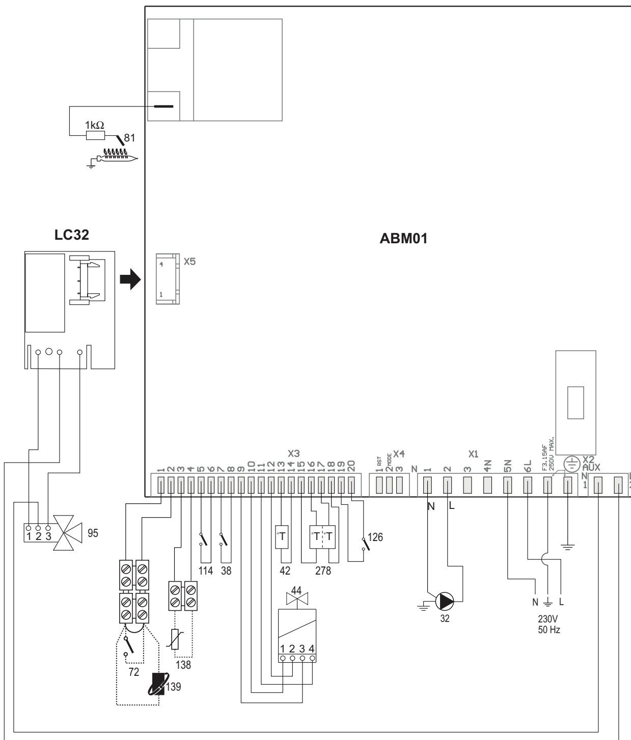
fig. 16 - Circuito eléctrico
