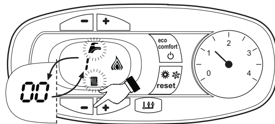
fig. 9 - Modo TEST (potencia de calefacción = 100 %)
