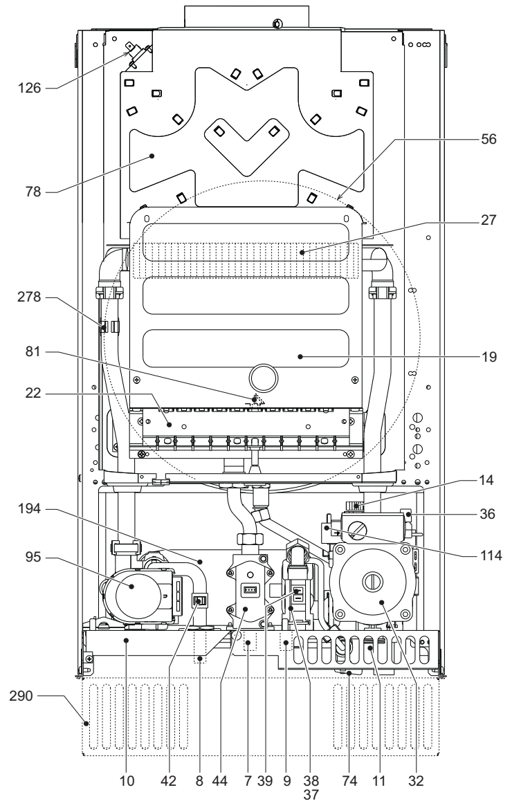
fig. 13 - Vista general CLIZIA D 24 A
