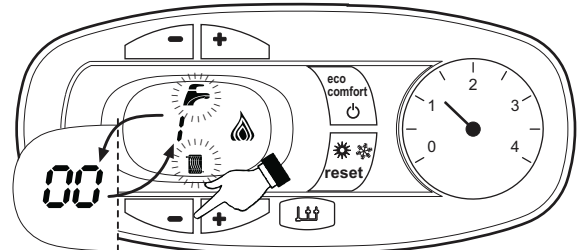
fig. 9 - Modalità TEST (potenza riscaldamento = 100%)
