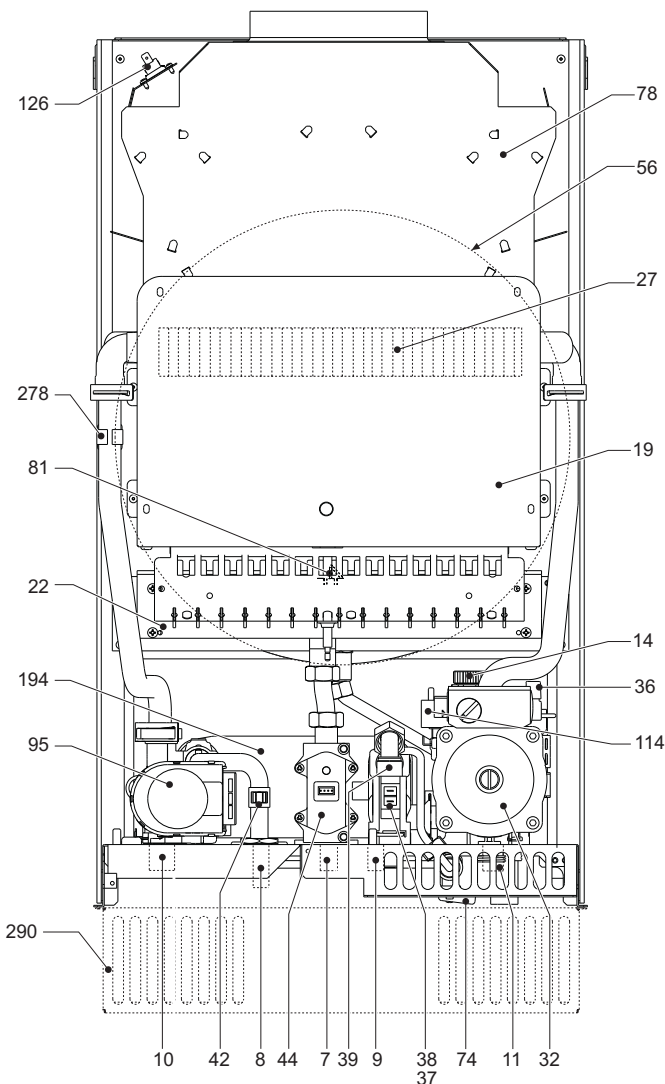
fig. 13 - Vista generale CLIZIA D 32 A
