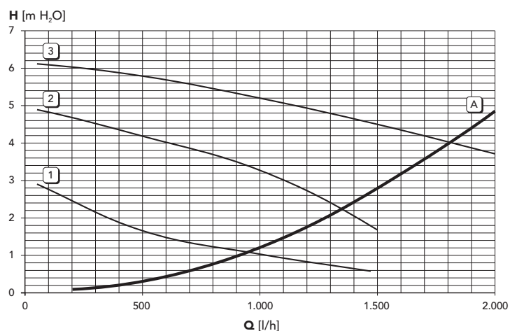
Потери напора / напор циркуляционных насосов CLIZIA D 32 A
