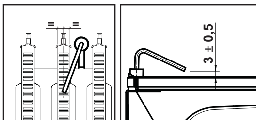
fig. 12 - Posizionamento elettrodo
