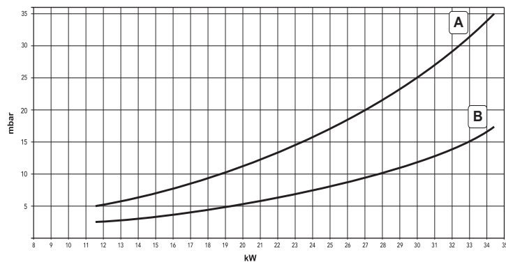
Потери напора / напор циркуляционных насосов CLIZIA D 32 A
