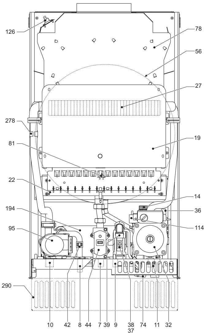
fig. 13 - Vista general CLIZIA D 32 A
