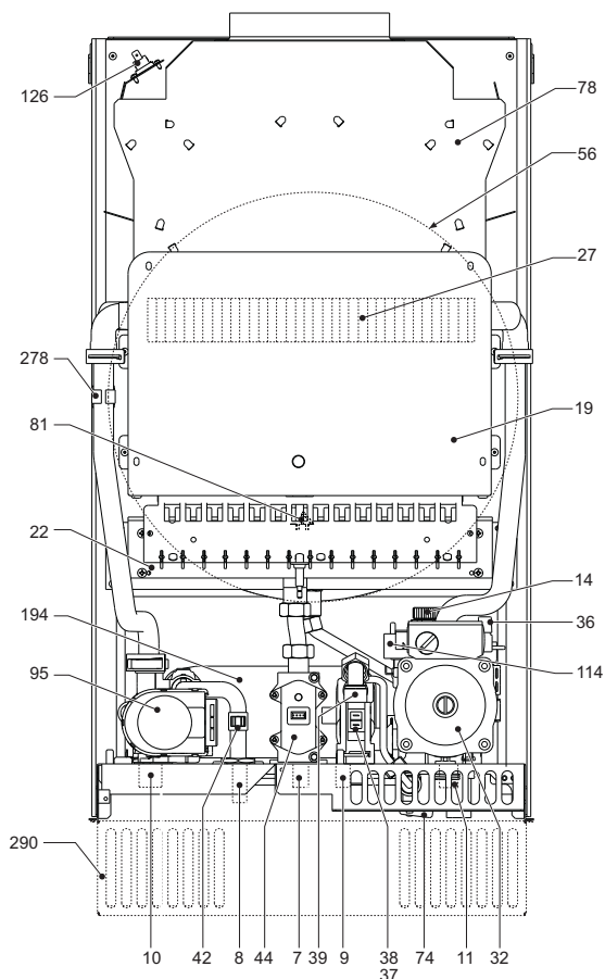
рис. 13 - Общий вид CLIZIA D 32 A
