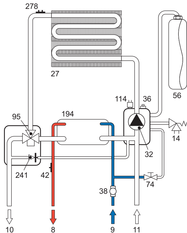
рис. 15 - Контур ГВС
