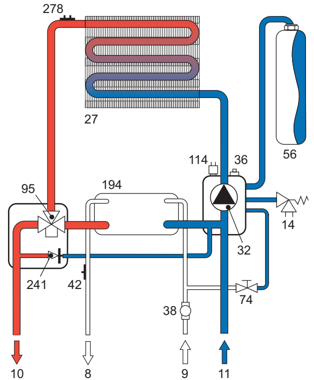
fig. 14 - Circuito de calefacción
