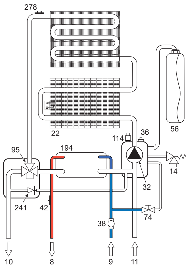
fig. 23 - Circuito sanitario
