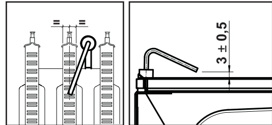
fig. 20 - Posizionamento elettrodo
