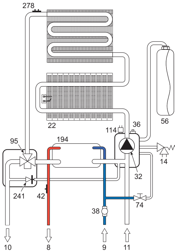
рис. 23 - Контур ГВС
