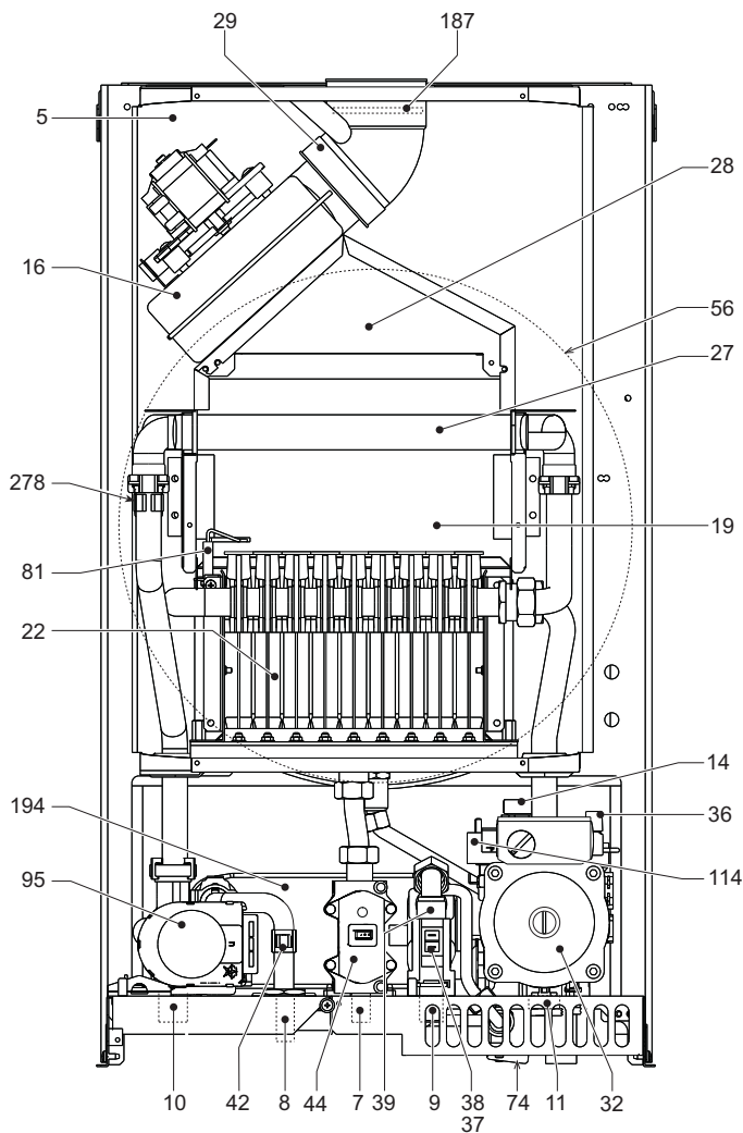
рис. 21 - Общий вид
