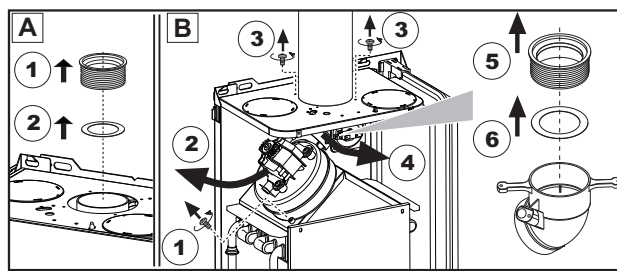
A Замена диафрагмы перед установкой котла B Замена диафрагмы после установки котла и соответствующих дымовых труб
