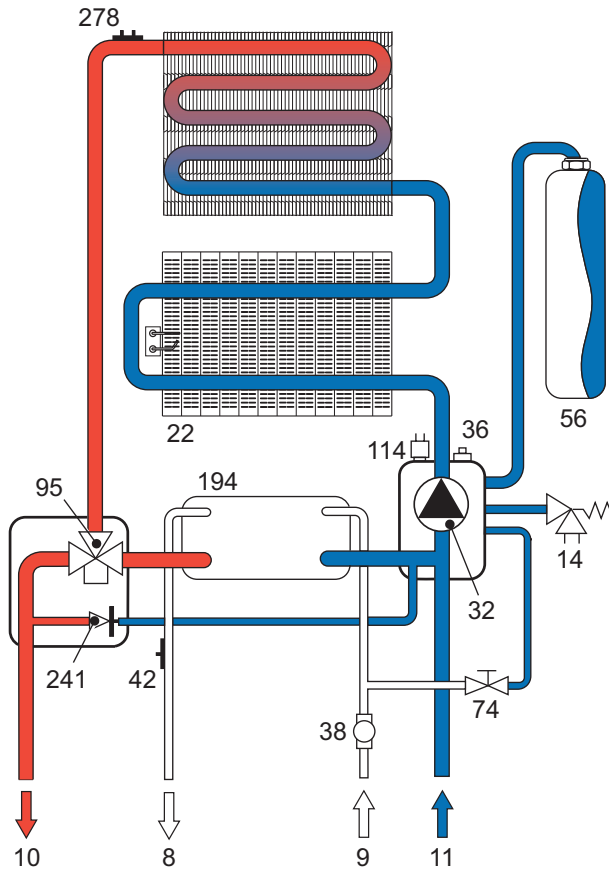
рис. 22 - Отопительный контур
