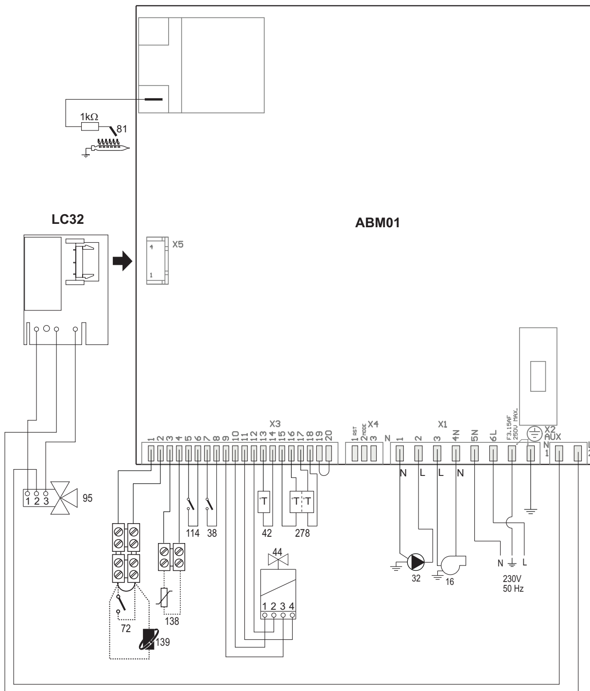
рис. 24 - Электрическая цепь
