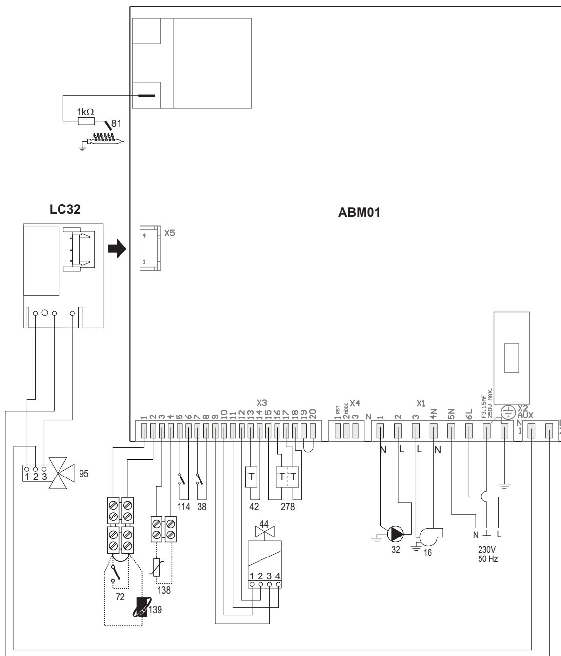
fig. 24 - Circuito elettrico
