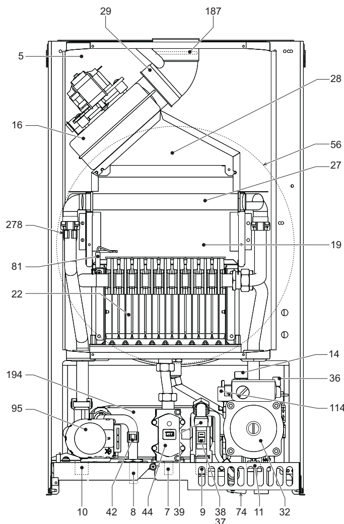
fig. 21 - Vista generale
