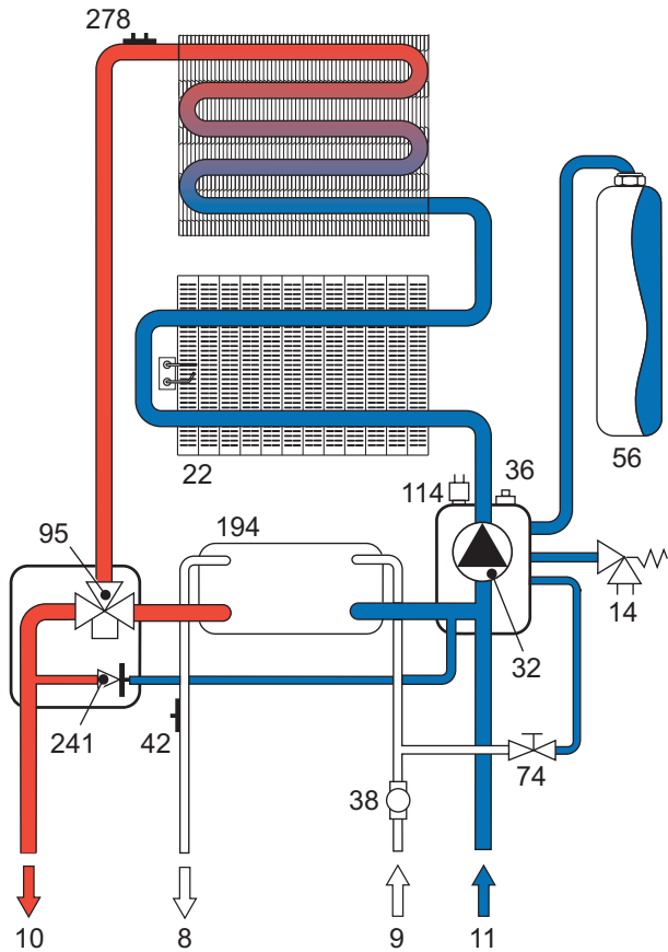
fig. 22 - Circuito calefacción
