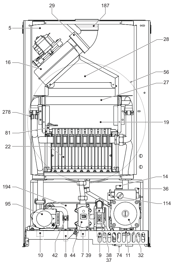
fig. 21 - Vista general
