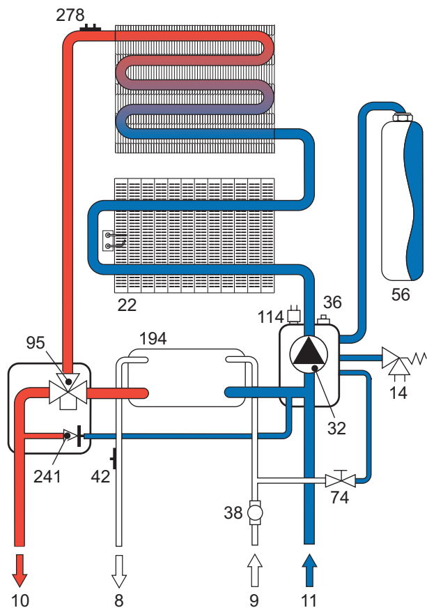
fig. 22 - Circuito riscaldamento
