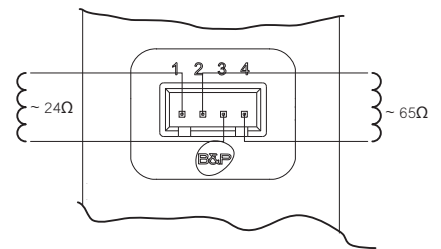
fig. 19 - Conexión de la válvula de gas
