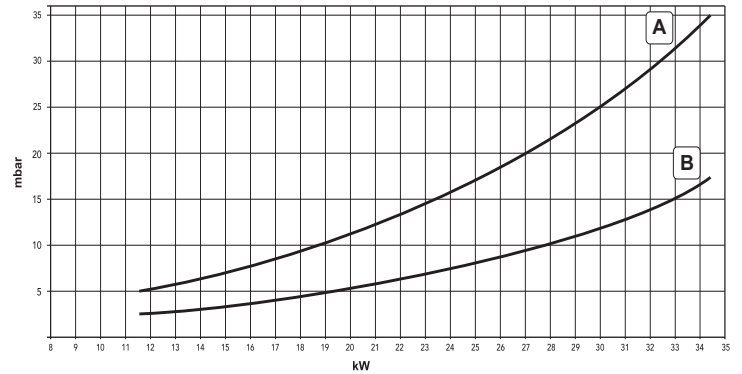
fig. 23 - Diagrama presión - potencia (CIPREA D 32 AS)
