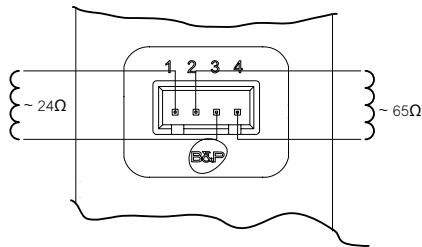
αέθ. 16 - Σύνδεση βαλβίδας αερίων
