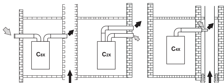
fig. 13 - Exemples de raccordement à des carreaux de fumées (→ = Air / ➔ = Fumées)
