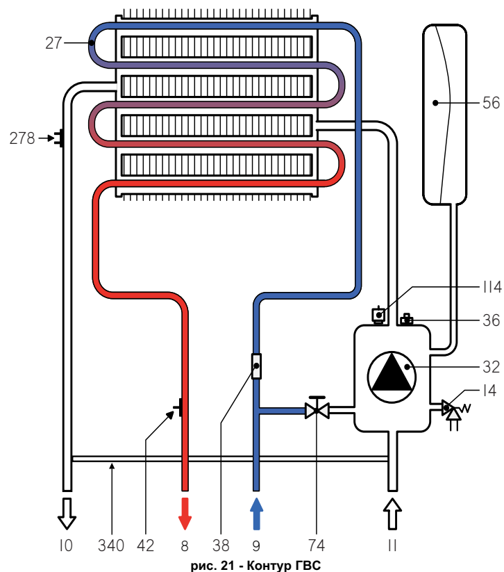
рис. 21 - Контур ГВС
