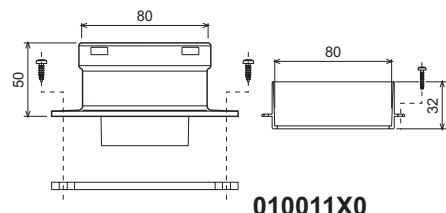
ΕΙΚ. 12 - Εξάρτημα σύνδεσης για ξεχωριστούς αγωγούς
