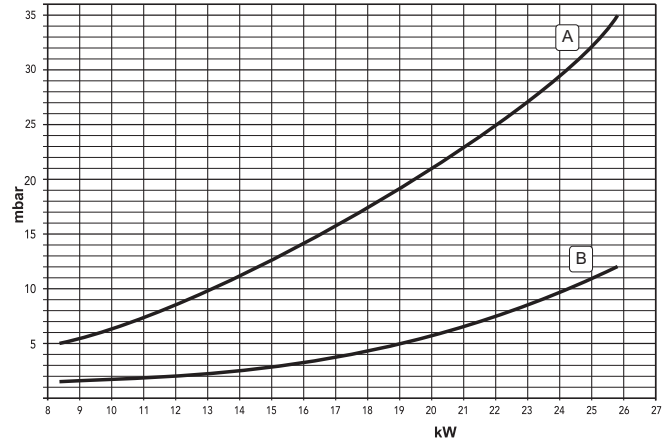
fig. 22 - Diagrama presión - potencia (CIPREA D 24 AS)
