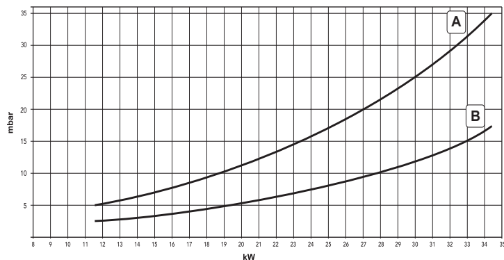
рис. 23 - Диаграммы давление - мощность (CIPREA D 32 AS)
