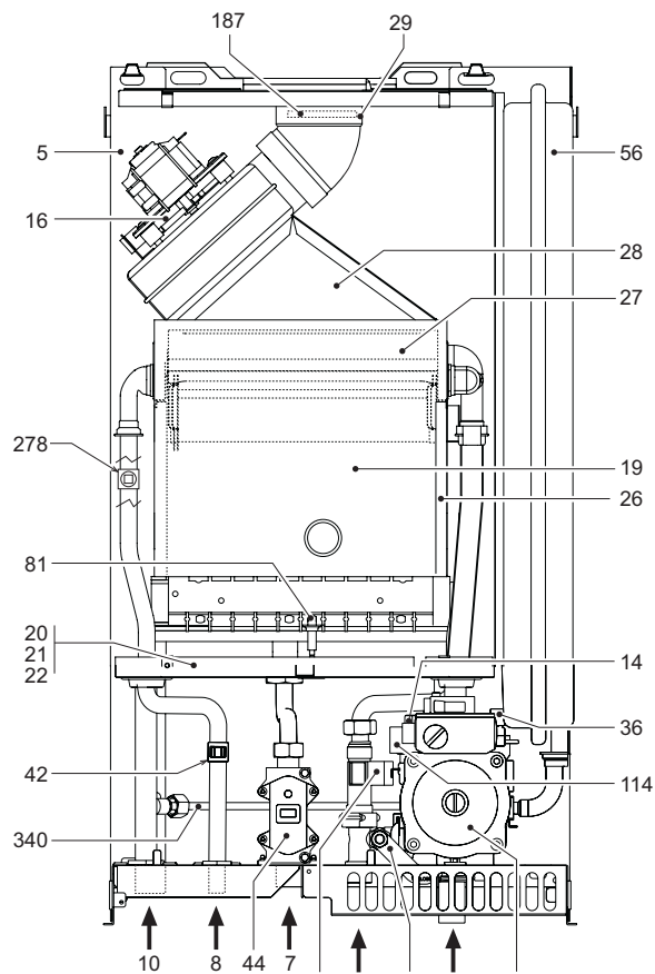
fig. 18 - Vedere generală CIPREA D 24 AS
