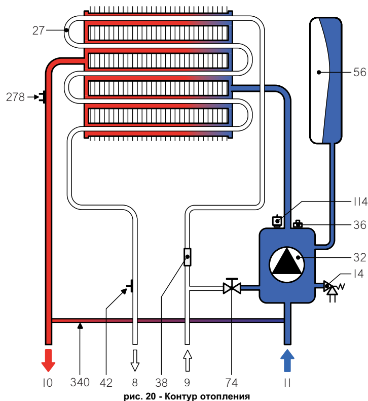
рис. 20 - Контур отопления
