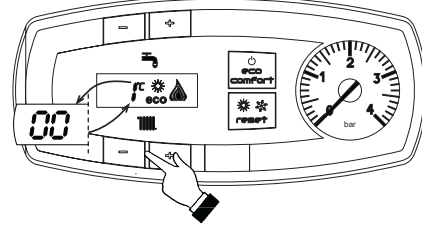
ΕΙΚ. 14 - Λειτουργία ΕΛΕΓΧΟΥ (ισχύς θέρμανσης = 100%)
