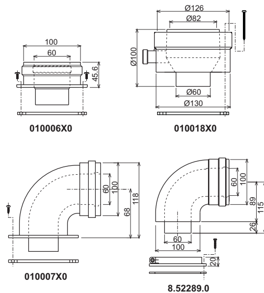
fig. 10 - Accesorios iniciales para conductos coaxiales
