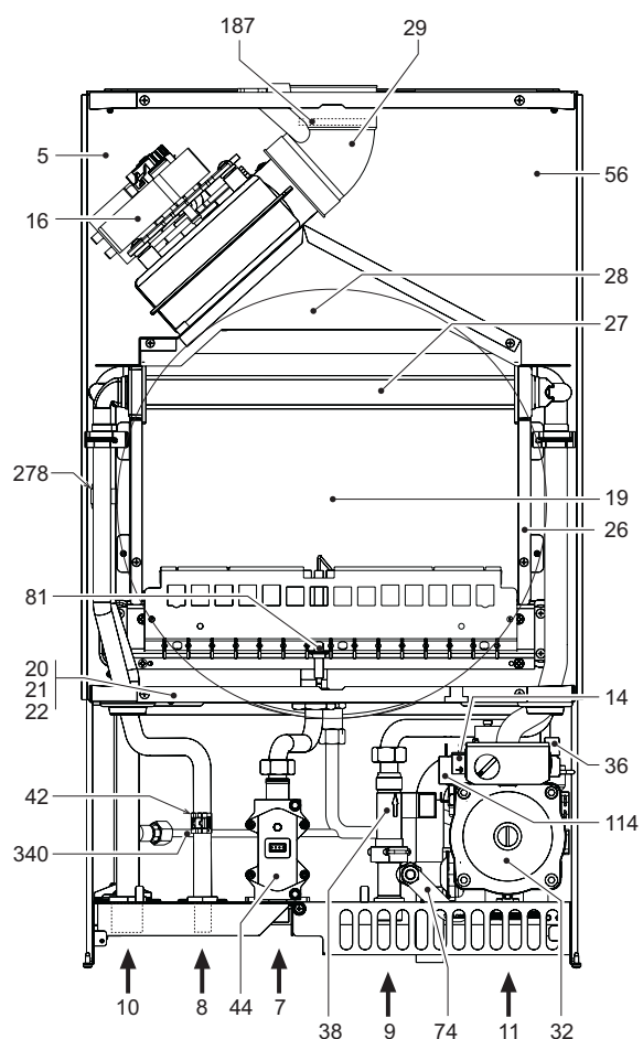
рис. 19 - Общий вид CIPREA D 32 AS
