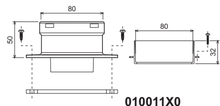
fig. 12 - Accessoire de départ pour conduits séparés
