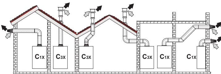
ΕΙΚ. 9 - Παραδείγματα σύνδεσης με ομοαξονικούς σωλήνες (← = Αέρας / → = Καυσαέρια)
