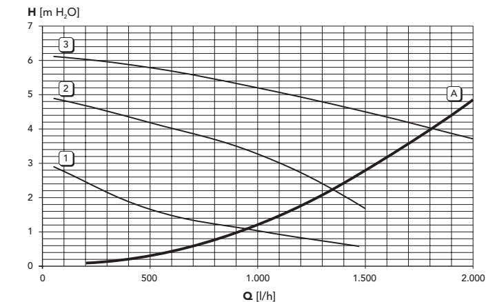
ΕΙΚ. 25 - Απώλειες φορτίου / μανομετρικό ύψος κυκλοφορητών (CIPREA D 32 AS)
