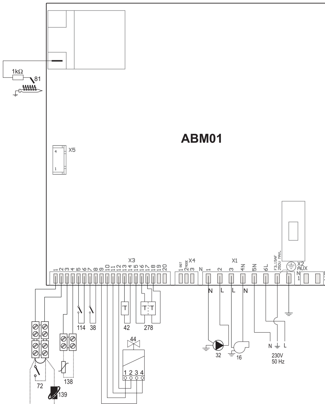
fig. 26 - Circuit électrique
