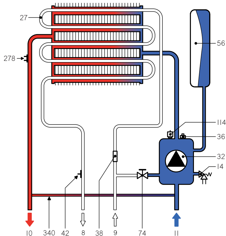
fig. 20 - Circuito Riscaldamento
