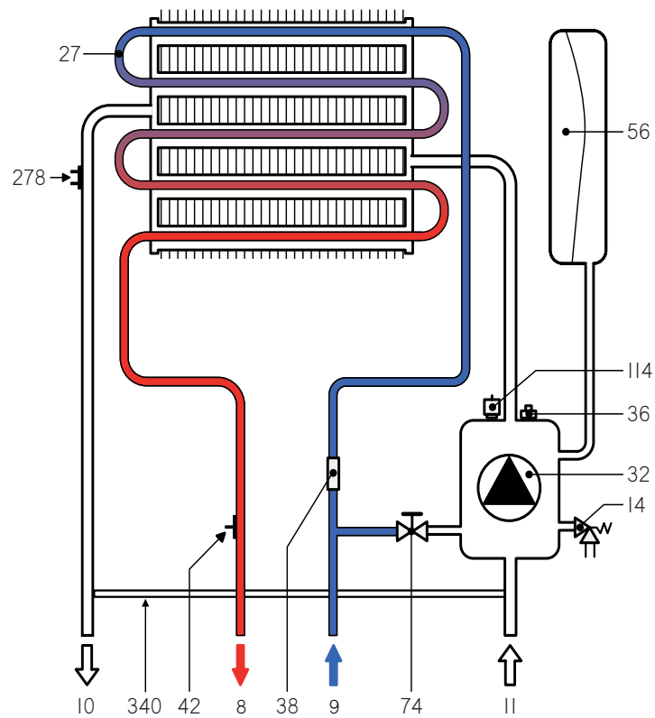
fig. 21 - Circuitul de apă caldă menajeră
