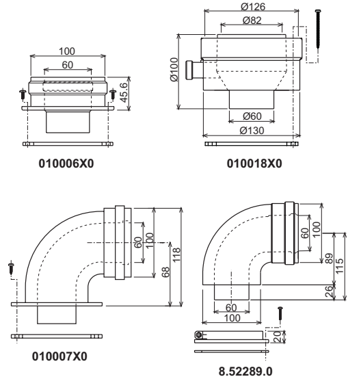
ΕΙΚ. 10 - Εξαρτήματα σύνδεσης για ομοαξονικούς αγωγούς
