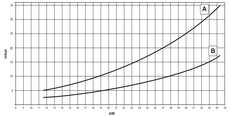
fig. 23 - Diagramme pression - puissance (CIPREA D 32 AS)
