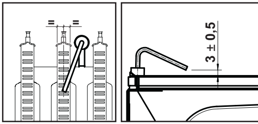
ΕΙΚ. 17 - Τοποθέτηση ηλεκτροδίου
