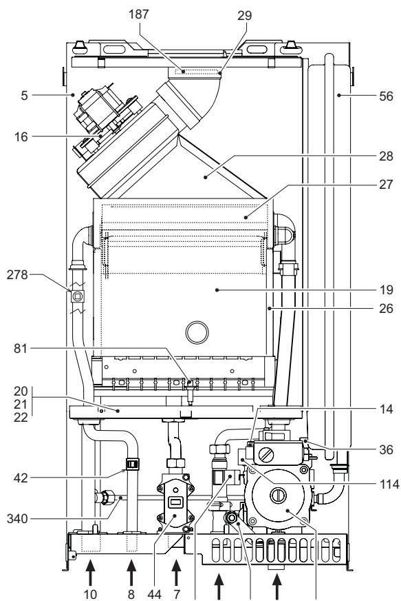
рис. 18 - Общий вид CIPREA D 24 AS
