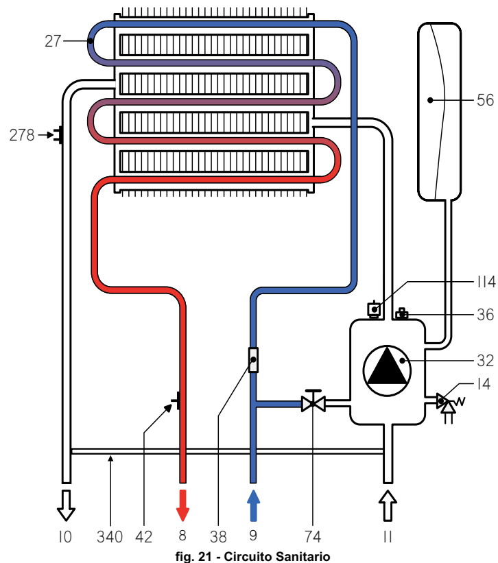
fig. 21 - Circuito Sanitario
