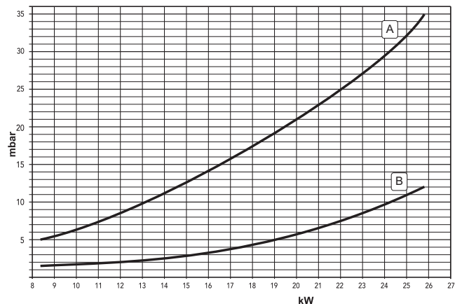
fig. 22 - Diagramă presiune - putere (CIPREA D 24 AS)
