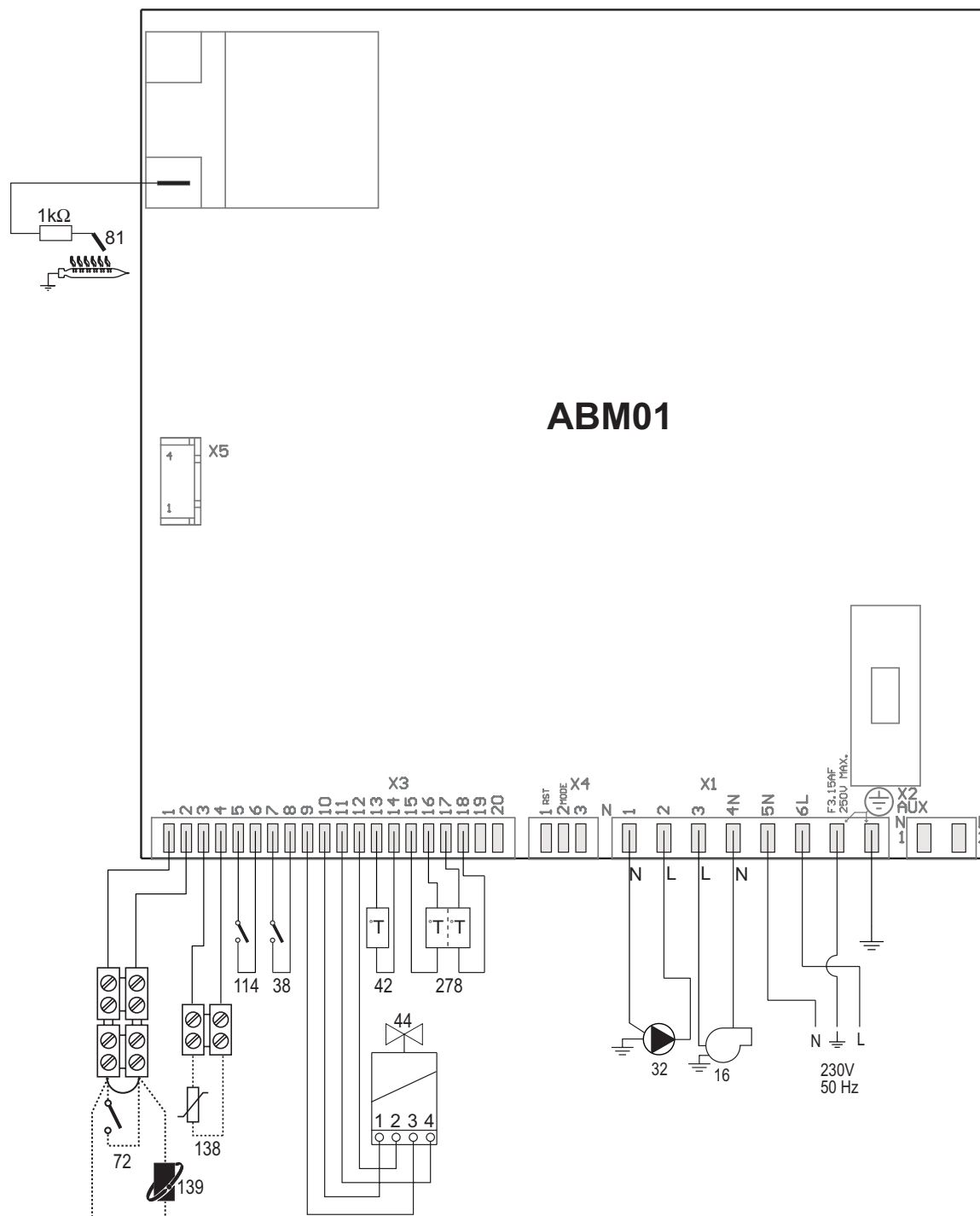
fig. 26 - Circuito eléctrico
