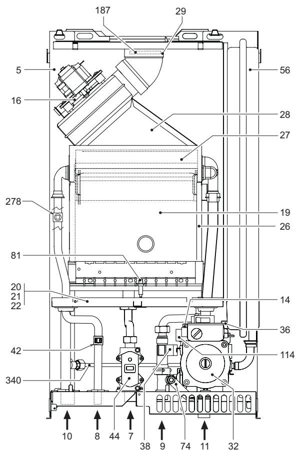
fig. 18 - Vista generale CIPREA D 24 AS
