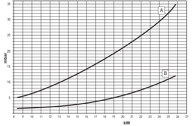
ΕΙΚ. 22 - Διάγραμμα πίεσης - ισχύος (CIPREA D 24 AS)
