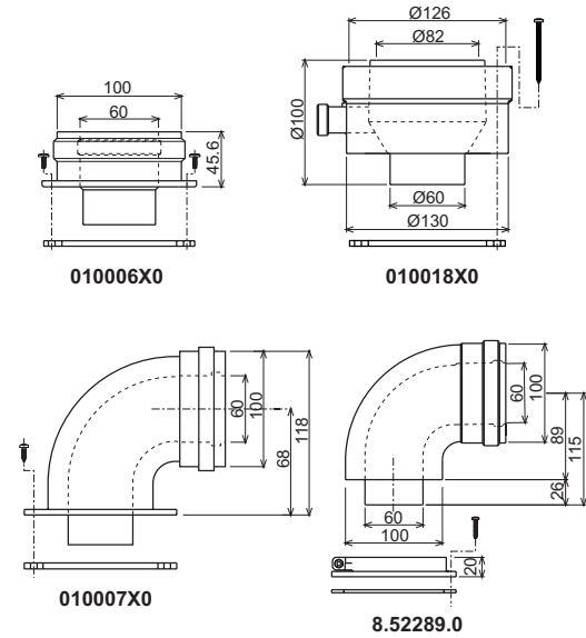
fig. 10 - Accessoires de départ pour conduits coaxiaux
