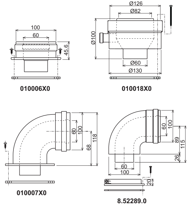
рис. 10 - Исходные элементы для коаксиальных воздуховодов
