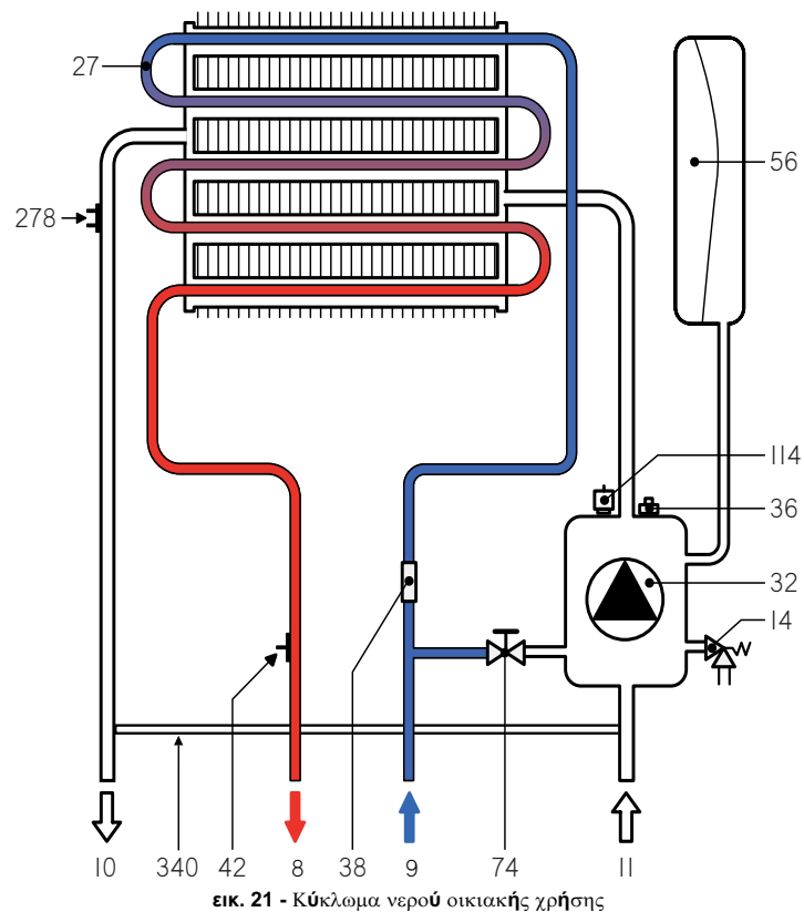
εικ. 21 - Κύκλωμα νερού οικιακής χρήσης
