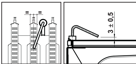
fig. 17 - Poziționarea electrozului
