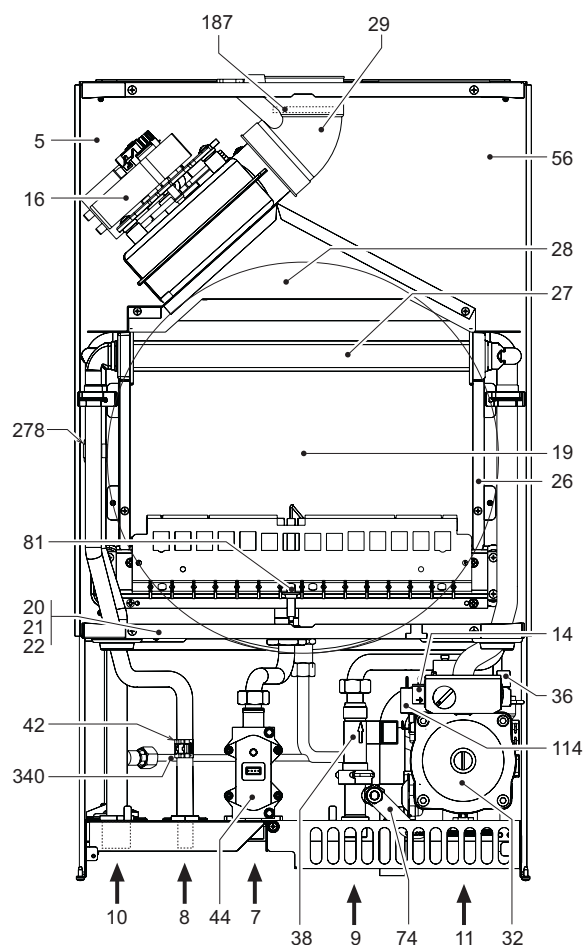
εικ. 19 - Γενική όψη CIPREA D 32 AS
