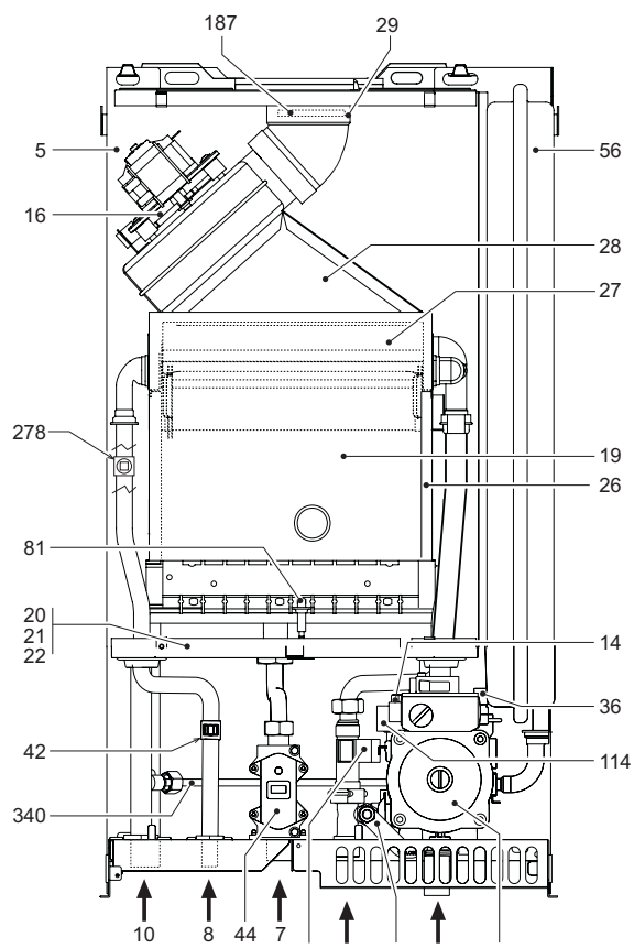
fig. 18 - Vue générale CIPREA D 24 AS
