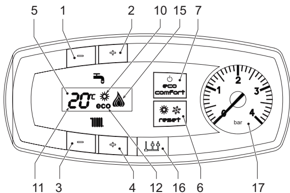
fig. 1 - Panneau de contrôle
