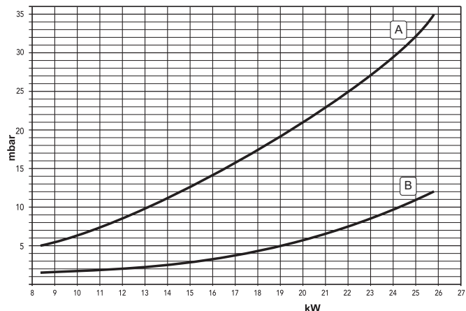
рис. 22 - Диаграммы давление - мощность (CIPREA D 24 AS)
