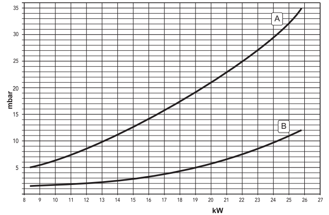
fig. 22 - Diagramma pressione - potenza (CIPREA D 24 AS)
