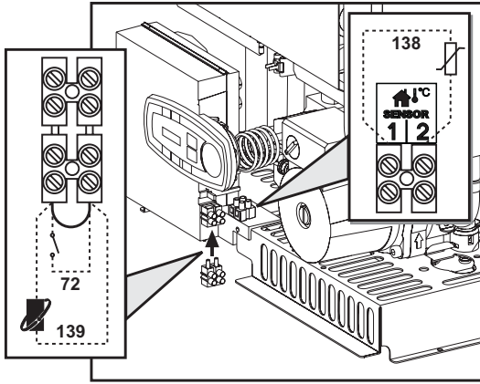
рис. 8 - Доступ к клеммной коробке
