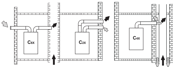
ΕΙΚ. 13 - Παραδείγματα σύνδεσης σε καπνοδόχους (⇨ = Αέρας / ⇩ = Καυσαέρια)
