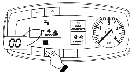
fig. 14 - Modo TEST (potencia de calefacción = 100%)
