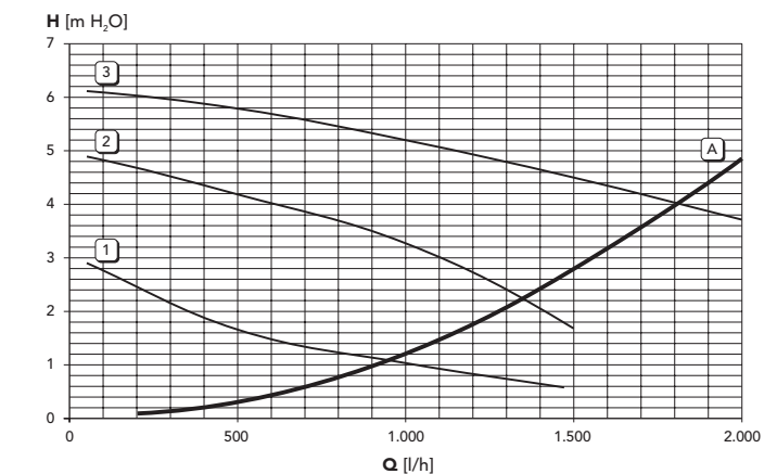
fig. 25 - Pertes de charge / pression circulateurs (CIPREA D 32 AS)
