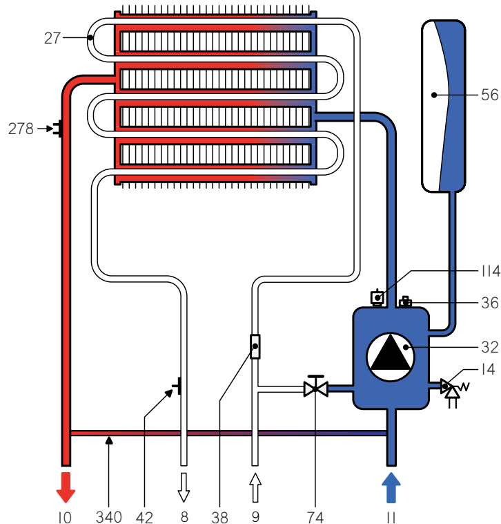
fig. 20 - Circuitul de încălzire
