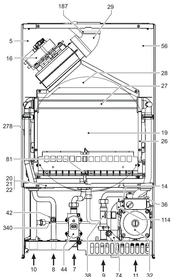
fig. 19 - Vedere generală CIPREA D 32 AS
