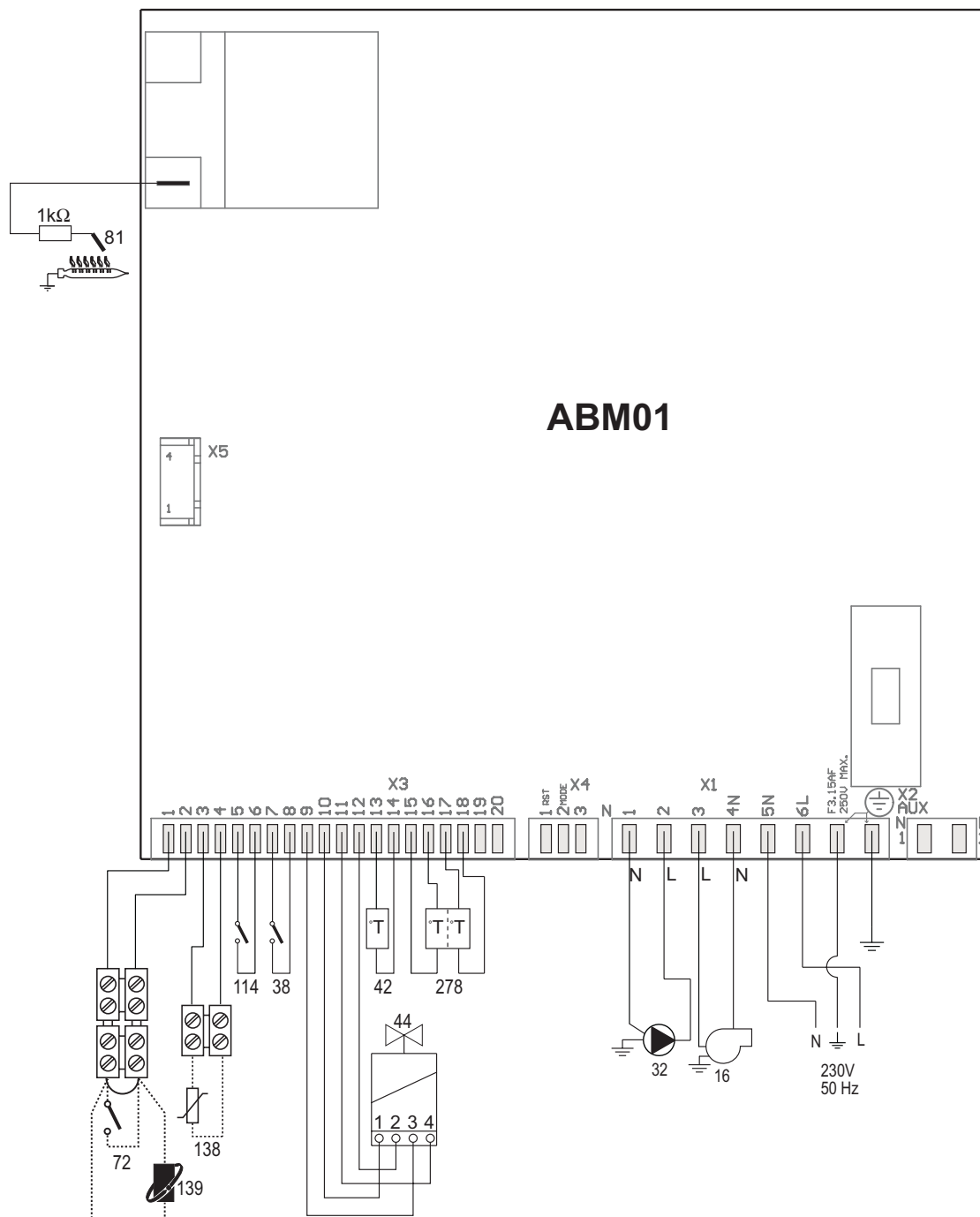
ΕΙΚ. 26 - Ηλεκτρικό κύκλωμα
