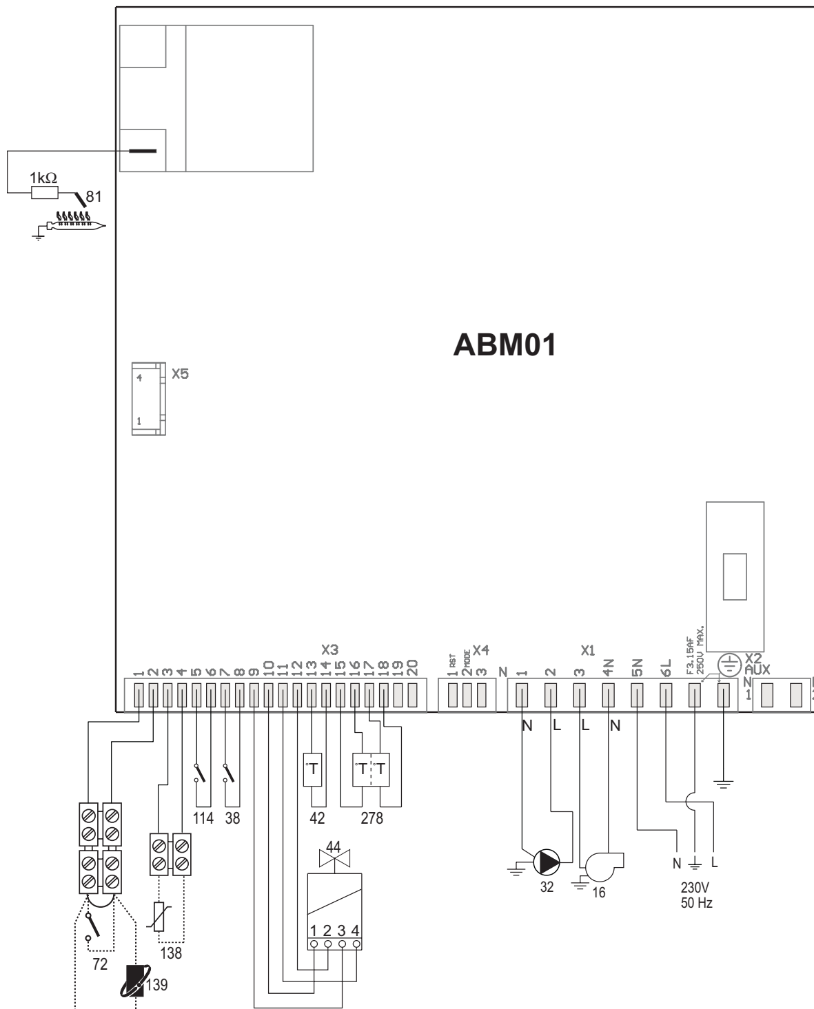
fig. 26 - Circuito elettrico
