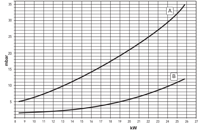
fig. 22 - Diagramme pression - puissance (CIPREA D 24 AS)
