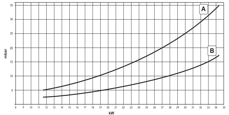
fig. 23 - Diagramma pressione - potenza (CIPREA D 32 AS)
