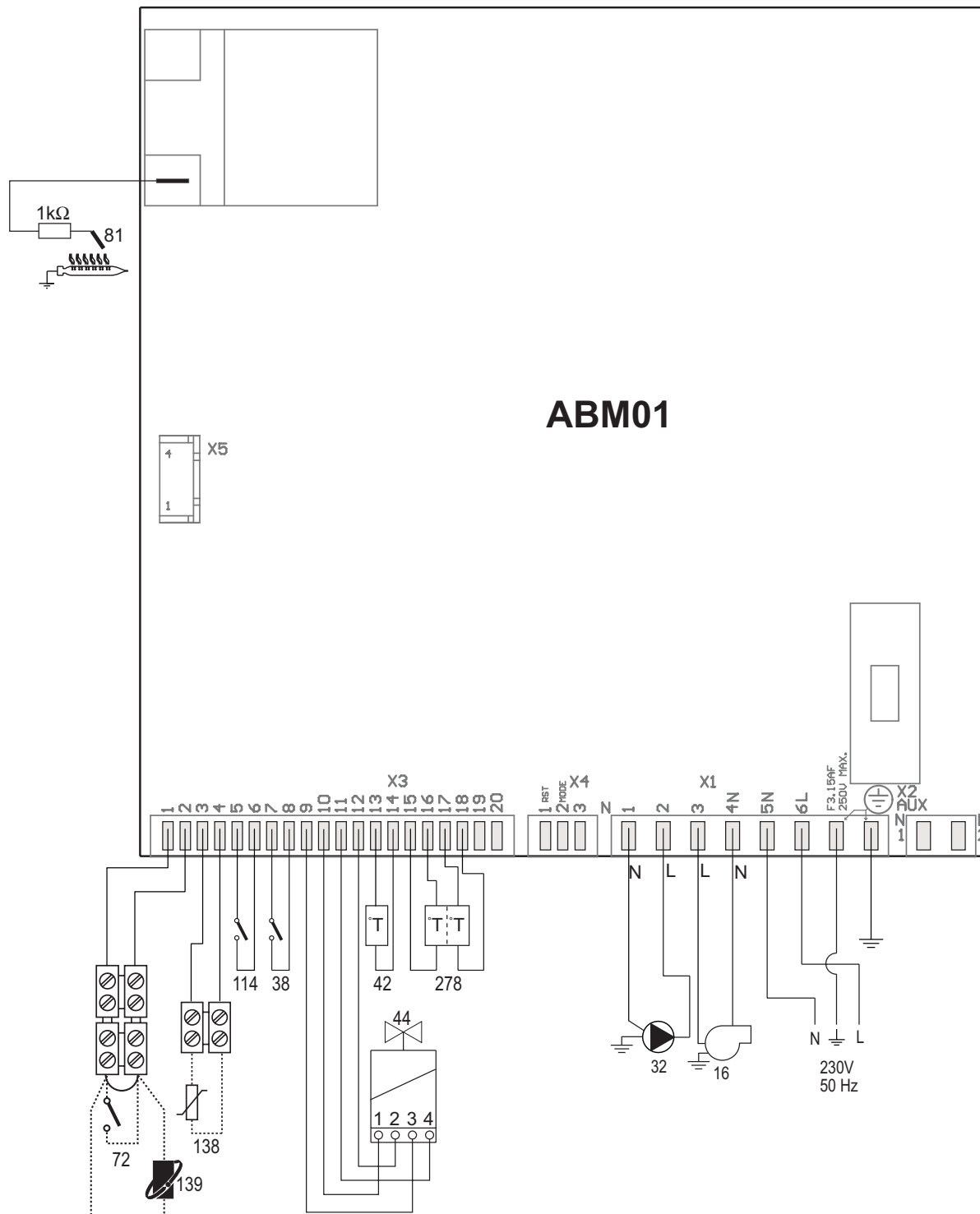
рис. 26 - Электрическая система
