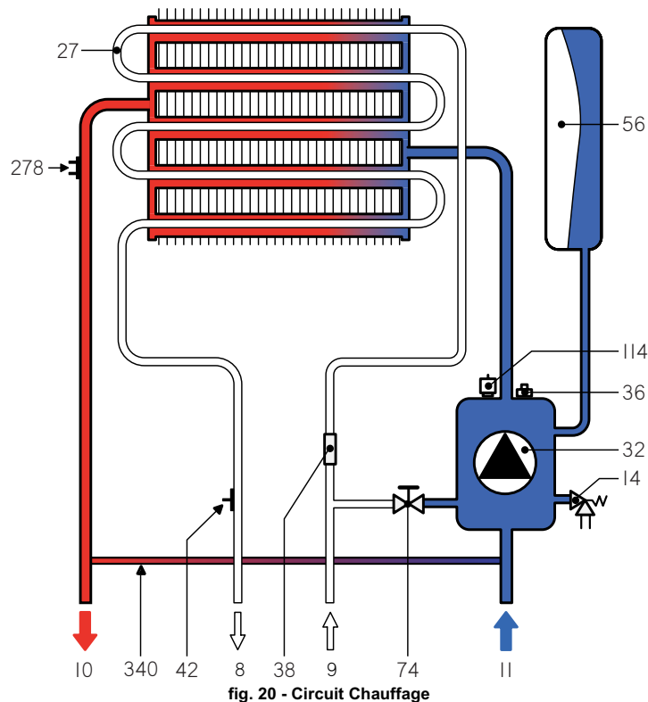
fig. 20 - Circuit Chauffage
