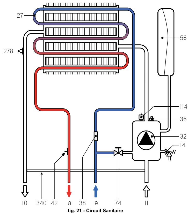
fig. 21 - Circuit Sanitaire
