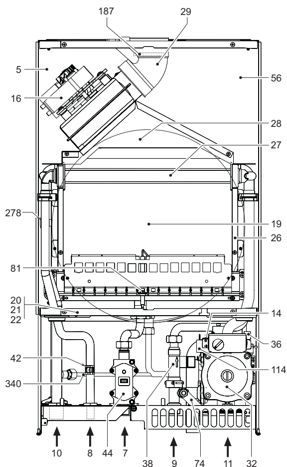
fig. 19 - Vue générale CIPREA D 32 AS
