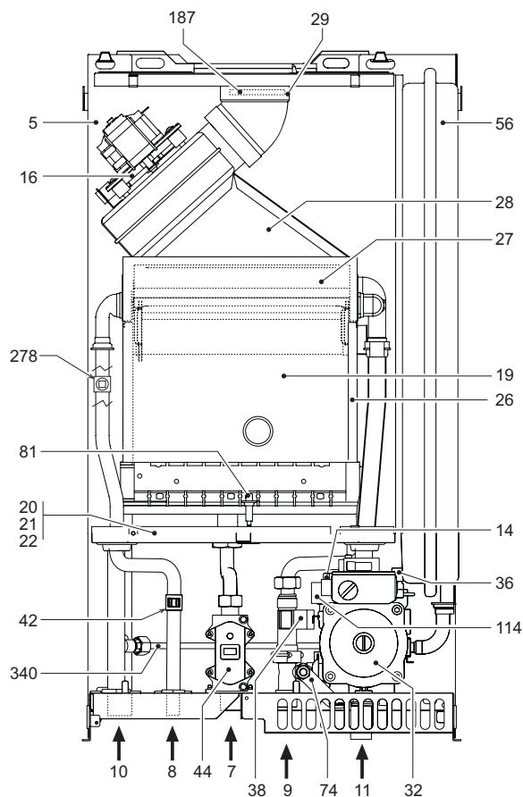
εικ. 18 - Γενική όψη CIPREA D 24 AS
