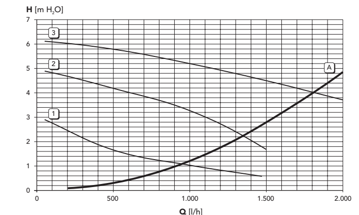
fig. 25 - Pérdidas de carga / altura manométrica bombas de circulación (CIPREA D 32 AS)
