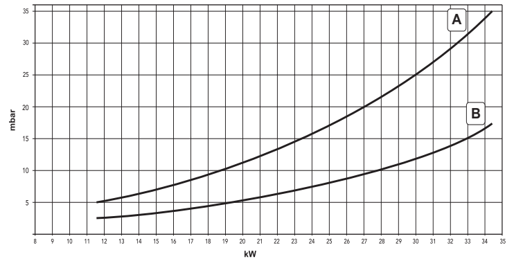
ΕΙΚ. 23 - Διάγραμμα πίεσης - ισχύος (CIPREA D 32 AS)
