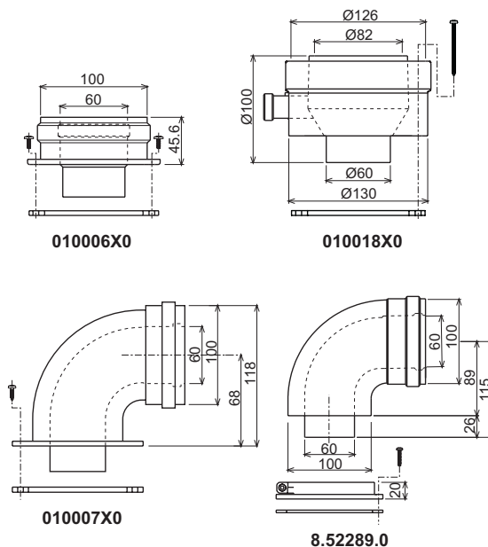
fig. 10 - Accessori di partenza per condotti coassiali
