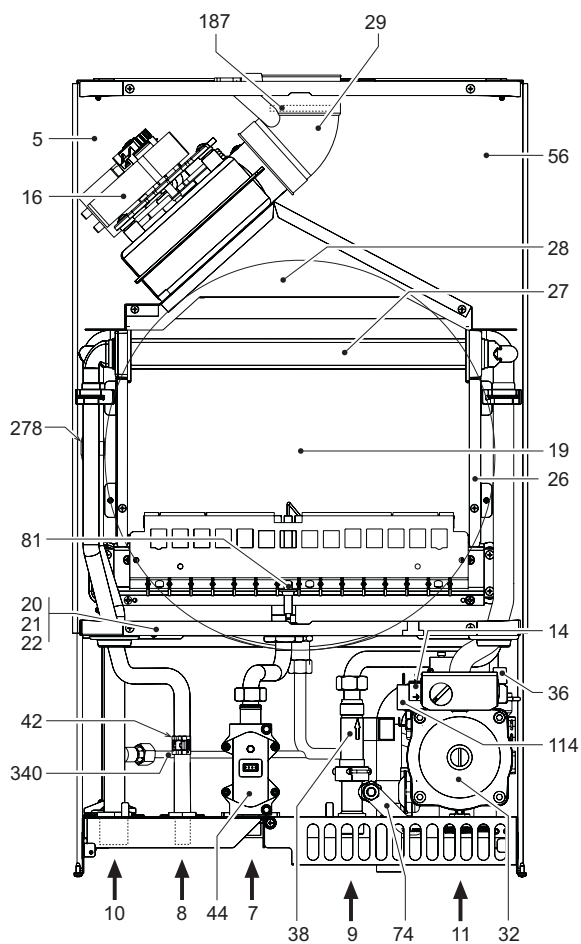
fig. 19 - Vista generale CIPREA D 32 AS
