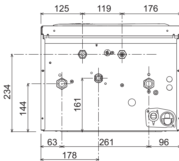
рис. 29 - Вид снизу
