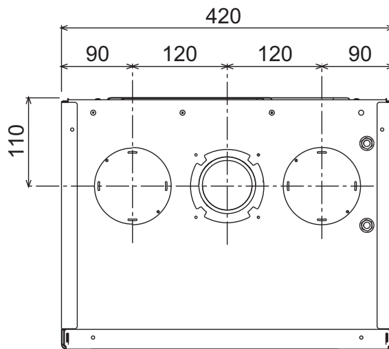
рис. 28 - Вид сверху
