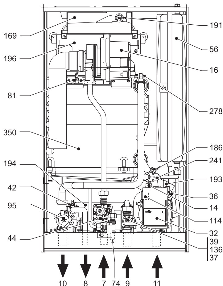
рис. 30 - Общий вид
