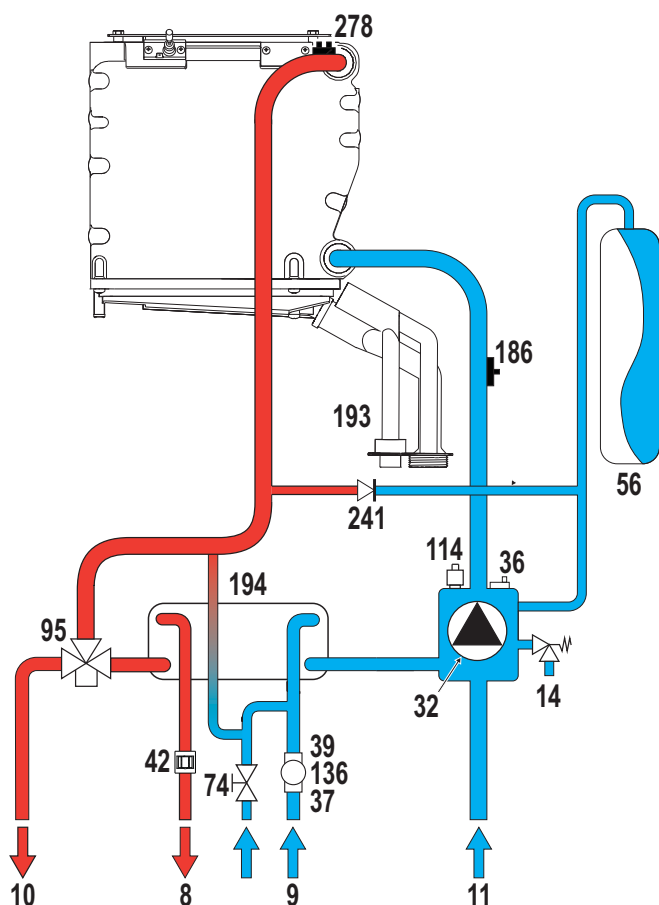
рис. 31 - Гидравлический контур
