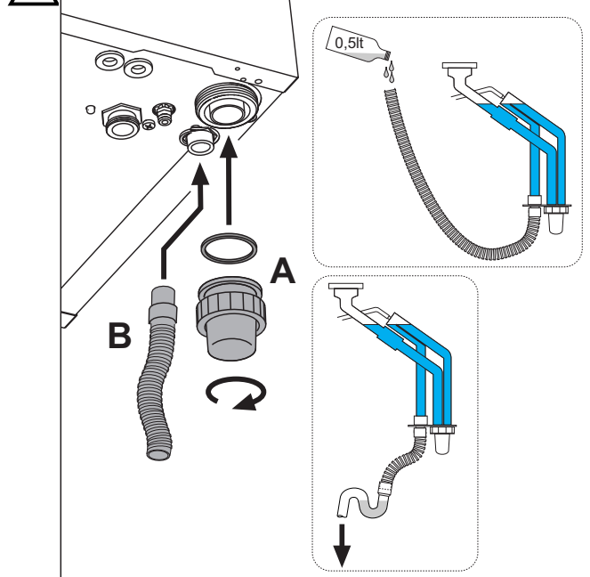
fig. 20 - Raccordement de l'évacuation de la condensation
