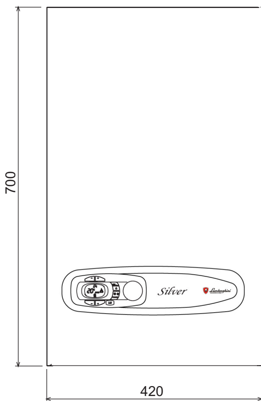
fig. 26 - Vue avant
