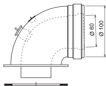
рис. 16 - Элементы для коаксиальных воздухопроводов
