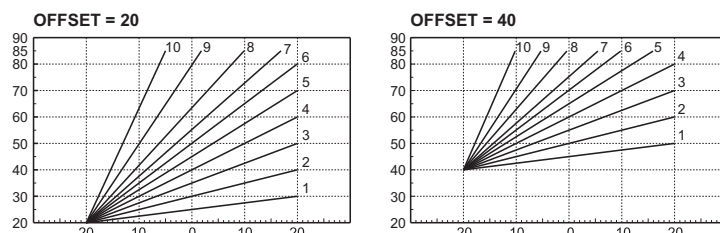
рис. 12 - Пример параллельного смещения компенсационных характеристик
